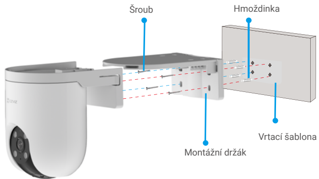
Obr. 2 Montáž na zeď
