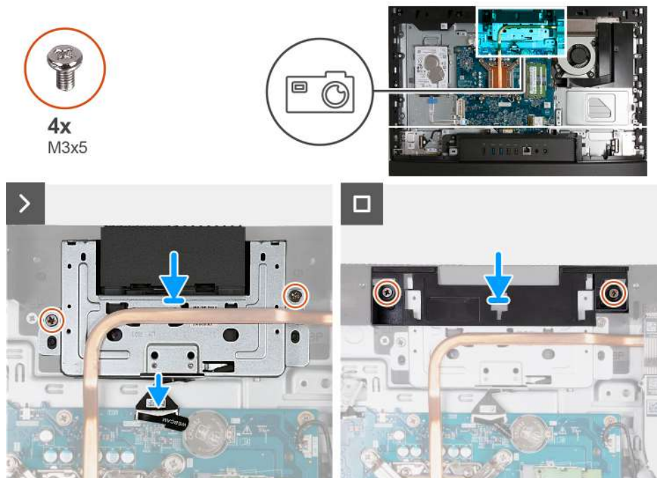
Obrázek 102. Montáž sestavy zasouvací kamery
