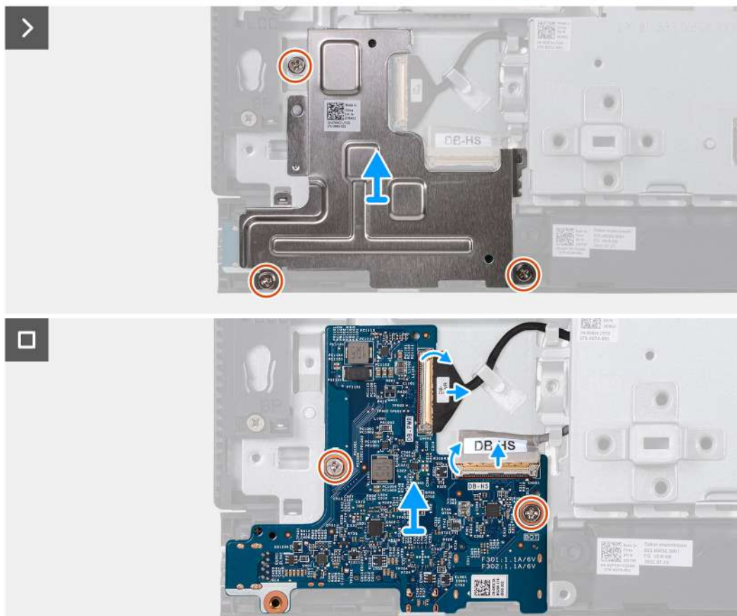
Obrázek 72. Demontáž desky vypínače a I/O
