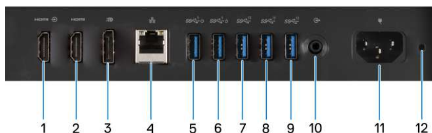
Obrázek 8. Pohled na zadní panel počítače OptiPlex All-in-One 7420 s výkonným procesorem
