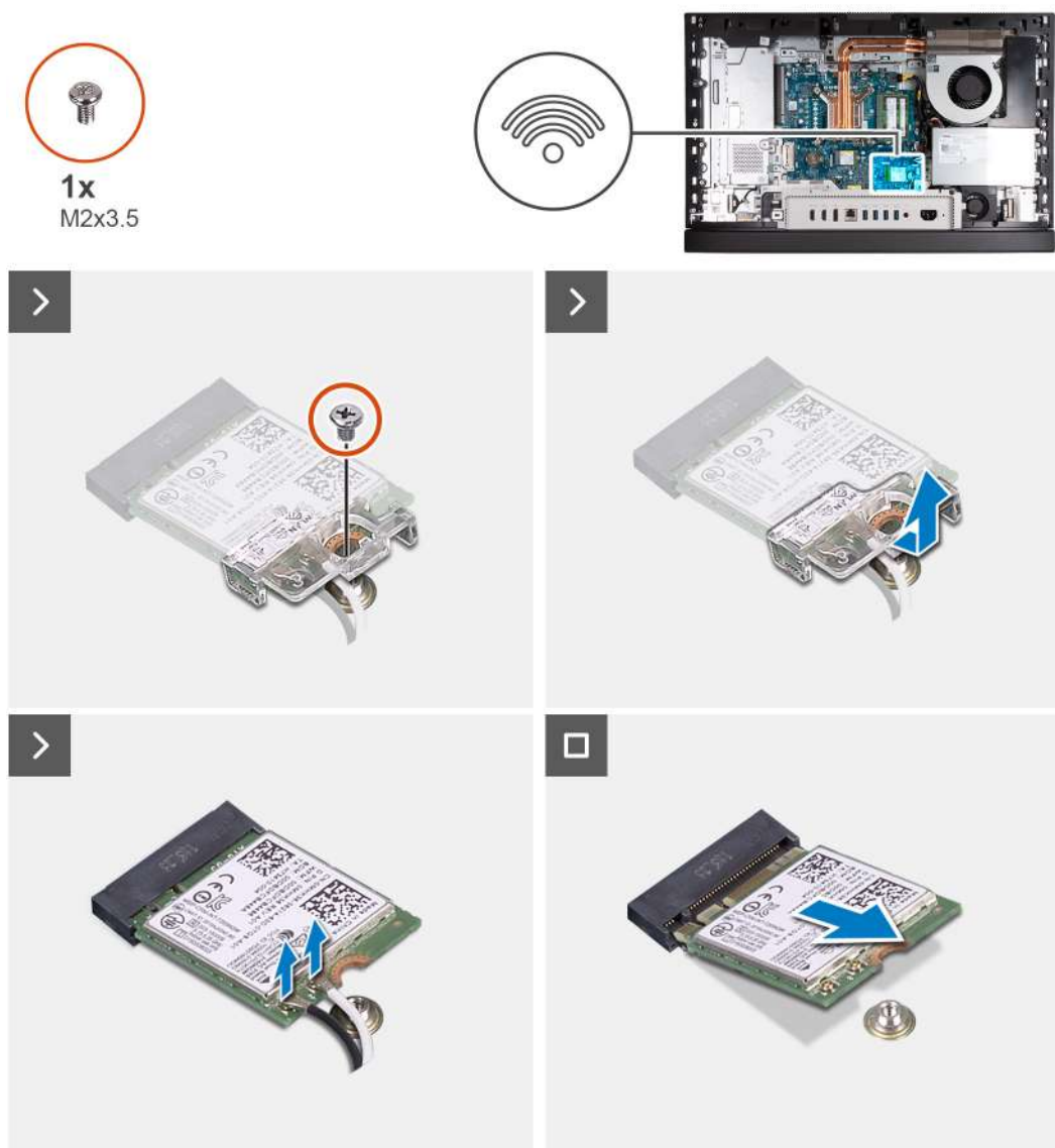
Obrázek 28. Demontáž bezdrátové karty
