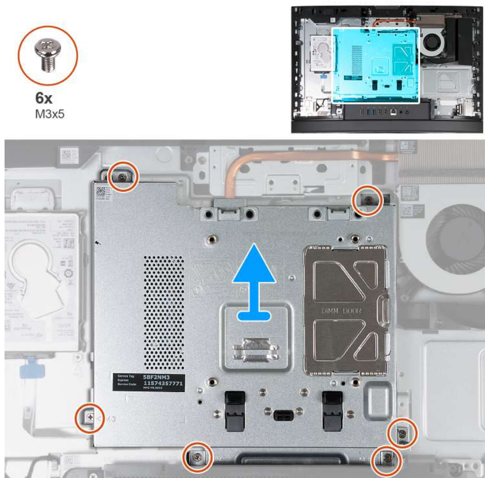
Obrázek 26. Demontáž krytu základní desky
