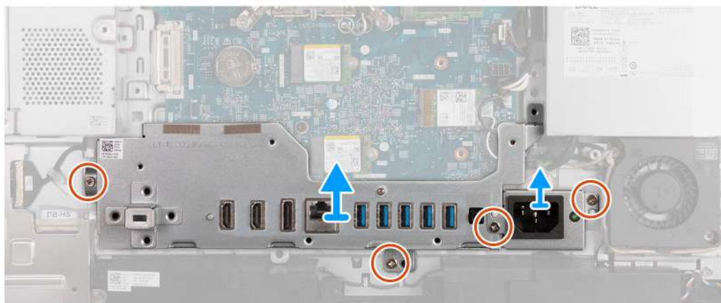
Obrázek 58. Demontáž držáku panelu I/O
