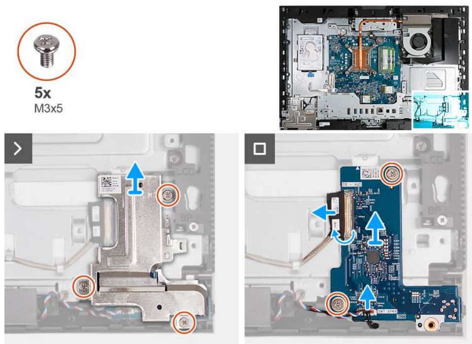
Obrázek 121. Demontáž zvukové karty
