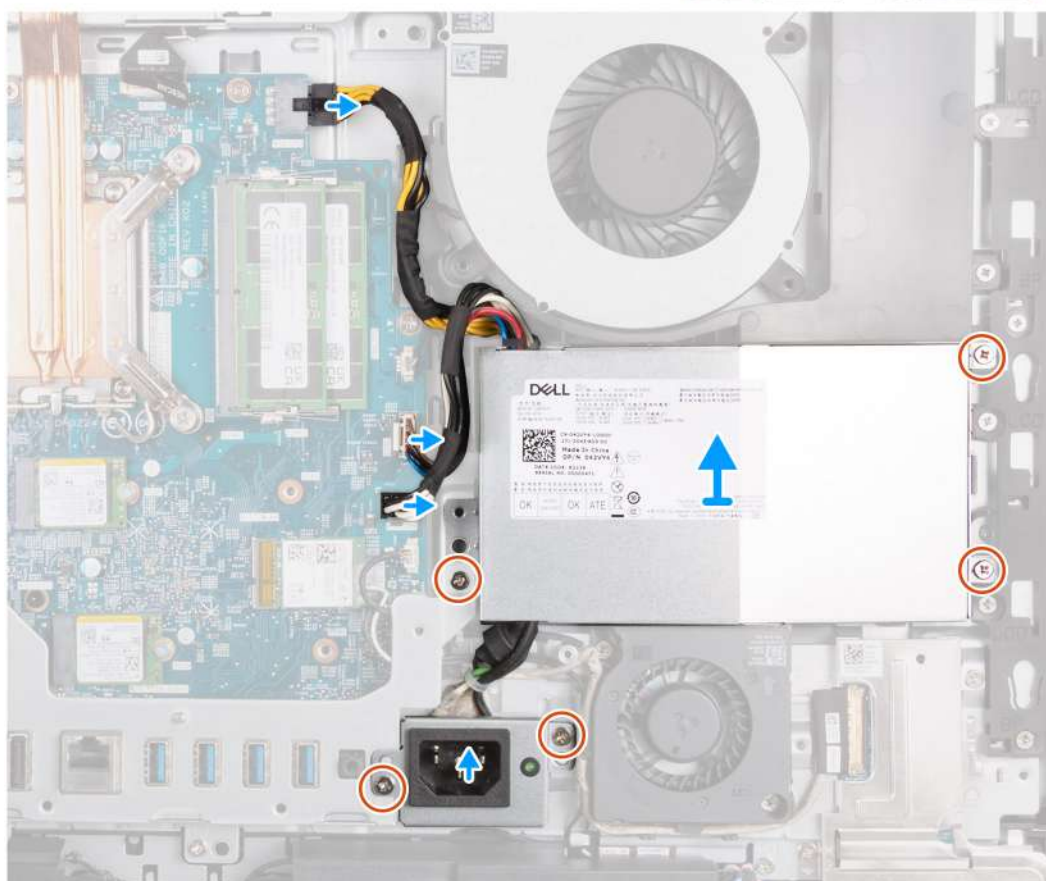
Obrázek 50. Demontáž napájecí jednotky
