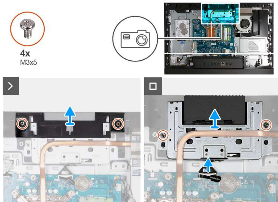
Obrázek 101. Demontáž sestavy zasouvací kamery
