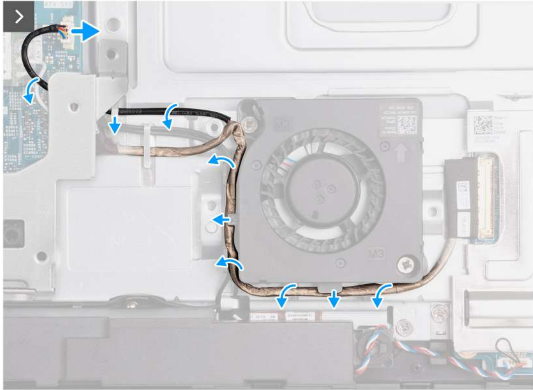
Obrázek 52. Demontáž jednotky ventilátoru napájecího zdroje
