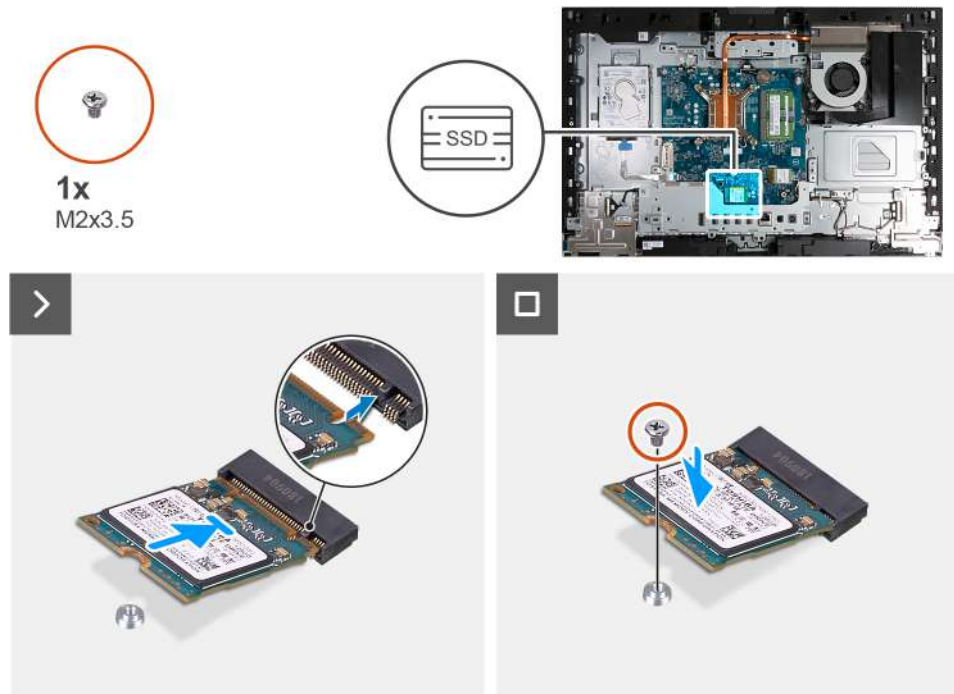
Obrázek 91. Montáž disku SSD M.2 2230
