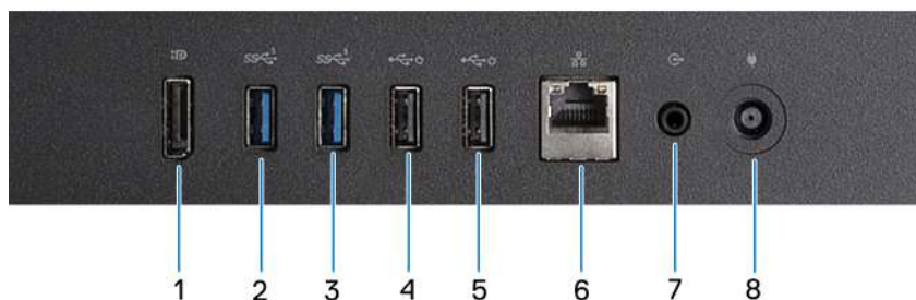
Obrázek 7. Pohled na zadní panel počítače OptiPlex All-in-One 7420 s úsporným procesorem
