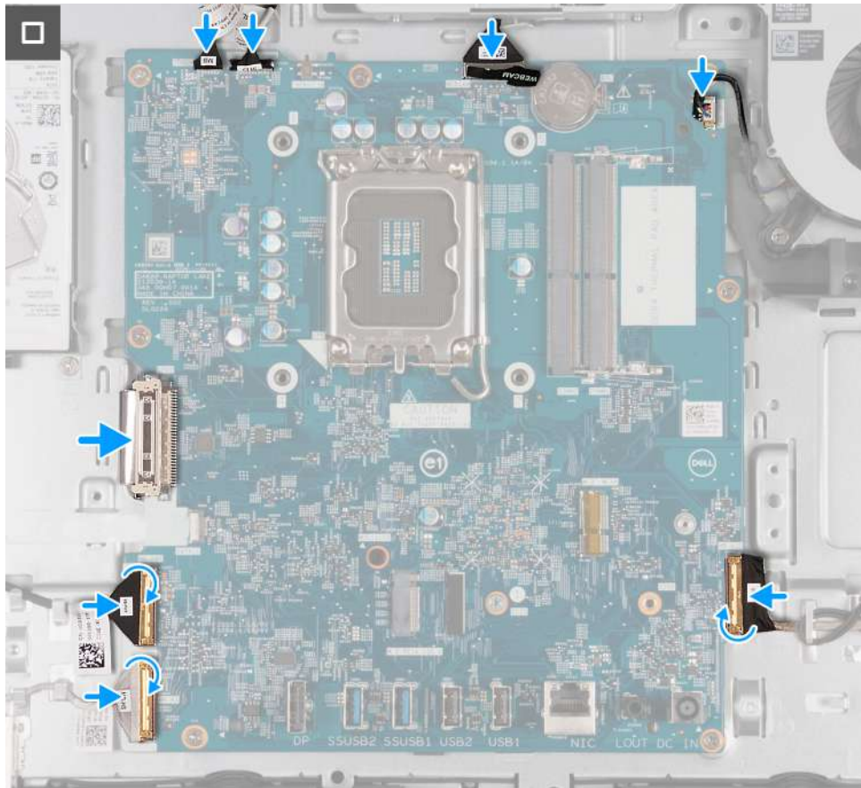
Obrázek 118. Montáž základní desky
