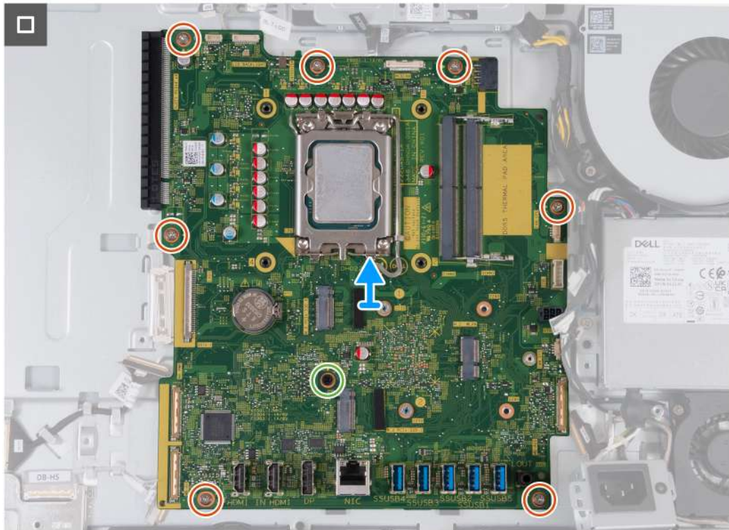
Obrázek 68. Demontáž základní desky
