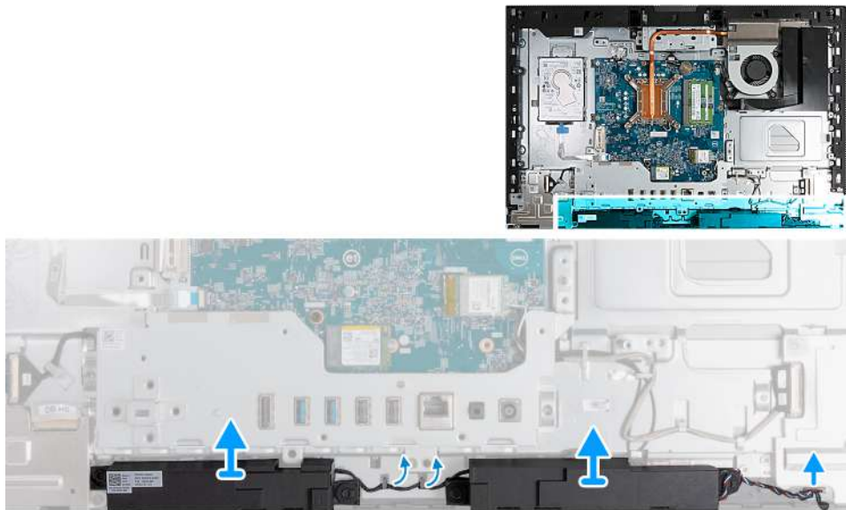
Obrázek 107. Demontáž reproduktorů
