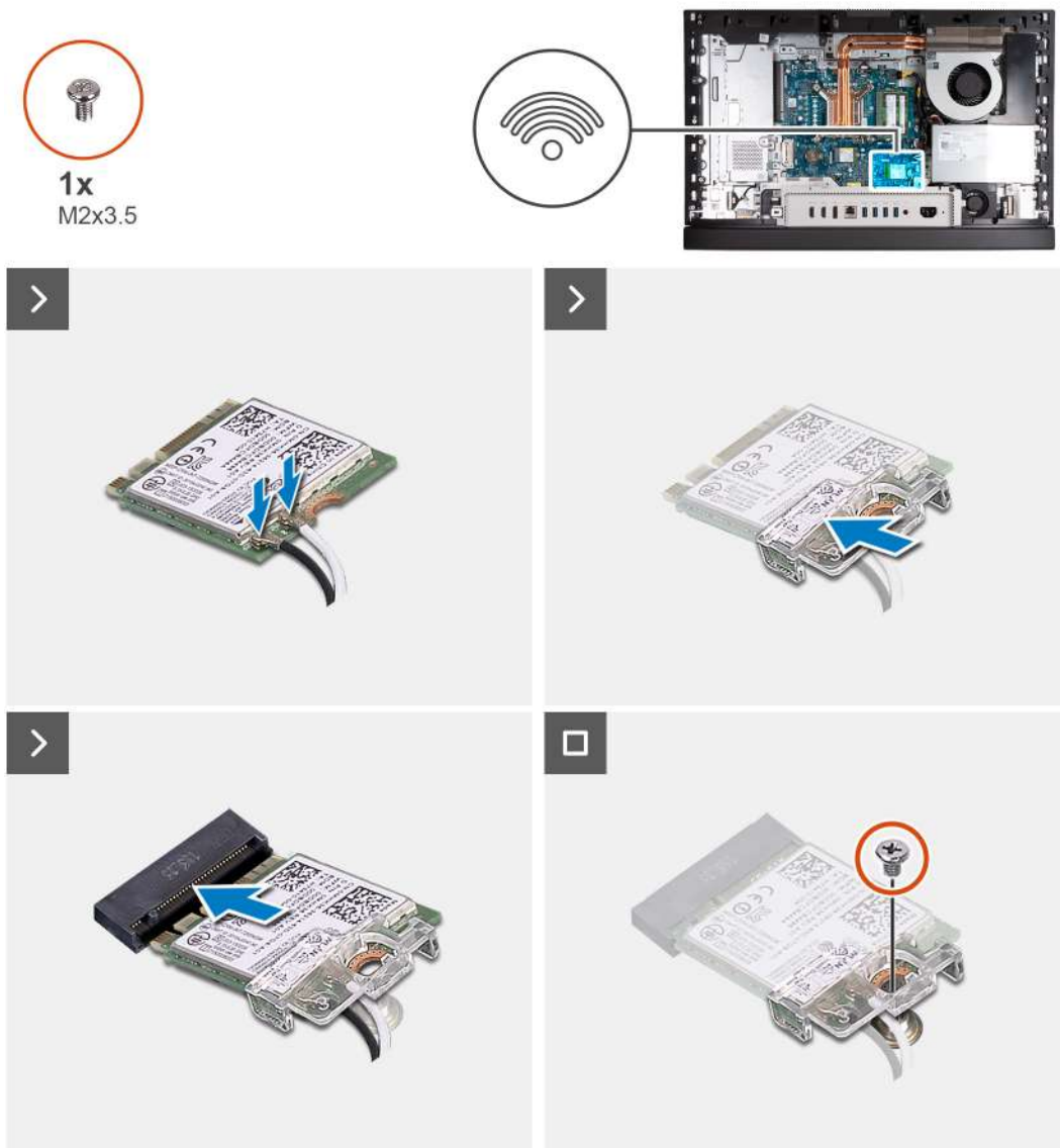
Obrázek 29. Montáž bezdrátové karty
