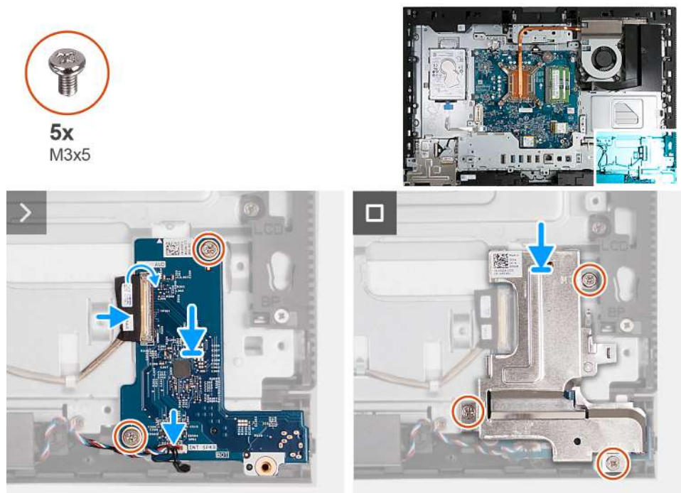
Obrázek 122. Montáž zvukové karty
