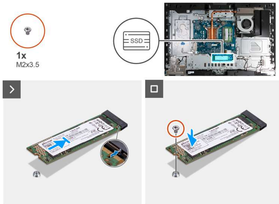
Obrázek 93. Montáž disku SSD M.2 2280
