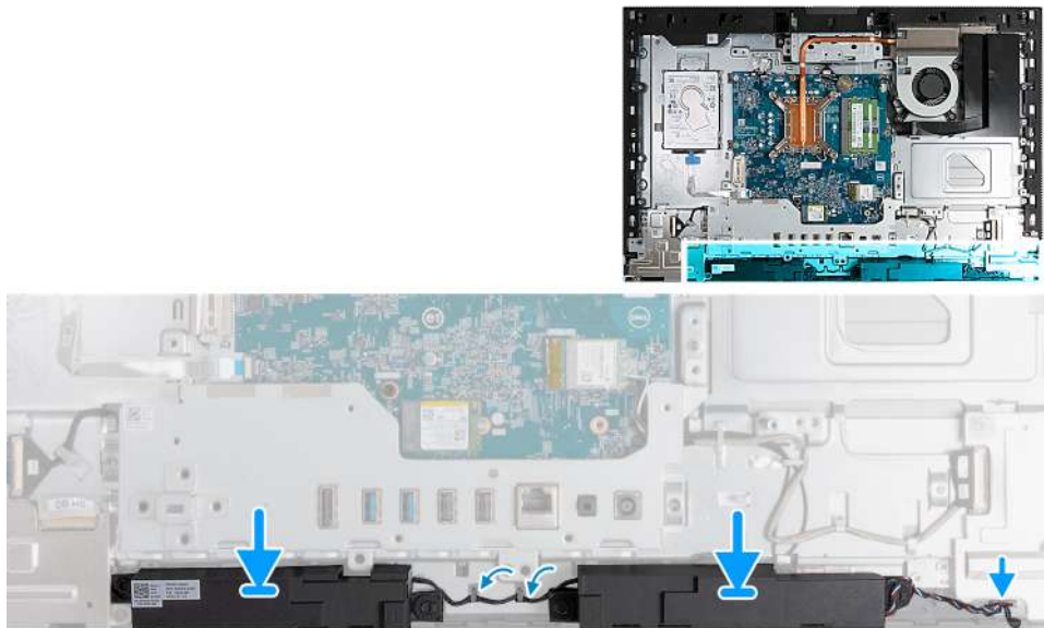
Obrázek 108. Montáž reproduktorů
