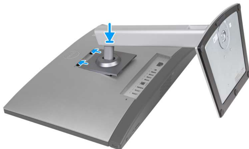
Obrázek 81. Montáž stojanu
