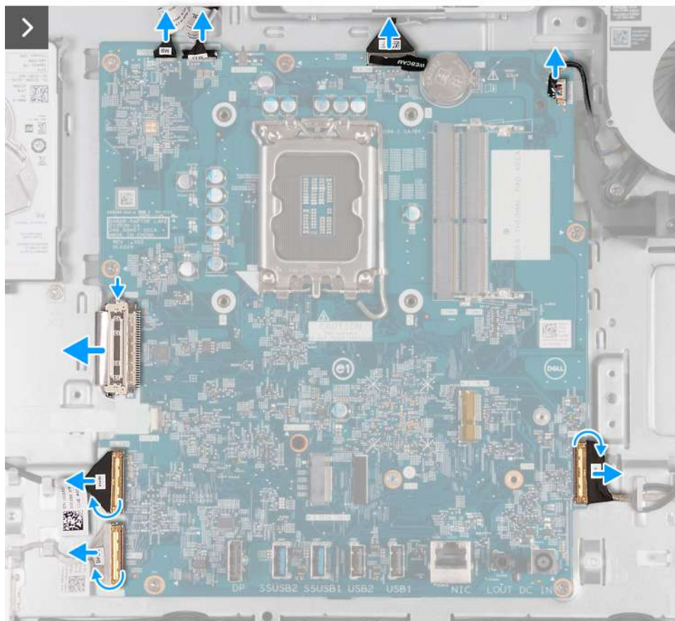
Obrázek 114. Demontáž základní desky
