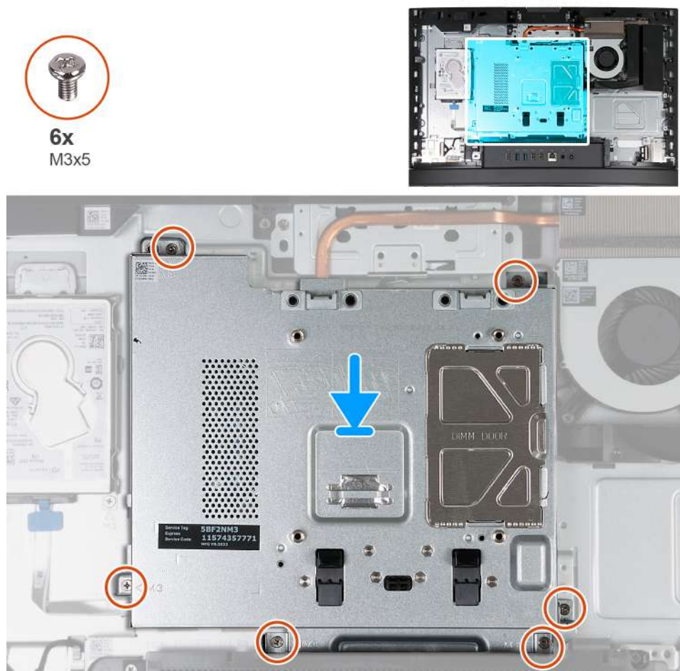
Obrázek 27. Montáž krytu základní desky
