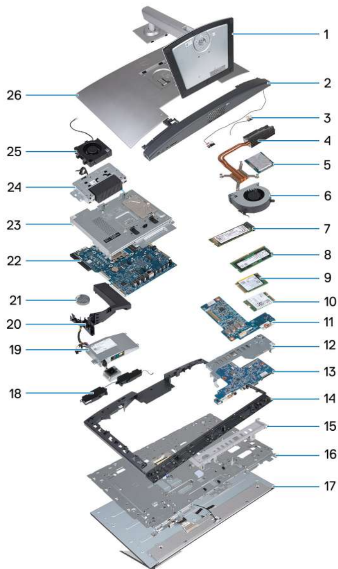
Obrázek 16. Hlavní komponenty počítače OptiPlex All-in-One 7420 s výkonným procesorem
