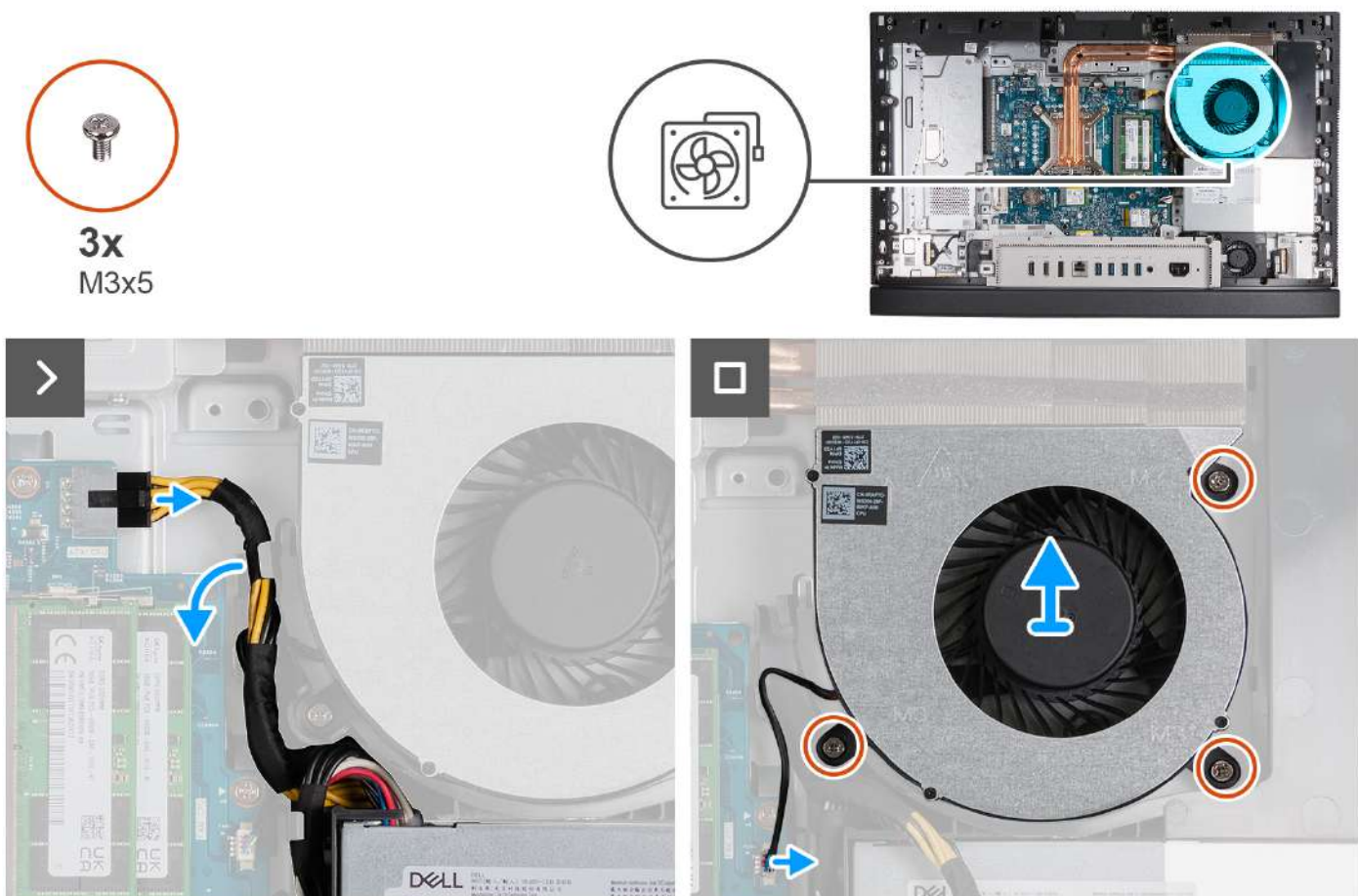
Obrázek 48. Demontáž ventilátoru
