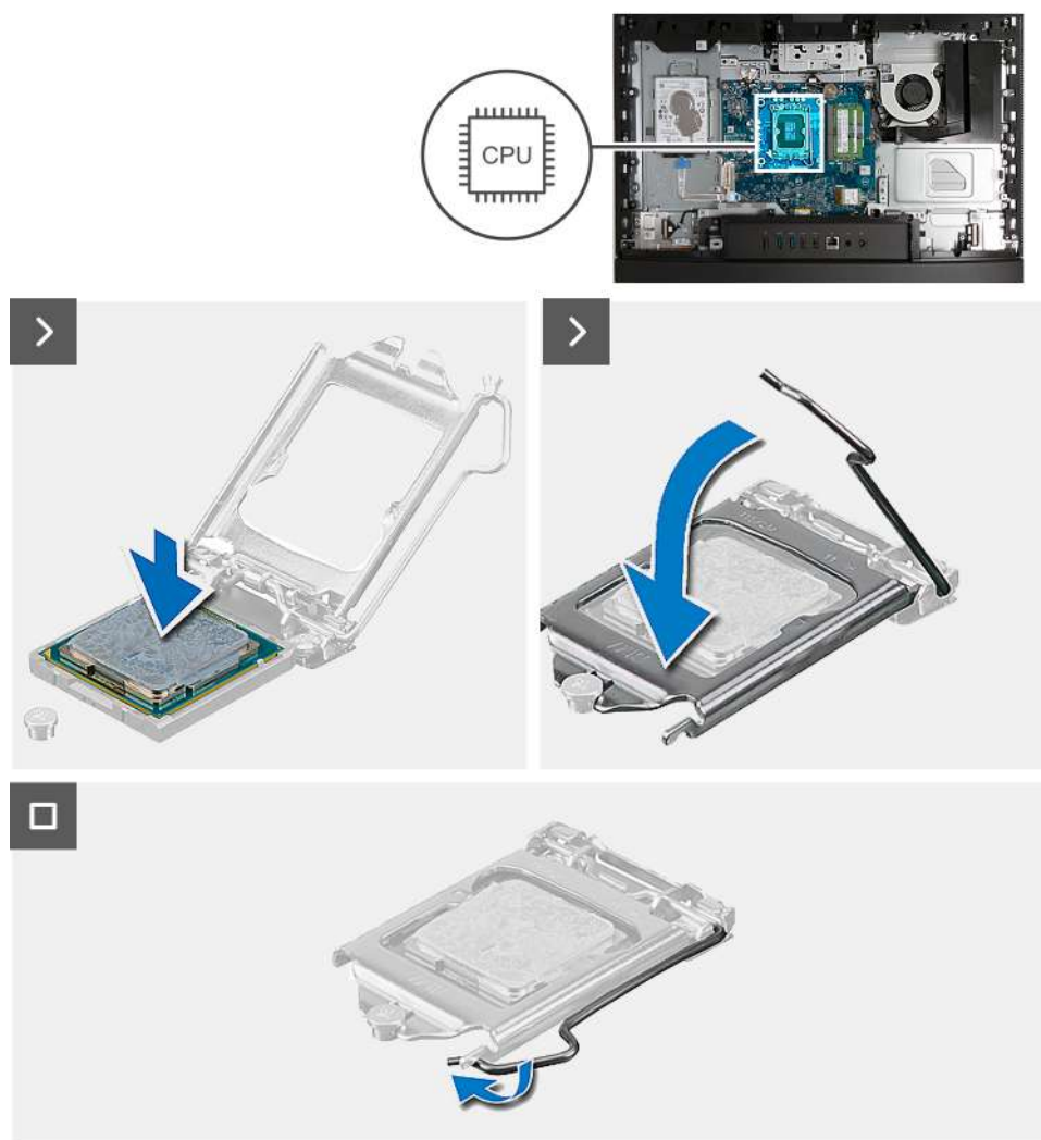
Obrázek 112. Montáž procesoru
