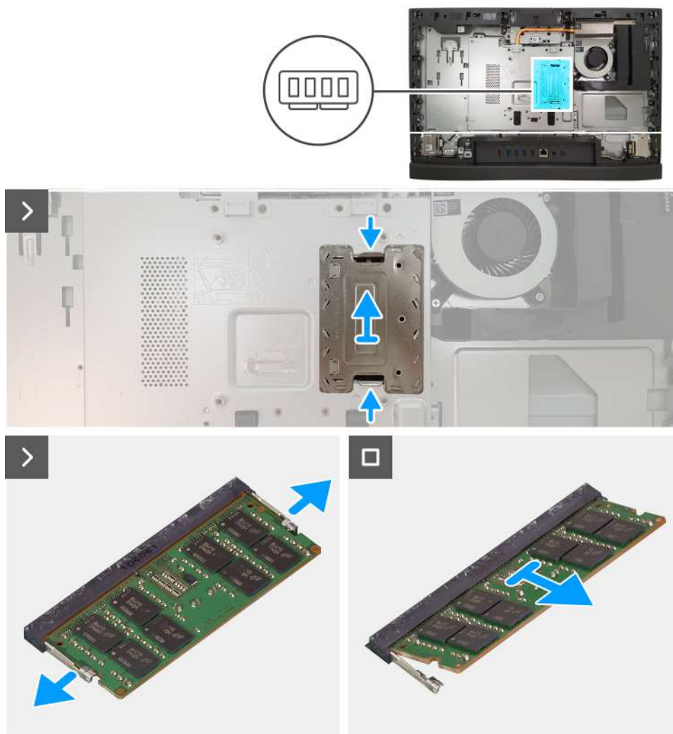
Obrázek 84. Vyjmutí paměti
