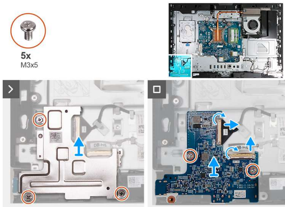
Obrázek 119. Demontáž desky vypínače a I/O
