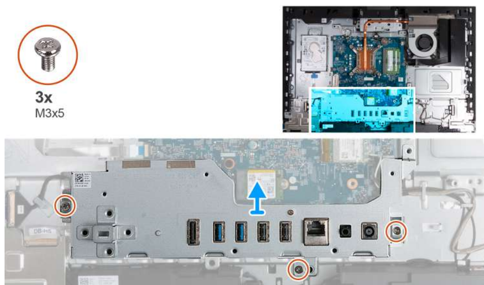
Obrázek 105. Demontáž držáku panelu I/O
