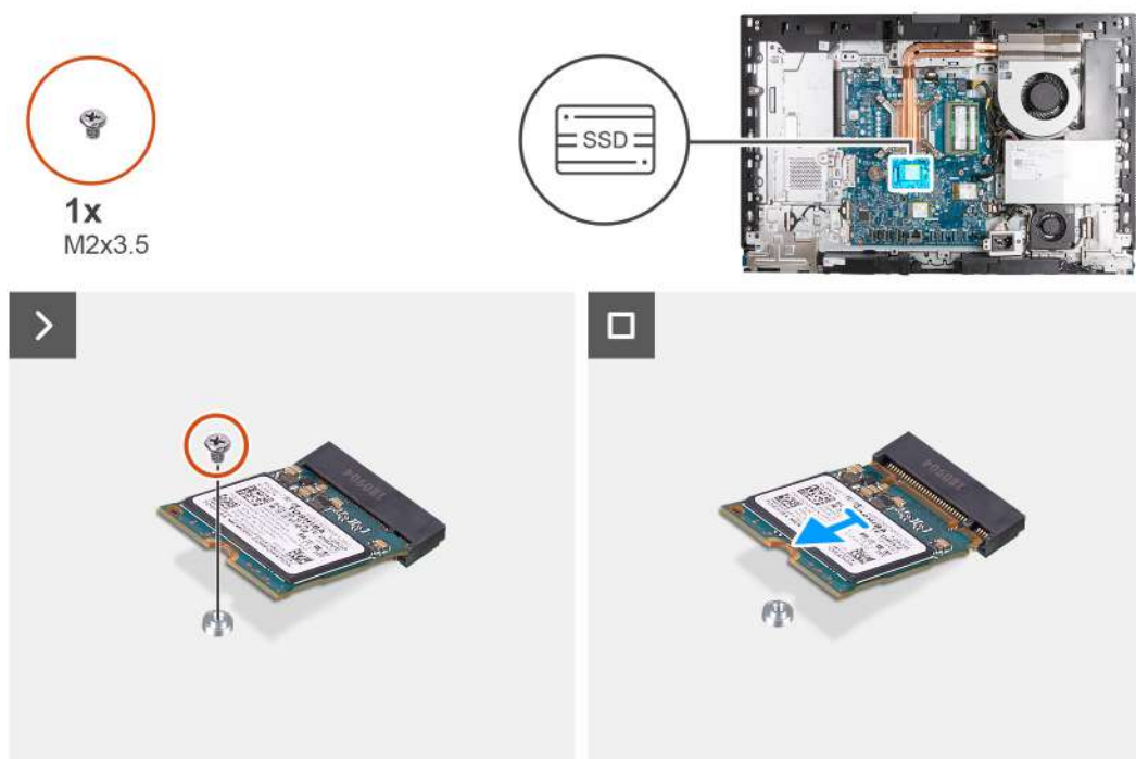
Obrázek 30. Demontáž disku SSD M.2 2230 ze slotu M.2 č. 0
