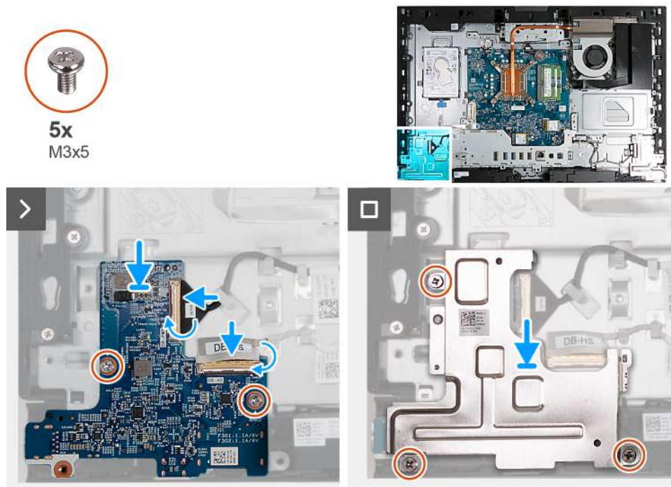
Obrázek 120. Montáž desky vypínače a I/O
