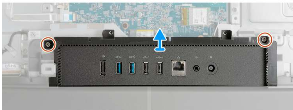
Obrázek 97. Demontáž krytu I/O
