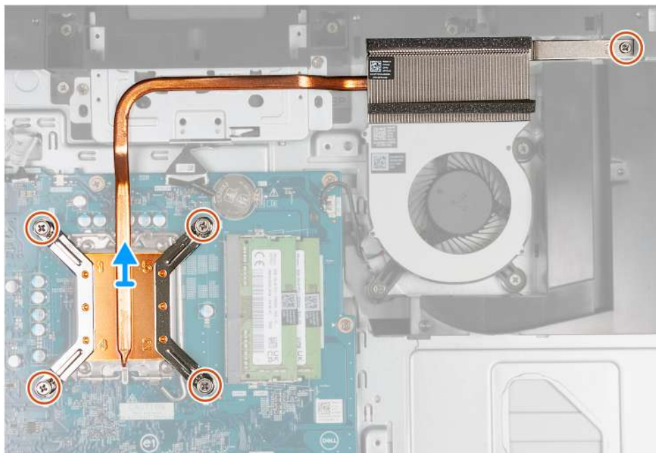
Obrázek 109. Demontáž chladiče
