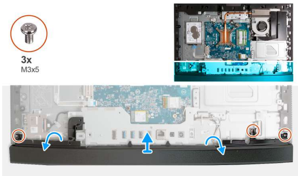
Obrázek 99. Sejmutí spodního krytu
