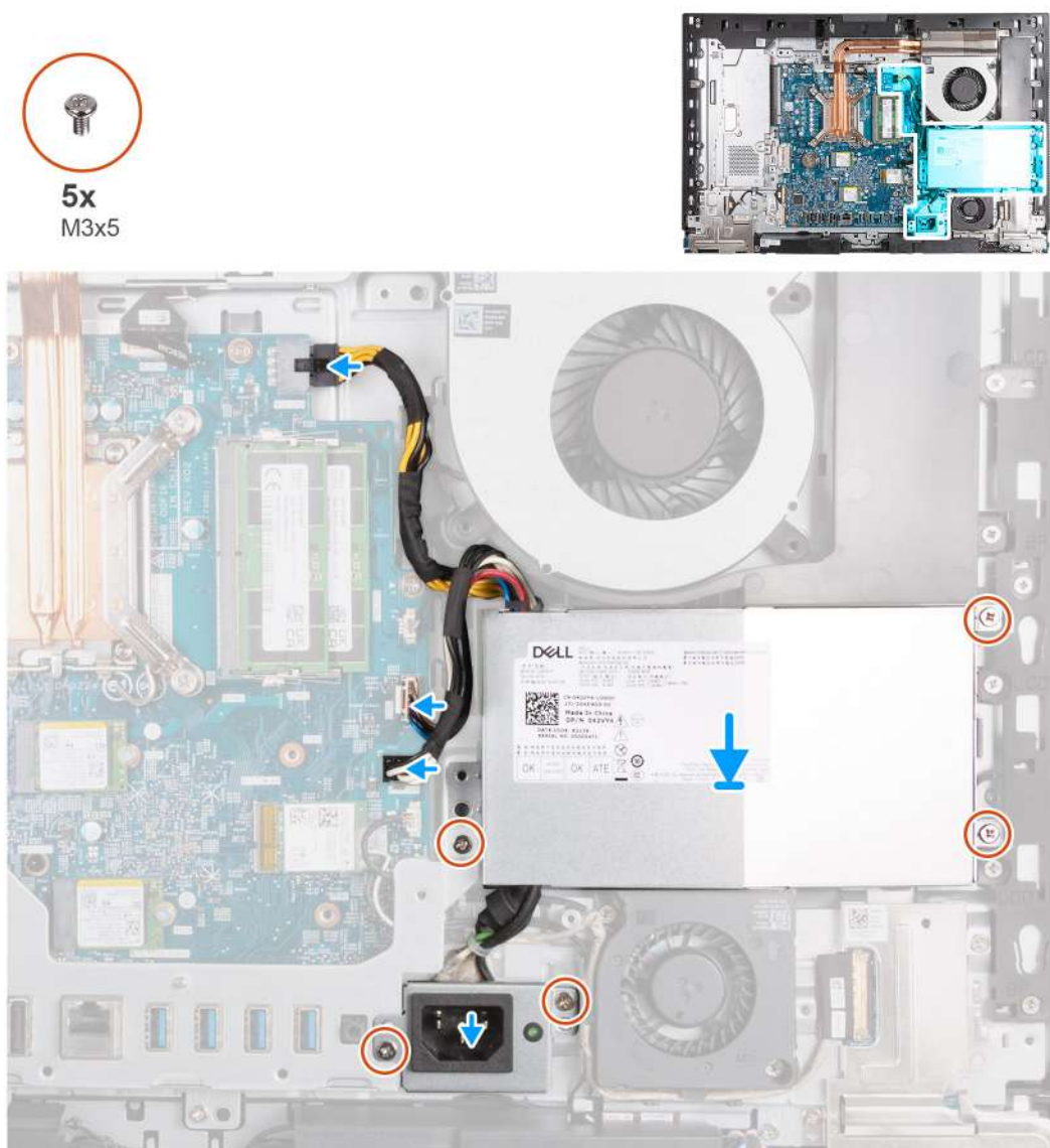
Obrázek 51. Montáž napájecí jednotky
