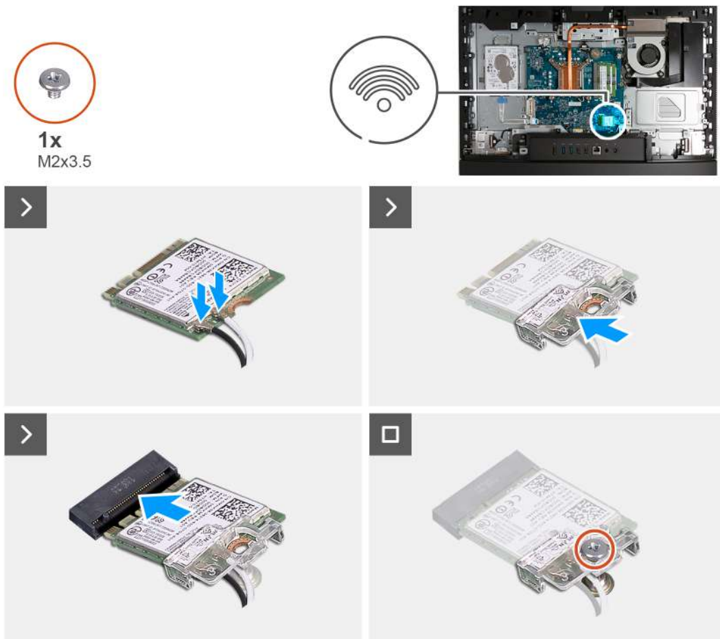
Obrázek 89. Montáž bezdrátové karty
