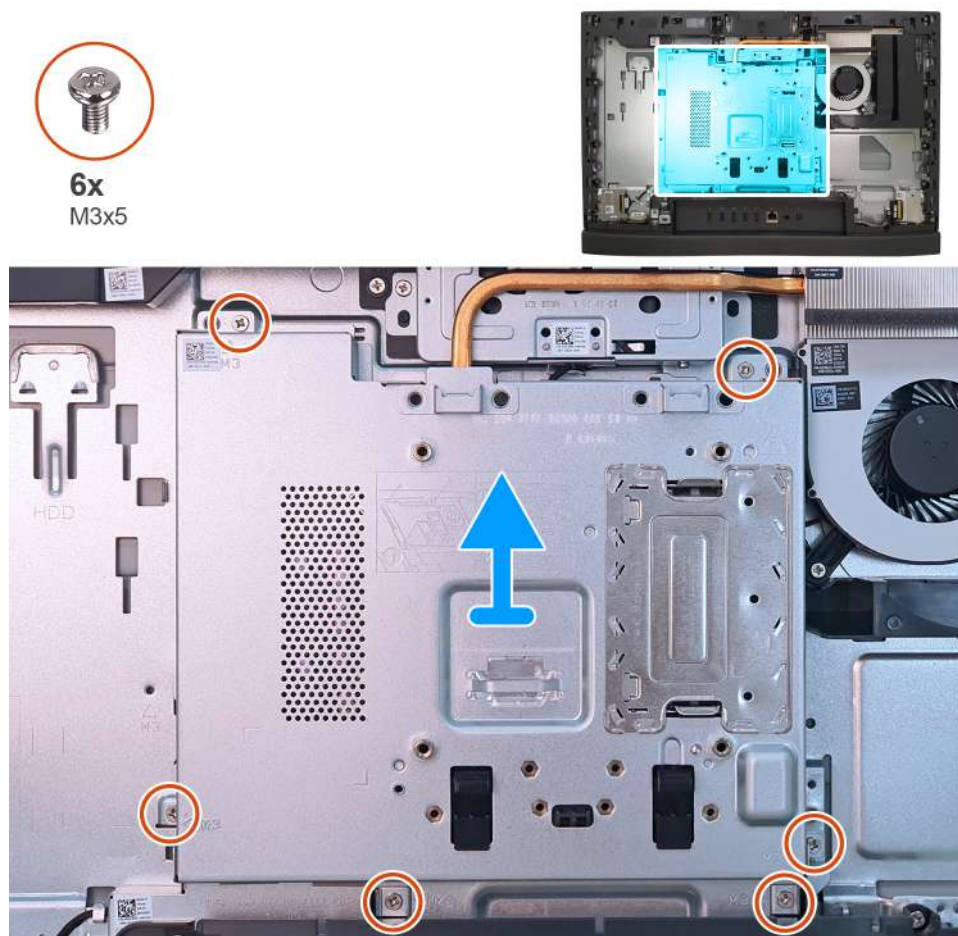
Obrázek 86. Demontáž krytu základní desky
