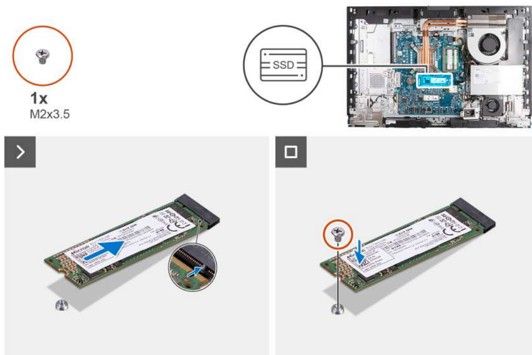
Obrázek 33. Montáž disku SSD M.2 2280 do slotu M.2 č. 0
