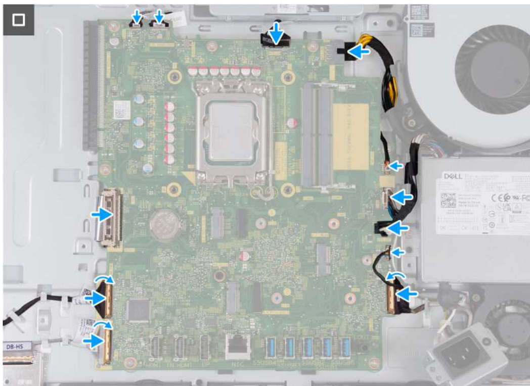
Obrázek 71. Montáž základní desky
