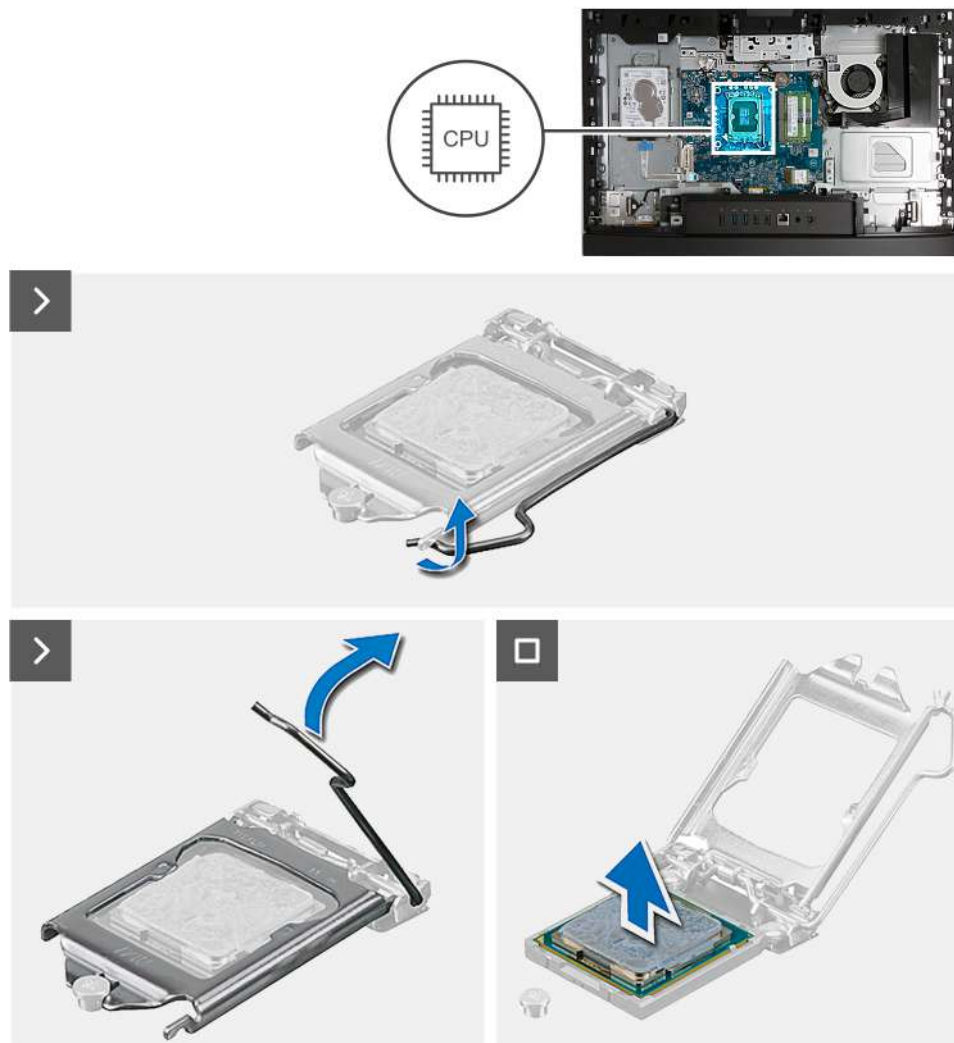
Obrázek 111. Demontáž procesoru
