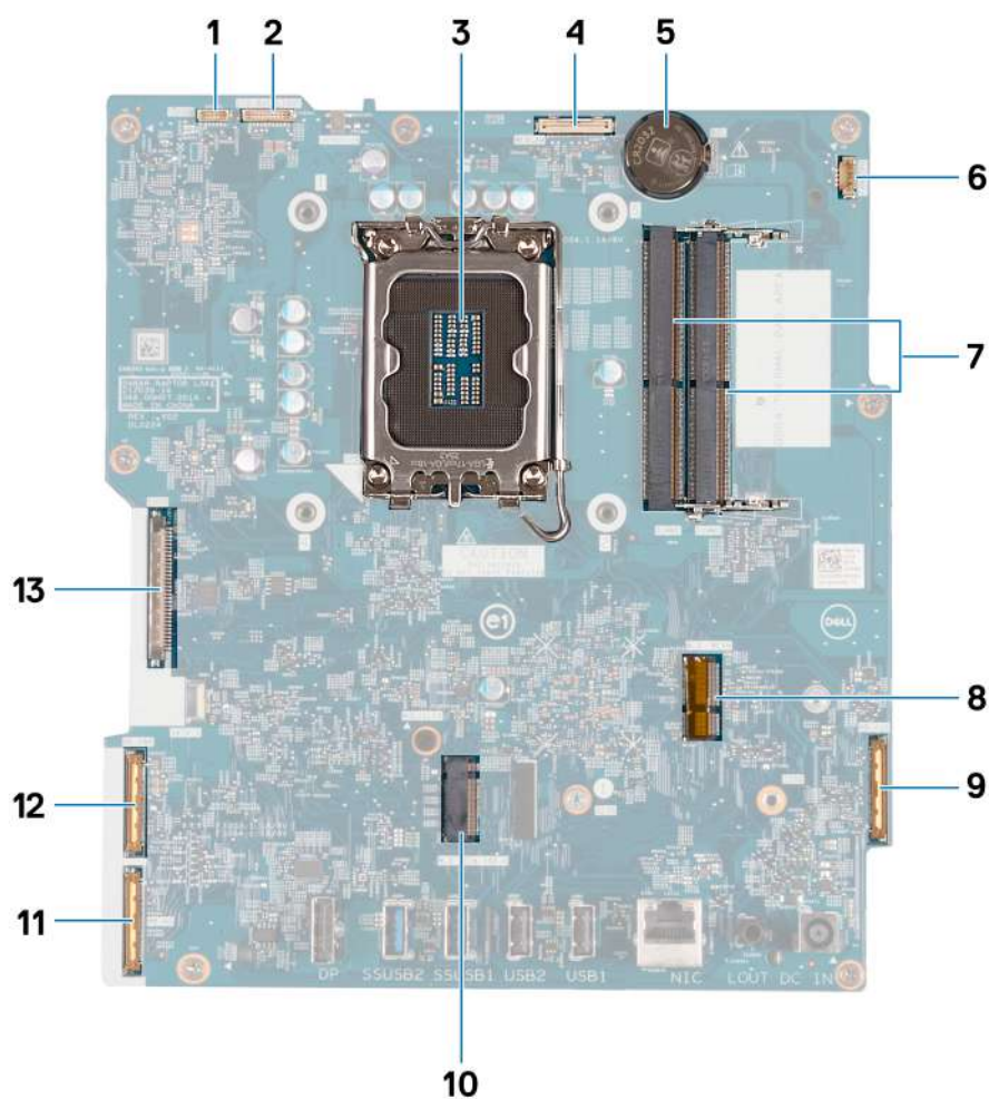
Obrázek 116. Popisky základní desky
