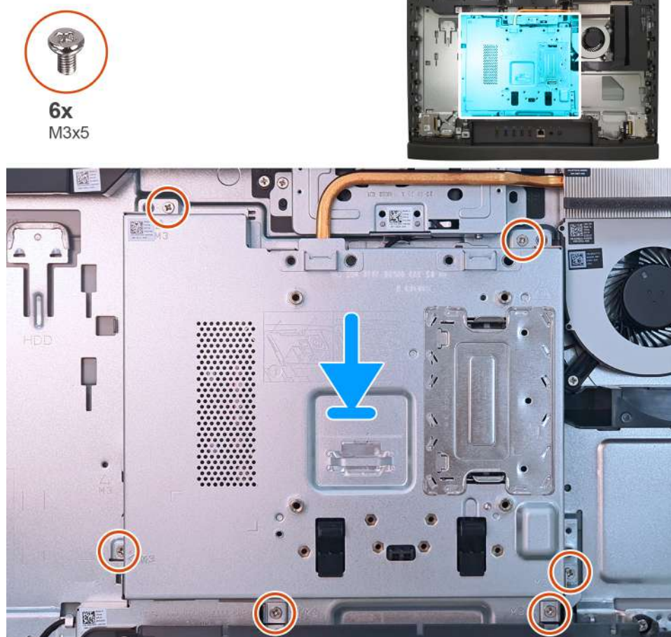
Obrázek 87. Montáž krytu základní desky
