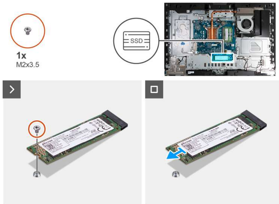
Obrázek 92. Demontáž disku SSD M.2 2280
