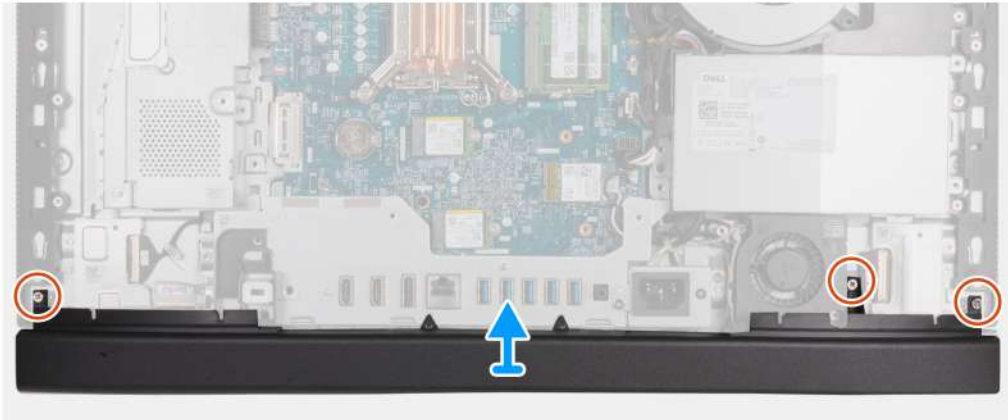
Obrázek 44. Sejmutí spodního krytu
