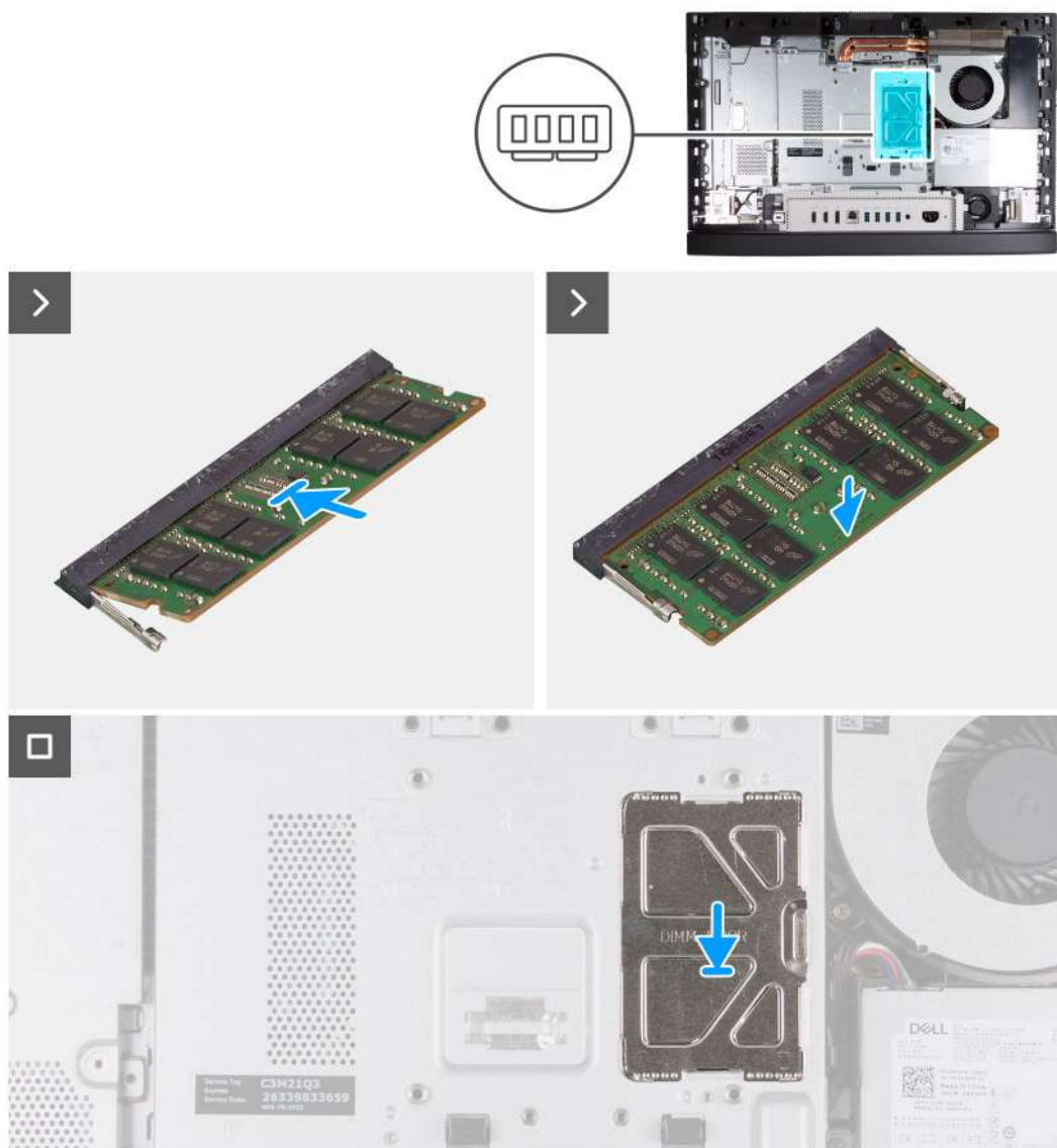
Obrázek 25. Instalace paměti
