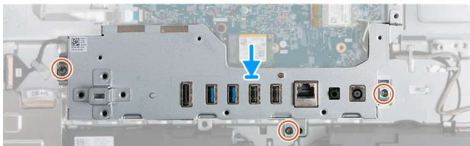
Obrázek 106. Montáž držáku I/O
