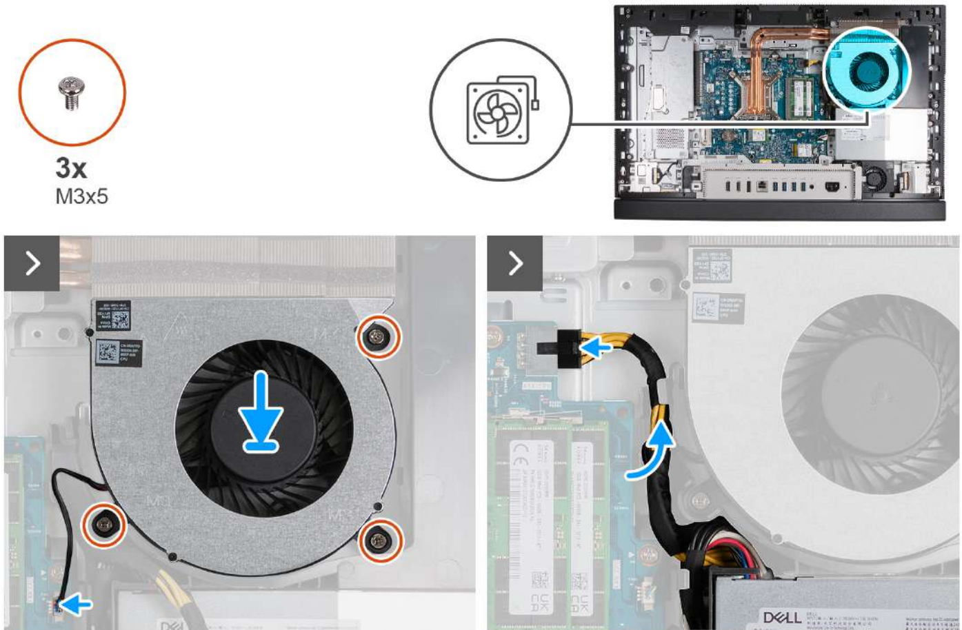
Obrázek 49. Montáž ventilátoru
