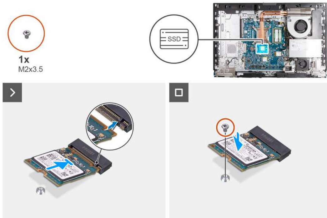
Obrázek 31. Montáž disku SSD M.2 2230 do slotu M.2 č. 0
