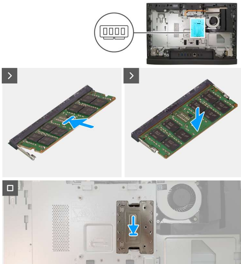
Obrázek 85. Instalace paměti
