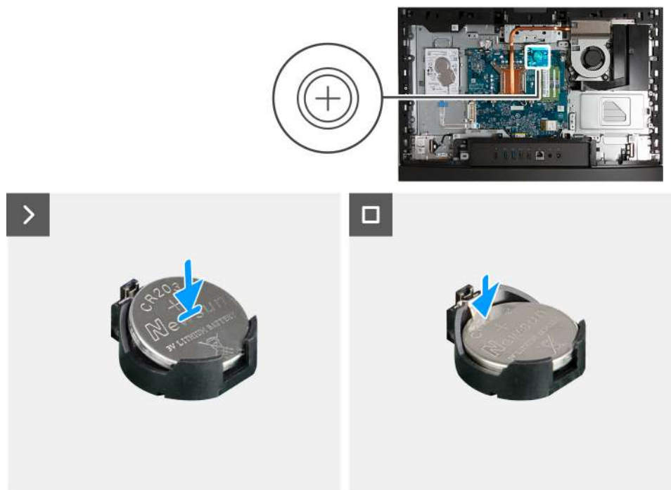
Obrázek 96. Montáž knoflíkové baterie
