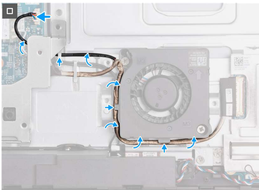
Obrázek 57. Montáž ventilátoru napájecího zdroje
