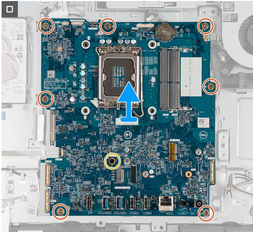
Obrázek 115. Demontáž základní desky
