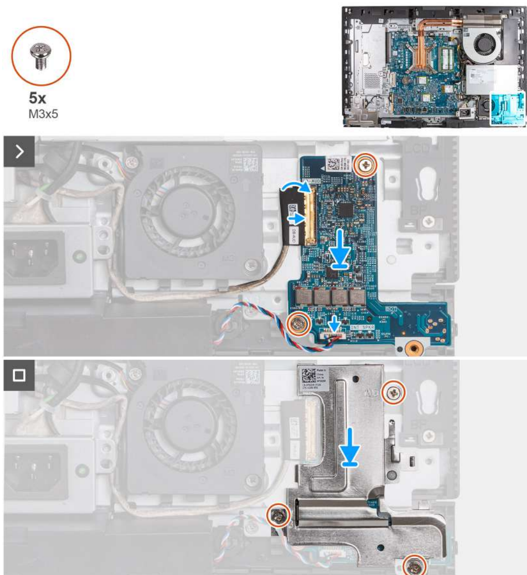
Obrázek 75. Montáž zvukové karty
