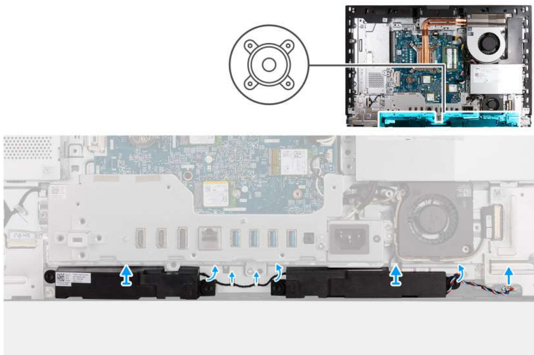
Obrázek 60. Demontáž reproduktorů
