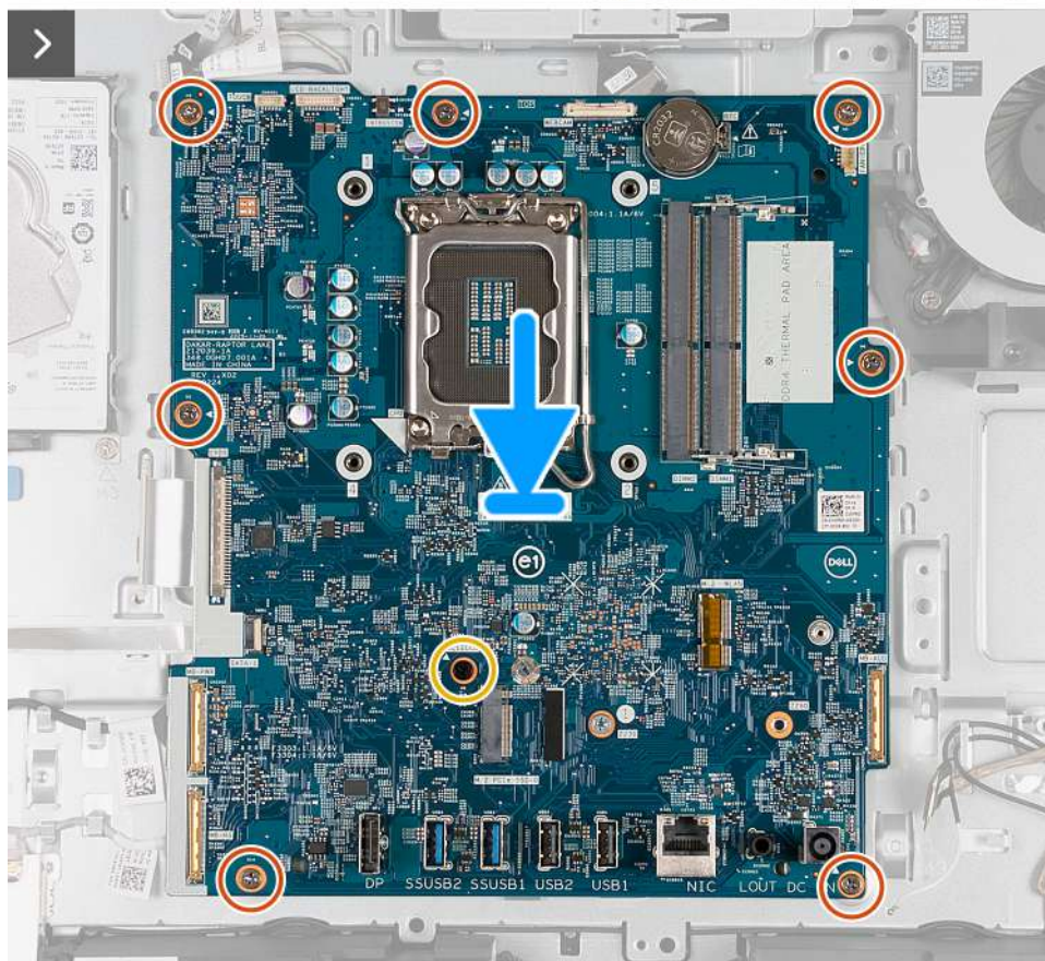
Obrázek 117. Montáž základní desky
