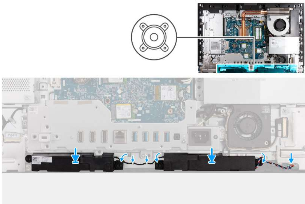
Obrázek 61. Montáž reproduktorů
