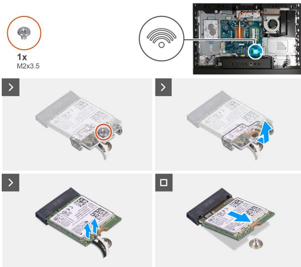
Obrázek 88. Demontáž bezdrátové karty
