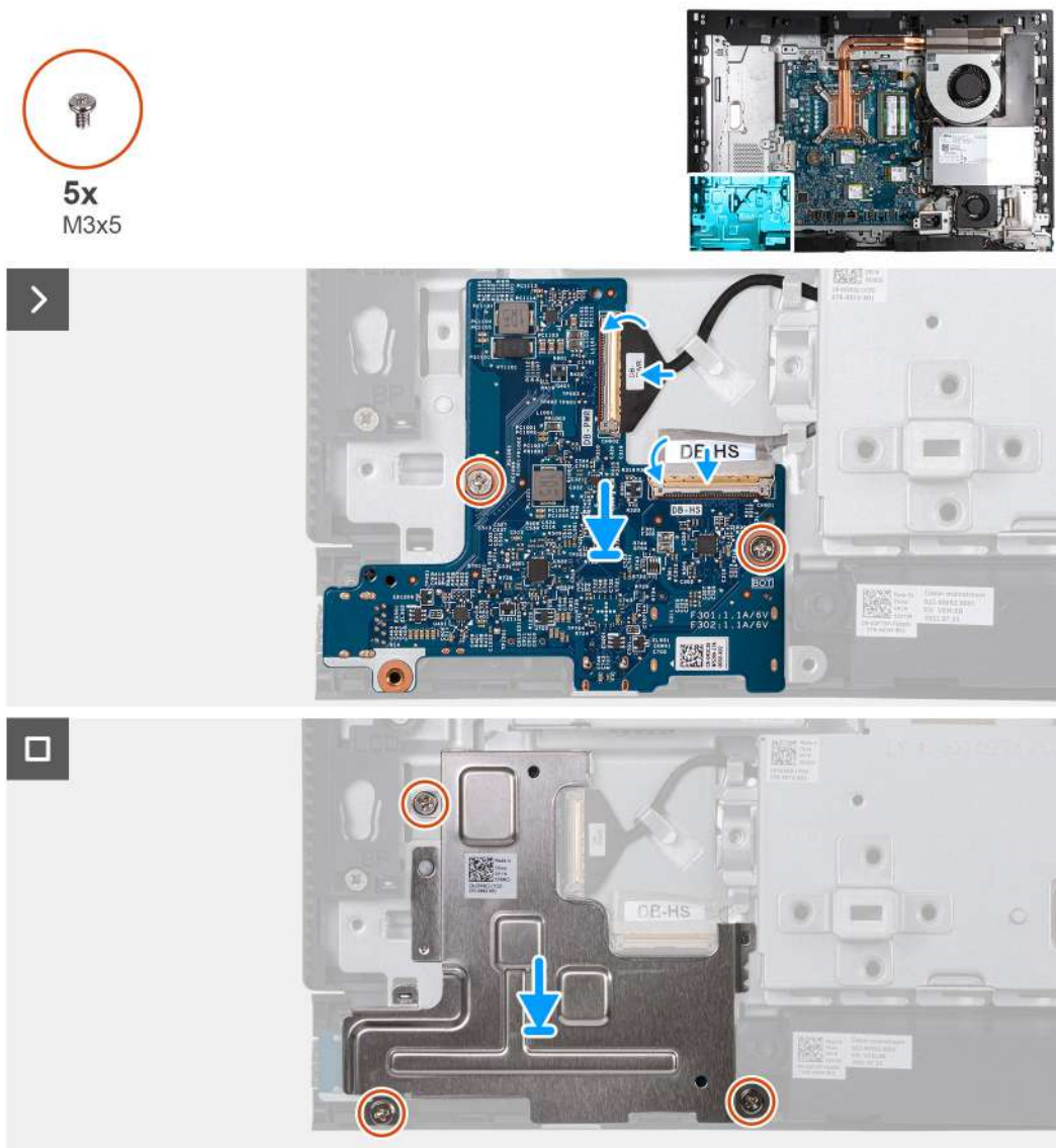
Obrázek 73. Montáž vypínače a desky I/O
