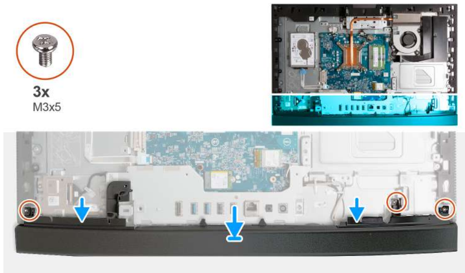
Obrázek 100. Montáž spodního krytu
