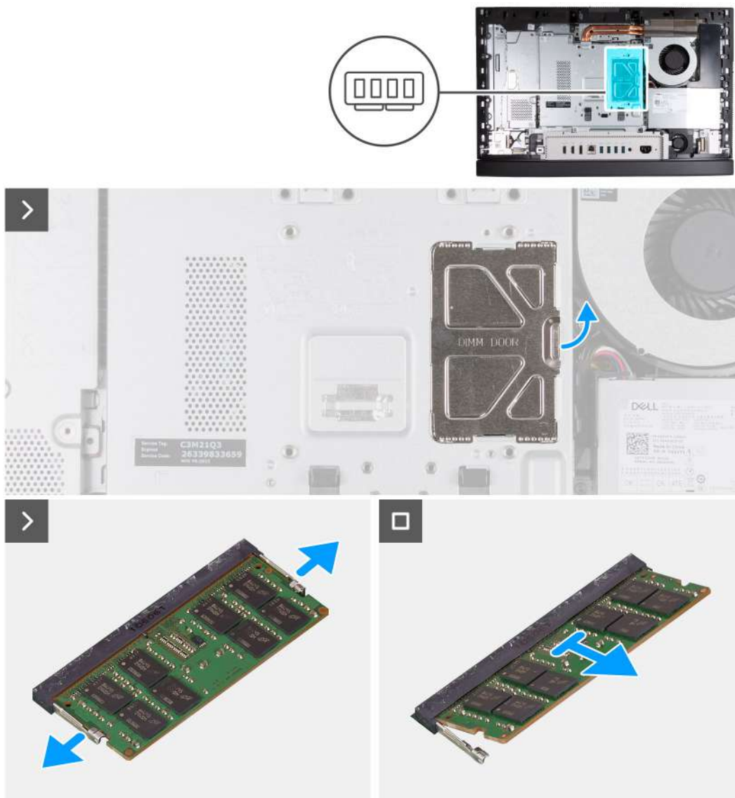
Obrázek 24. Vyjmutí paměti
