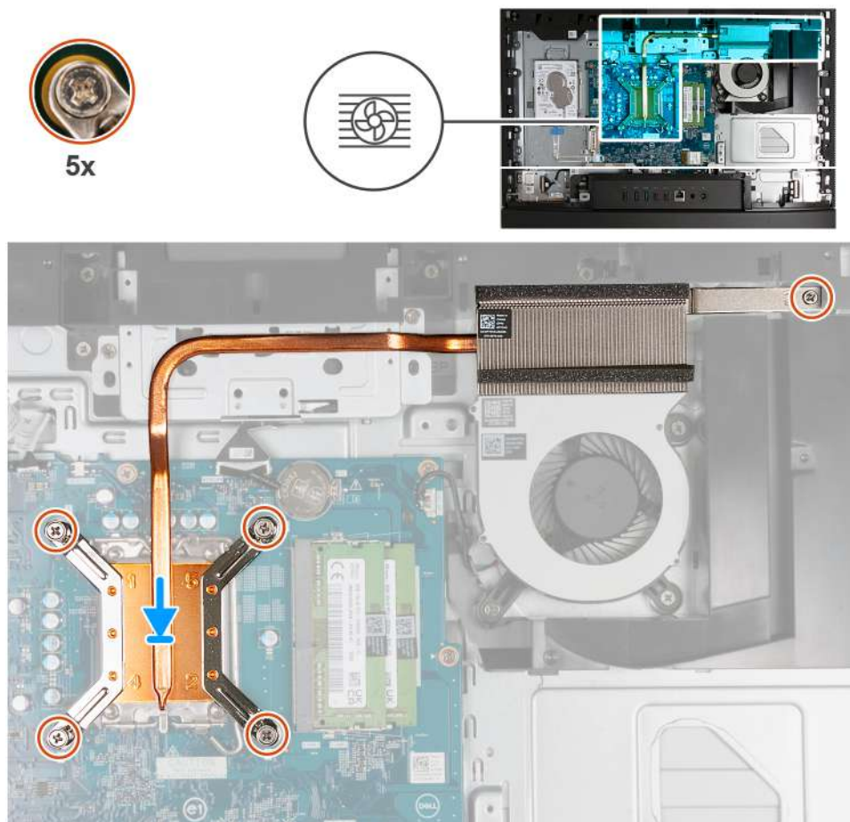
Obrázek 110. Montáž chladiče
