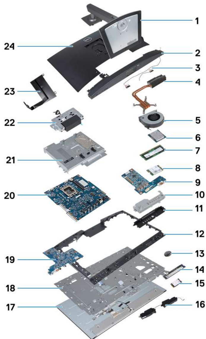
Obrázek 17. Hlavní komponenty počítače OptiPlex All-in-One 7420 s úsporným procesorem
