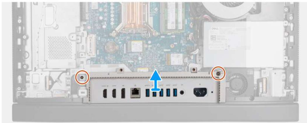
Obrázek 42. Demontáž krytu I/O
