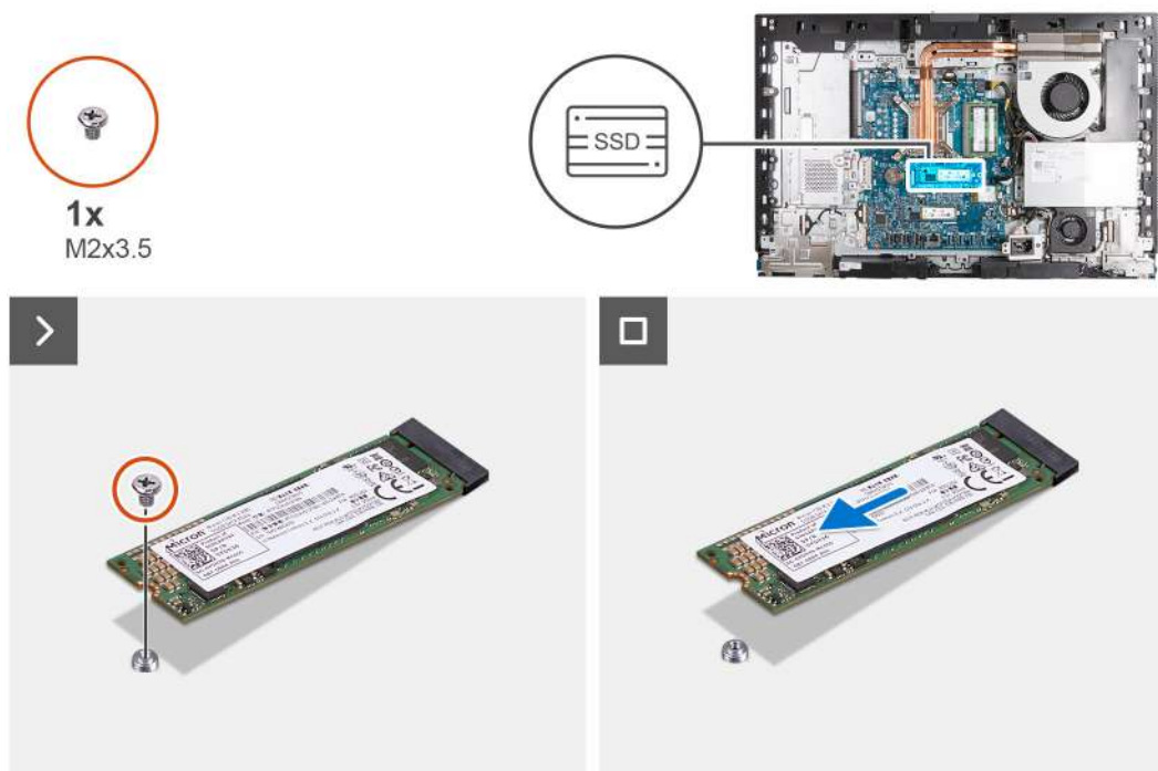
Obrázek 32. Demontáž disku SSD M.2 2280 ze slotu M.2 č. 0
