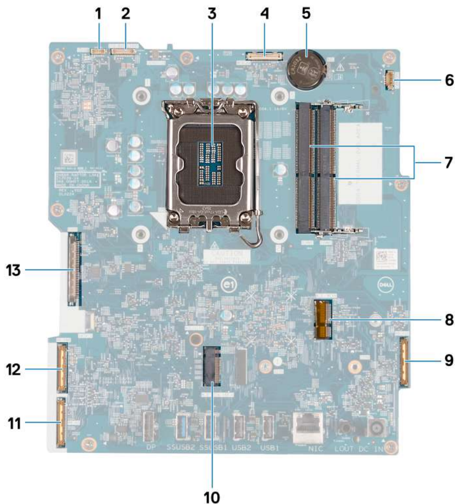
Obrázek 113. Popisky základní desky
