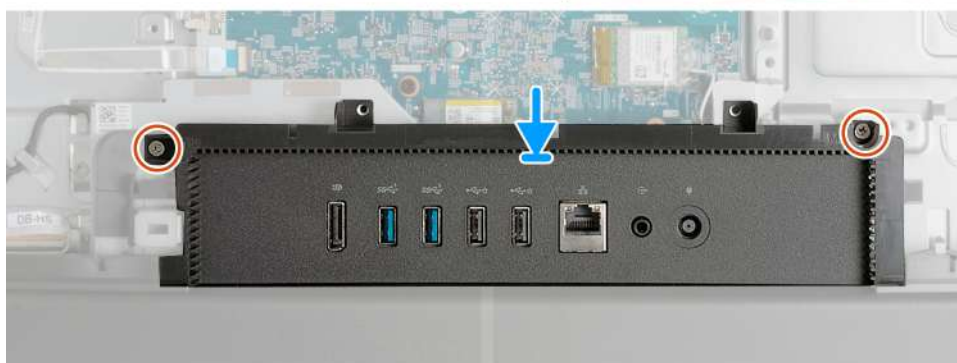
Obrázek 98. Montáž krytu I/O
