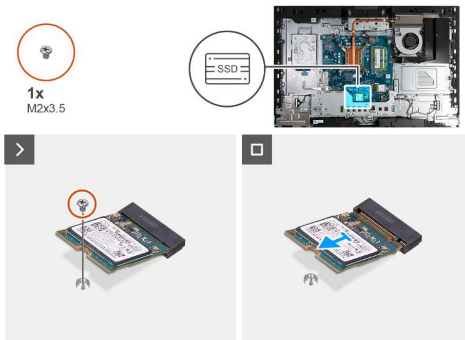
Obrázek 90. Demontáž disku SSD M.2 2230
