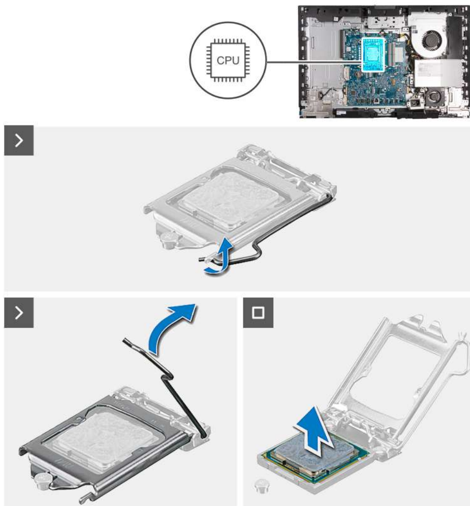
Obrázek 64. Demontáž procesoru
