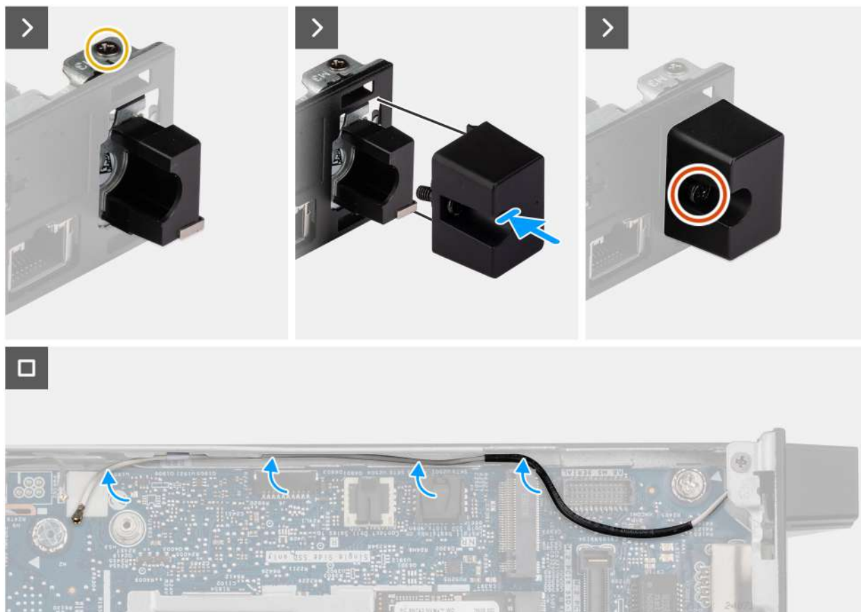
Obrázek 65. Montáž anténního modulu (bílý kabel)
