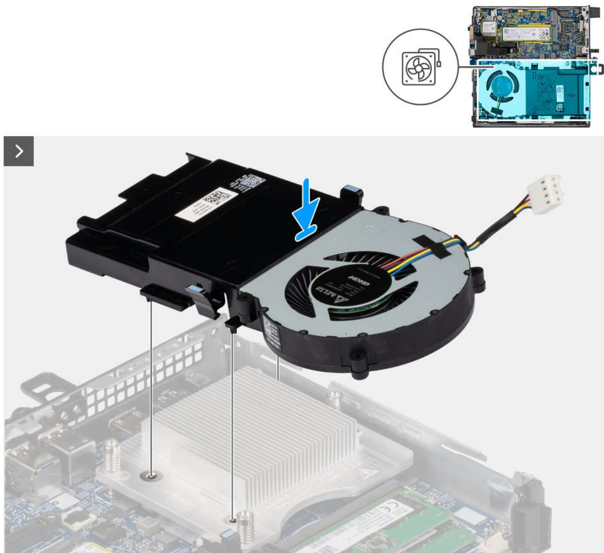
Obrázek 30. Montáž ventilátoru
