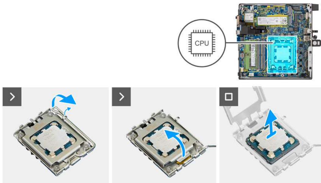
Obrázek 68. Demontáž procesoru
