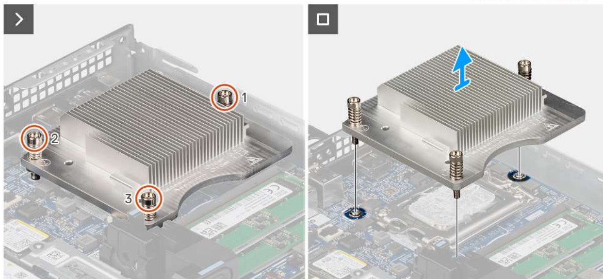
Obrázek 60. Demontáž chladiče
