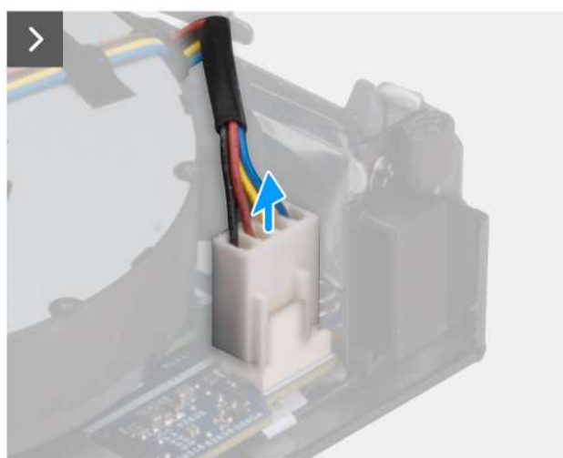
Obrázek 28. Demontáž ventilátoru
