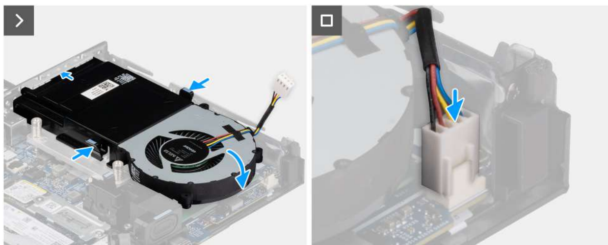
Obrázek 31. Montáž ventilátoru
