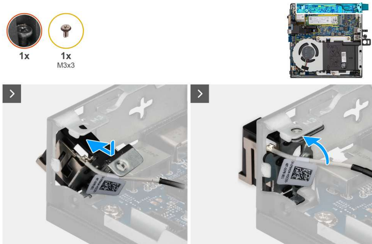
Obrázek 64. Montáž anténního modulu (bílý kabel)
