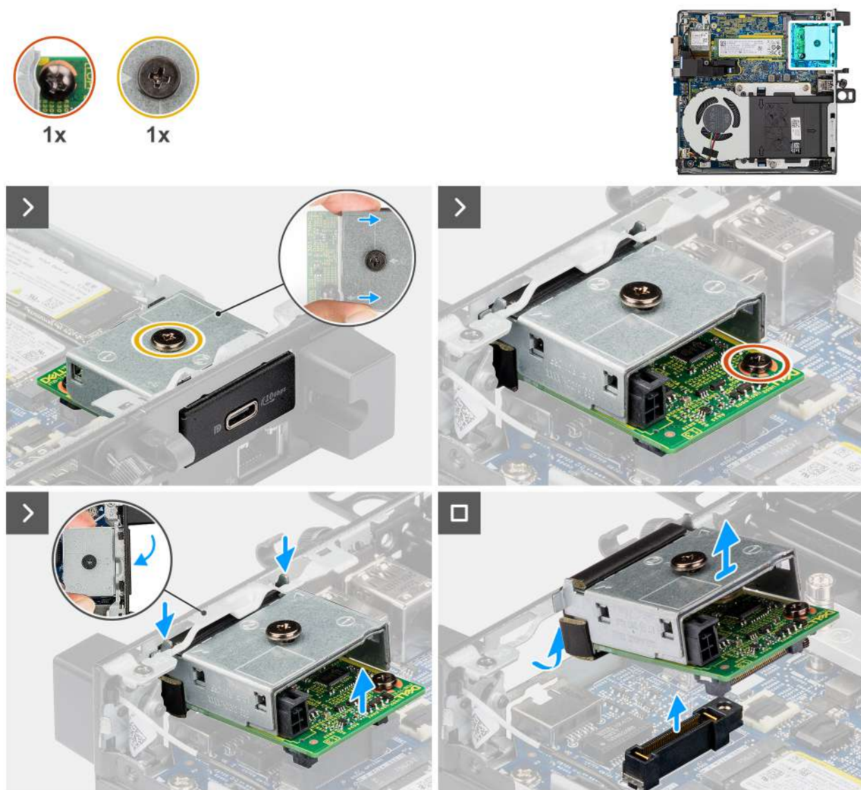
Obrázek 41. Demontáž modulu USB Type-C
