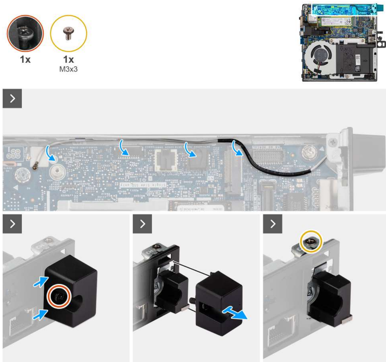
Obrázek 62. Demontáž anténního modulu (bílý kabel)
