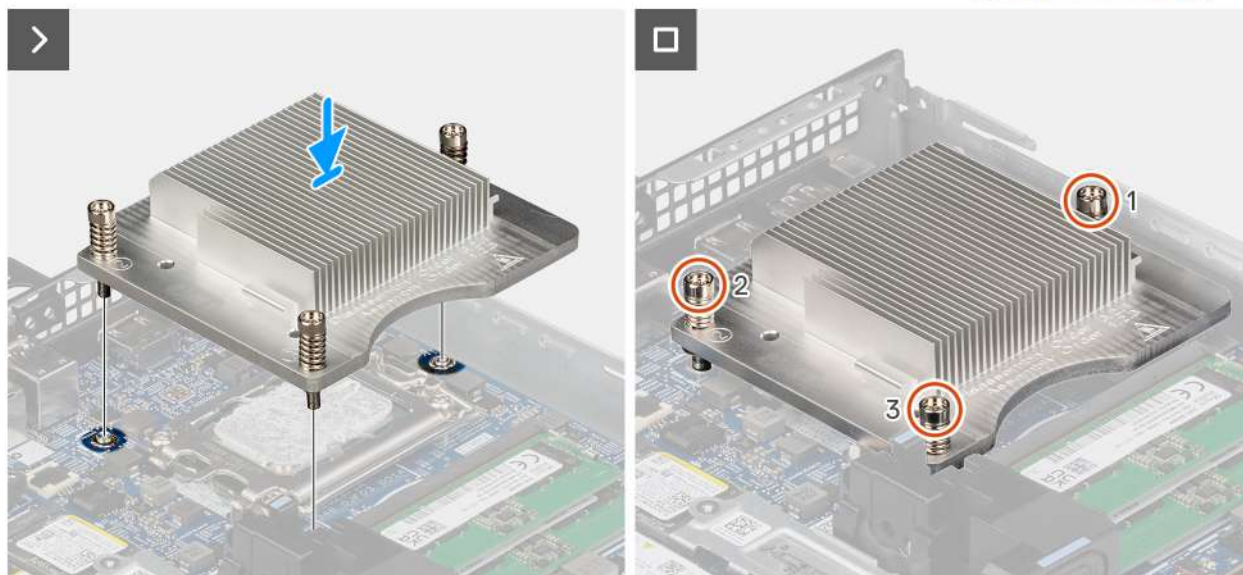
Obrázek 61. Montáž chladiče
