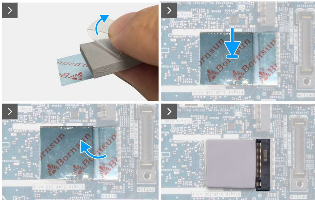
Obrázek 20. Montáž disku SSD M.2 2280
