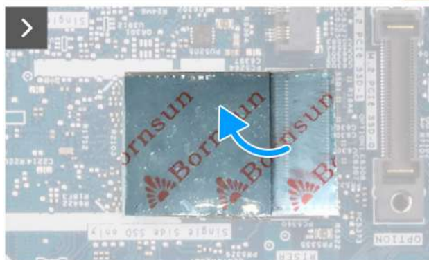
Obrázek 17. Montáž disku SSD 2230
