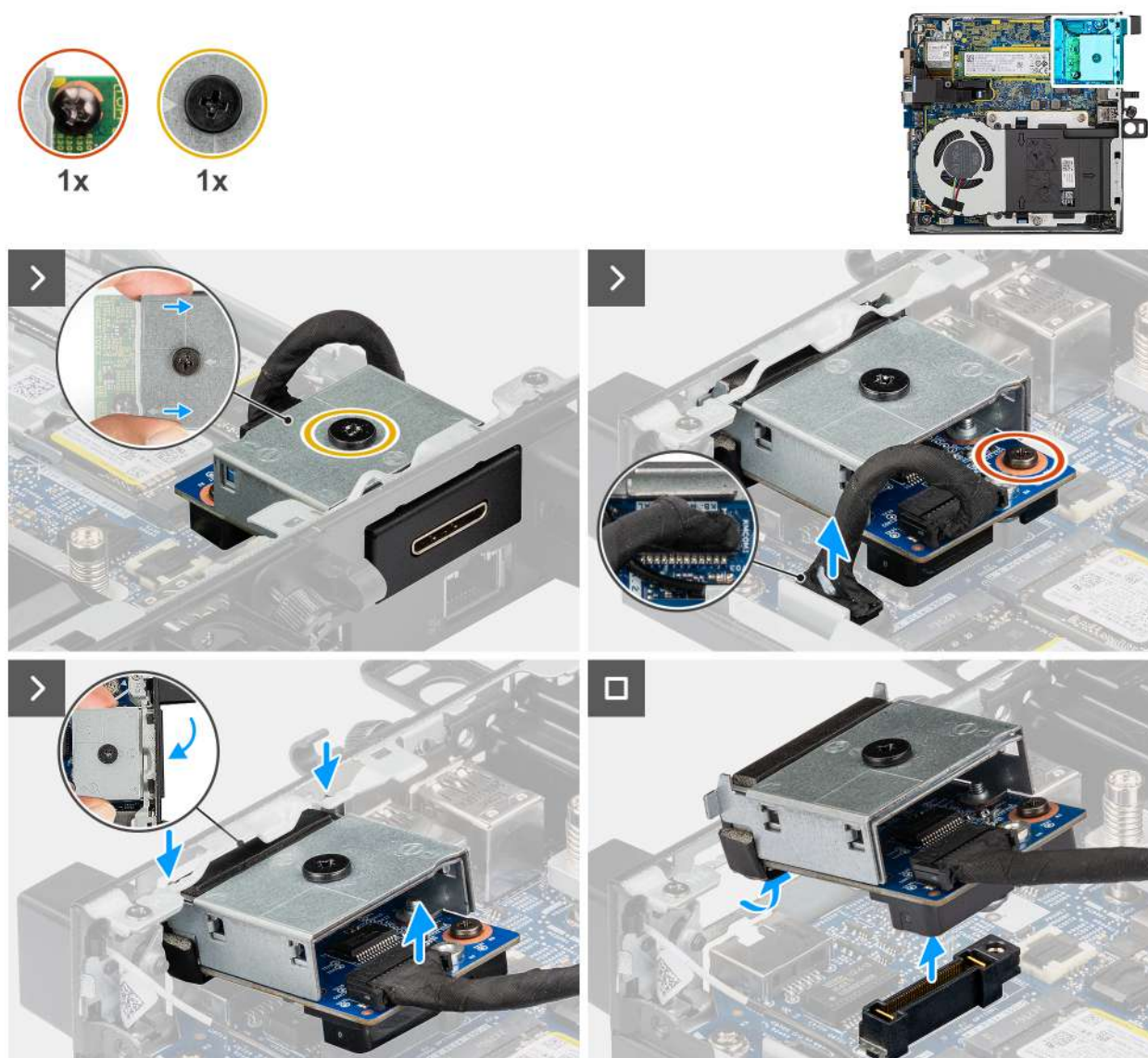
Obrázek 51. Demontáž modulu PS2
