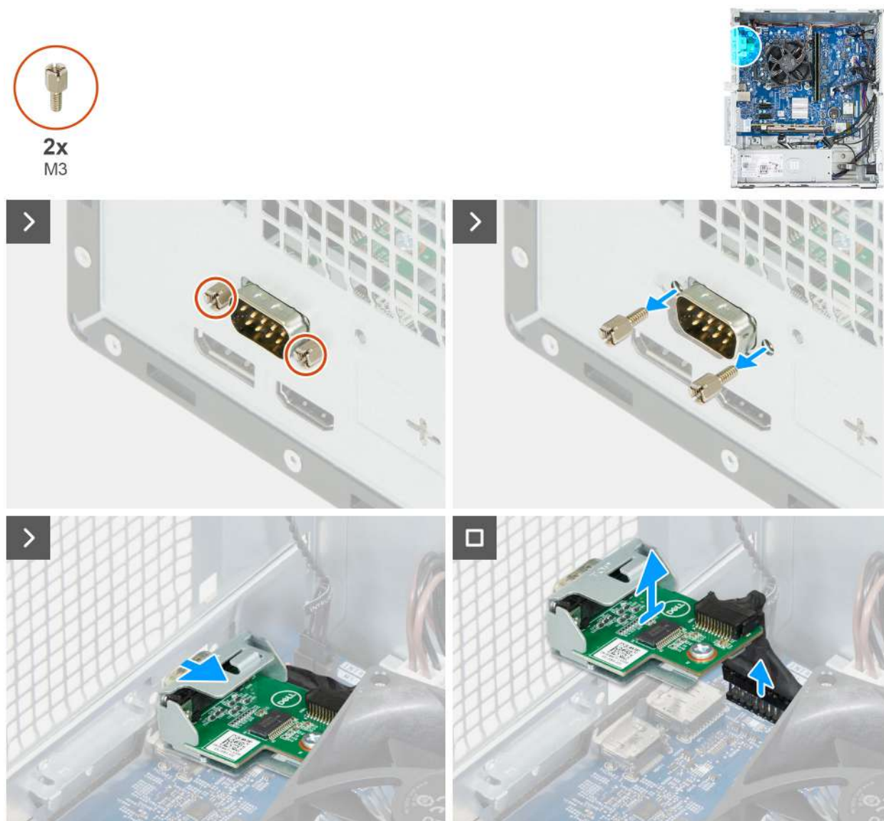
Obrázek 51. Demontáž modulu sériového portu
