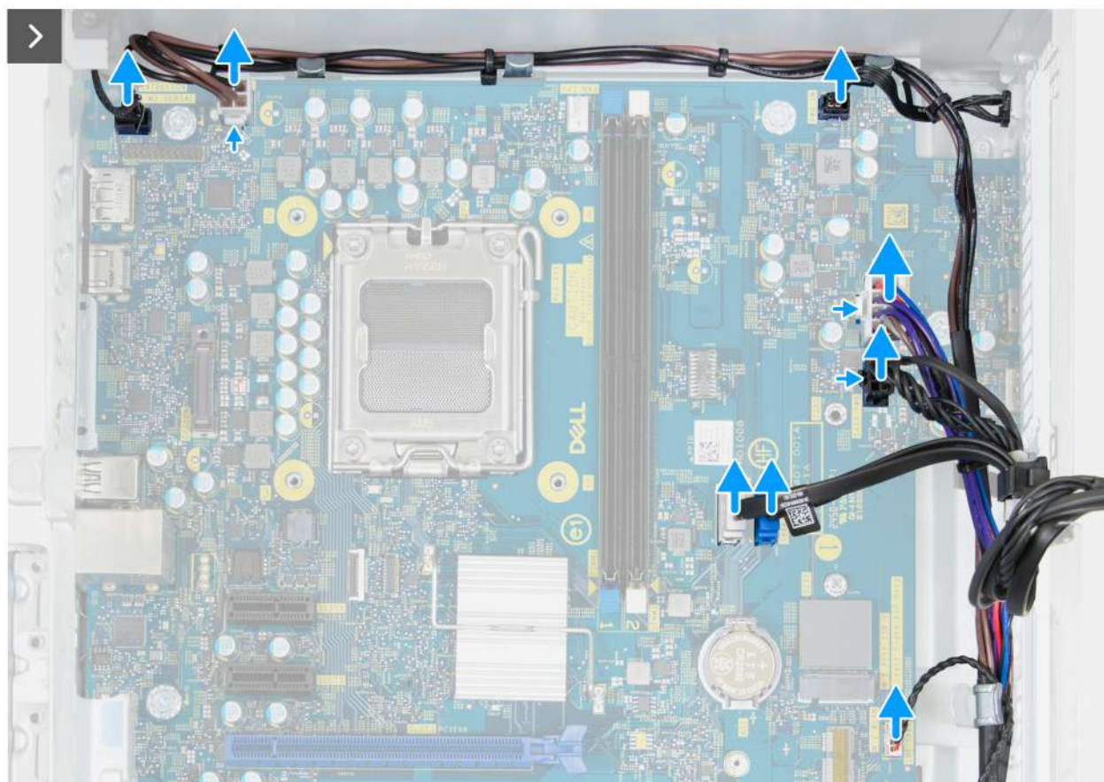
Obrázek 68. Demontáž základní desky
