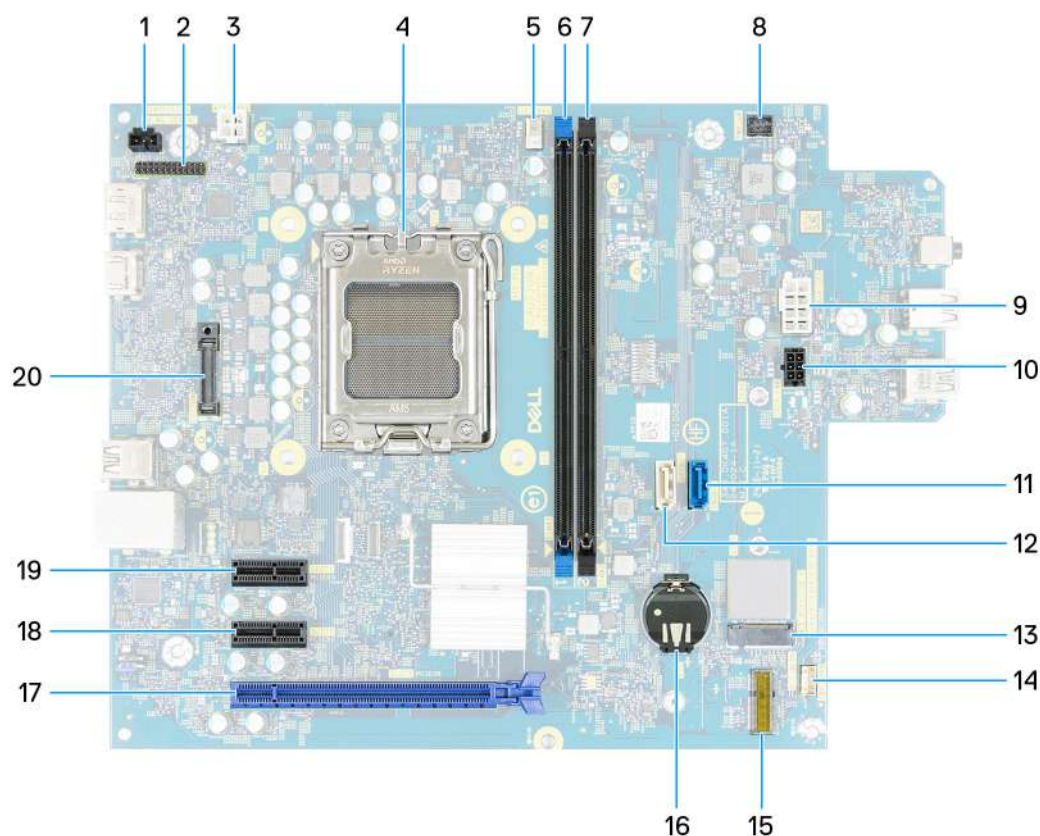
Obrázek 71. Popisky základní desky
