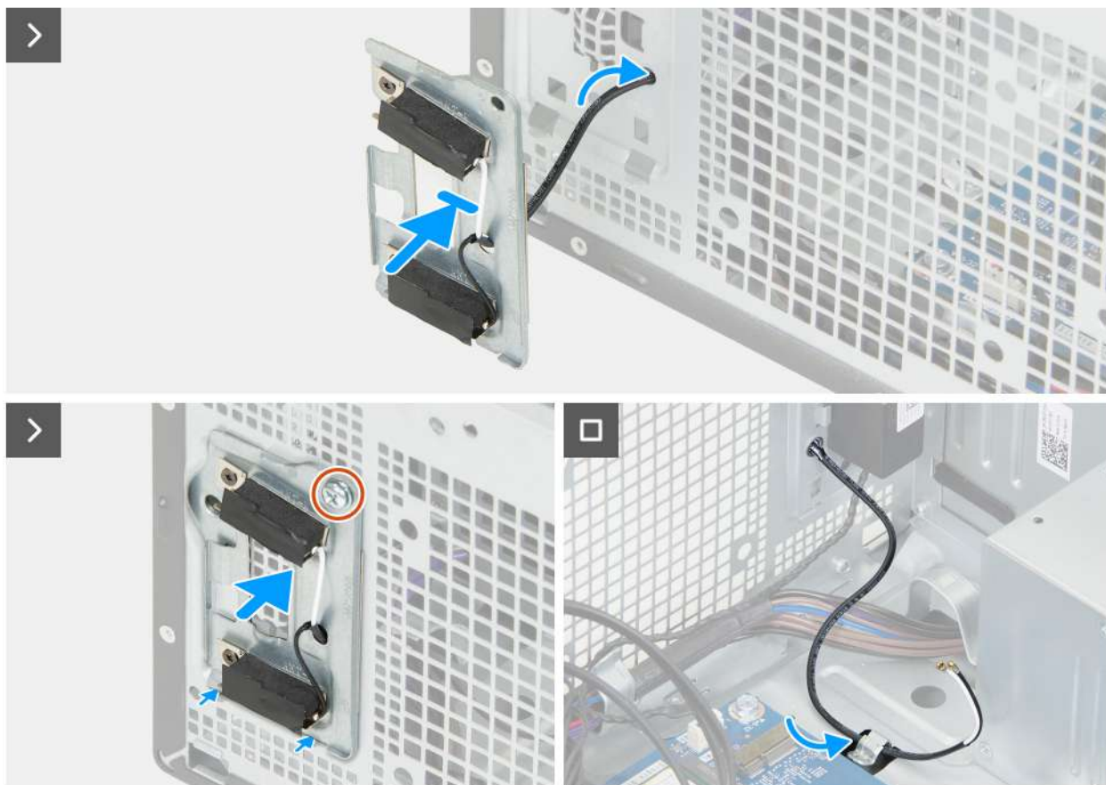
Obrázek 57. Montáž anténních modulů
