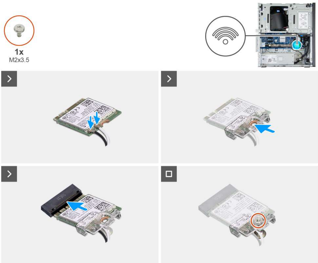
Obrázek 33. Montáž bezdrátové karty
