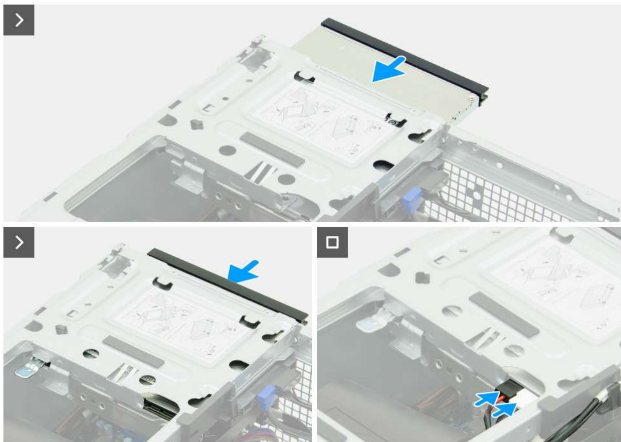
Obrázek 37. Montáž optické jednotky
