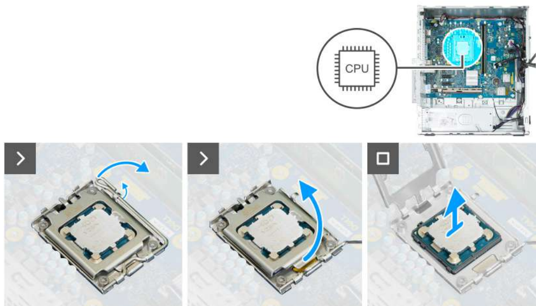
Obrázek 64. Demontáž procesoru
