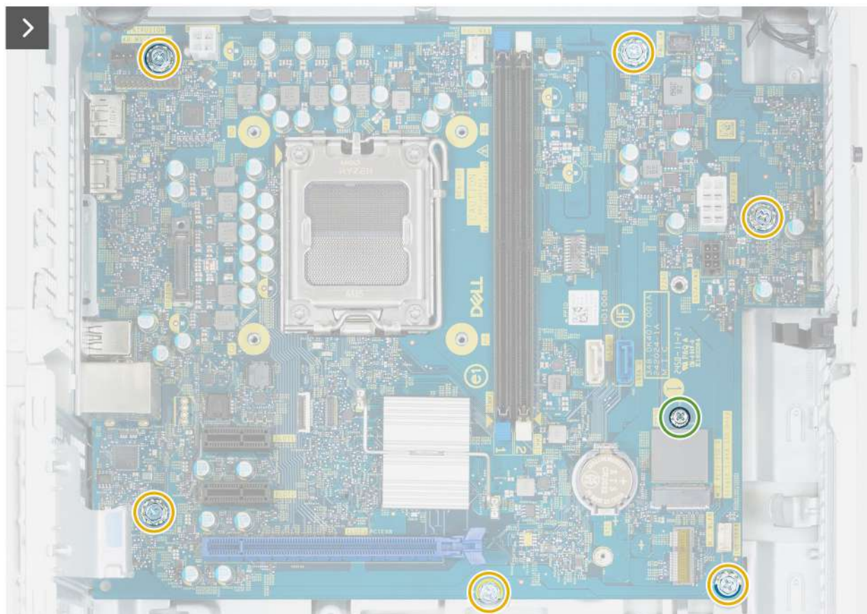
Obrázek 73. Montáž základní desky
