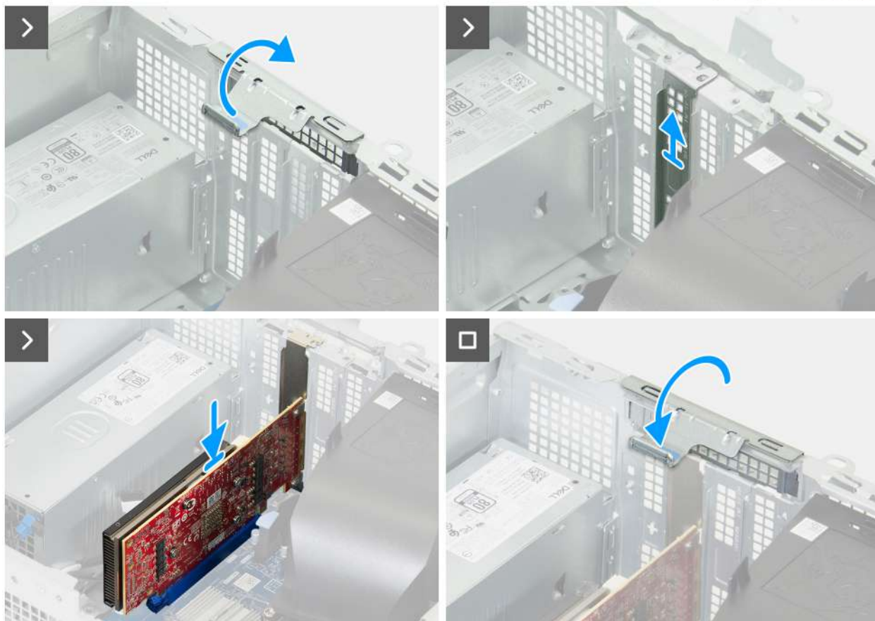
Obrázek 31. Montáž grafické karty
