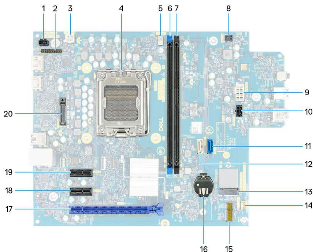
Obrázek 66. Popisky základní desky
