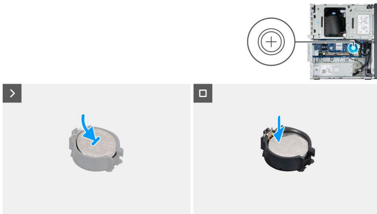
Obrázek 16. Montáž knoflíkové baterie
