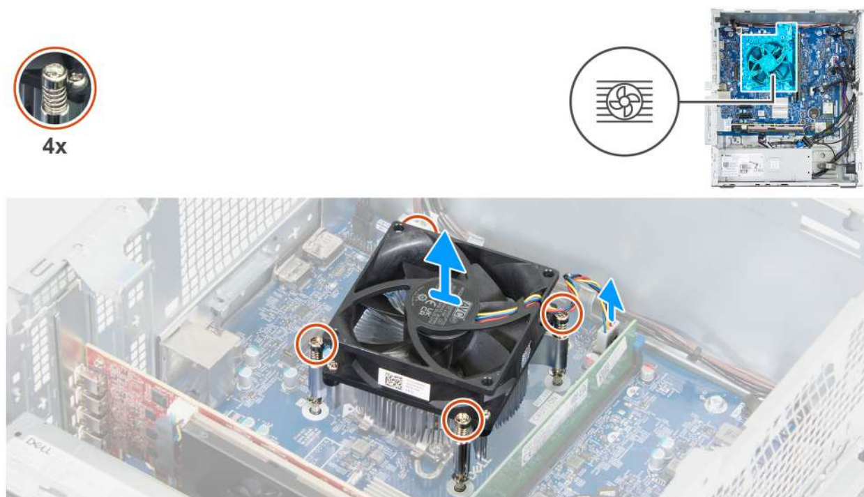
Obrázek 62. Demontáž sestavy ventilátoru a chladiče procesoru
