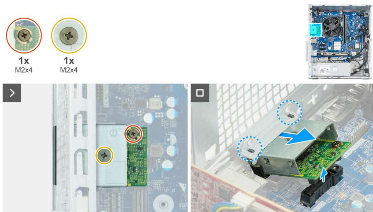
Obrázek 48. Odebrání modulu volitelného portu
