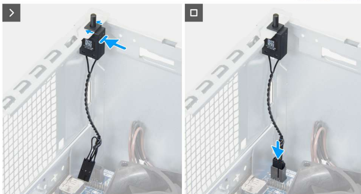
Obrázek 45. Montáž spínače detekce vniknutí do šasi
