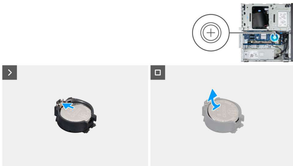
Obrázek 15. Vyjmutí knoflíkové baterie
