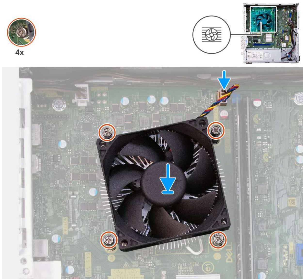
Obrázek 40. Montáž sestavy ventilátoru a chladiče procesoru
