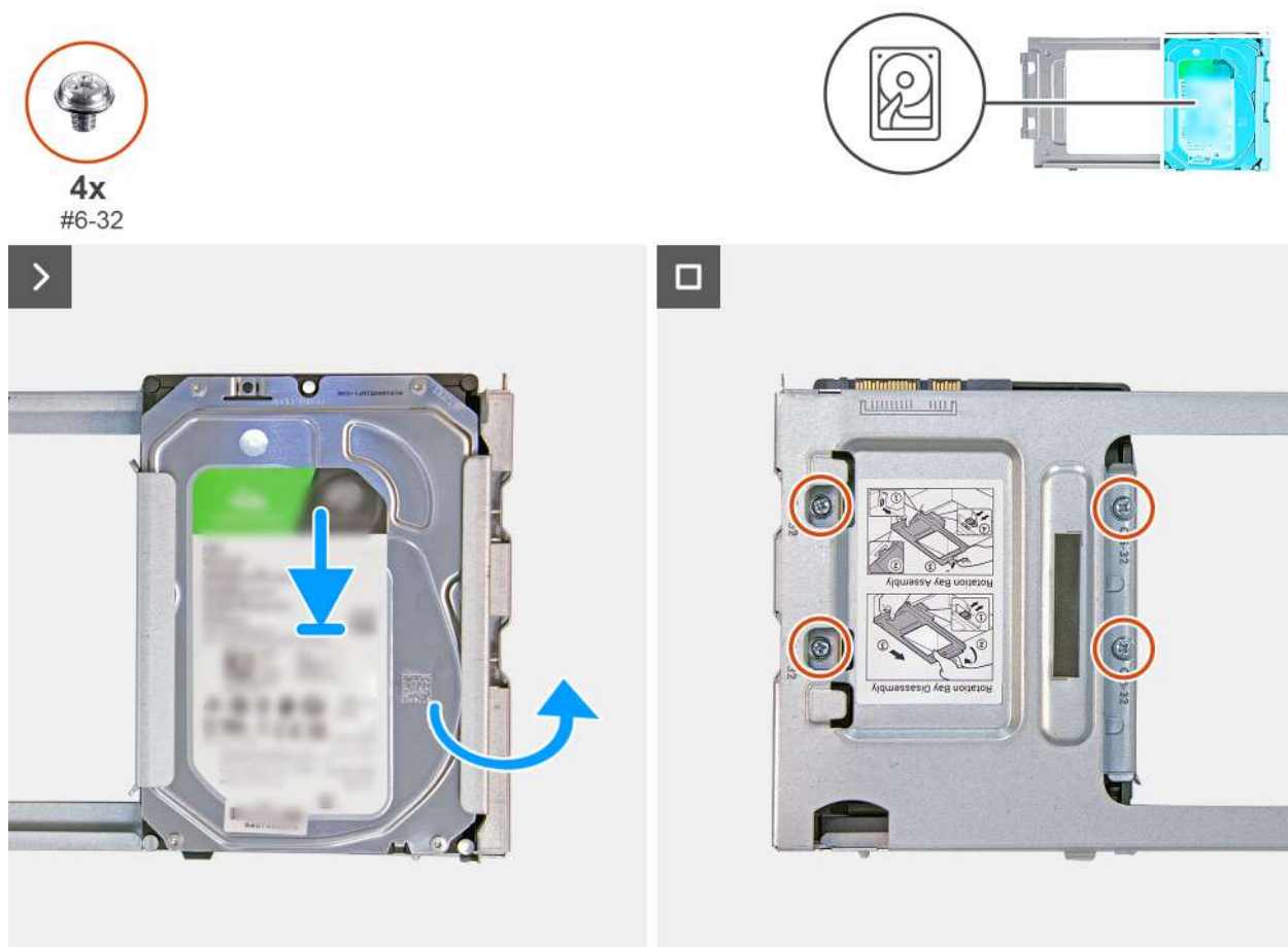
Obrázek 22. Montáž pevného disku
