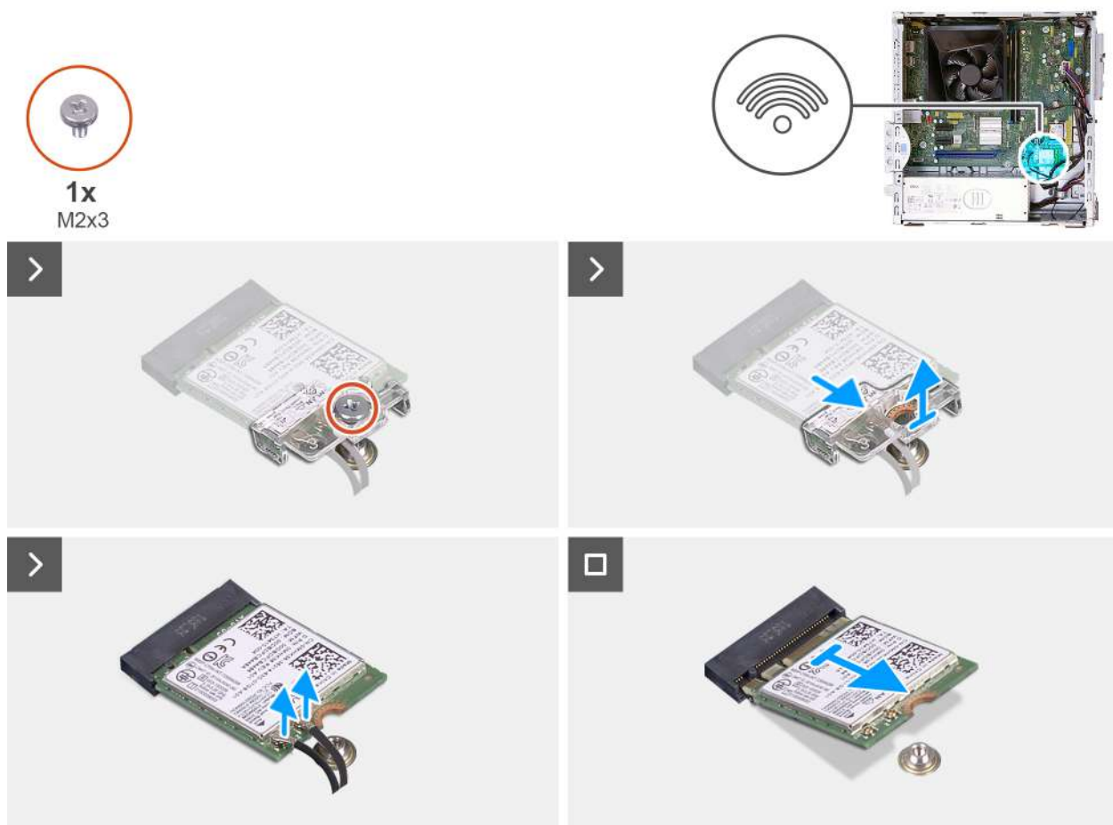
Obrázek 27. Demontáž bezdrátové karty
