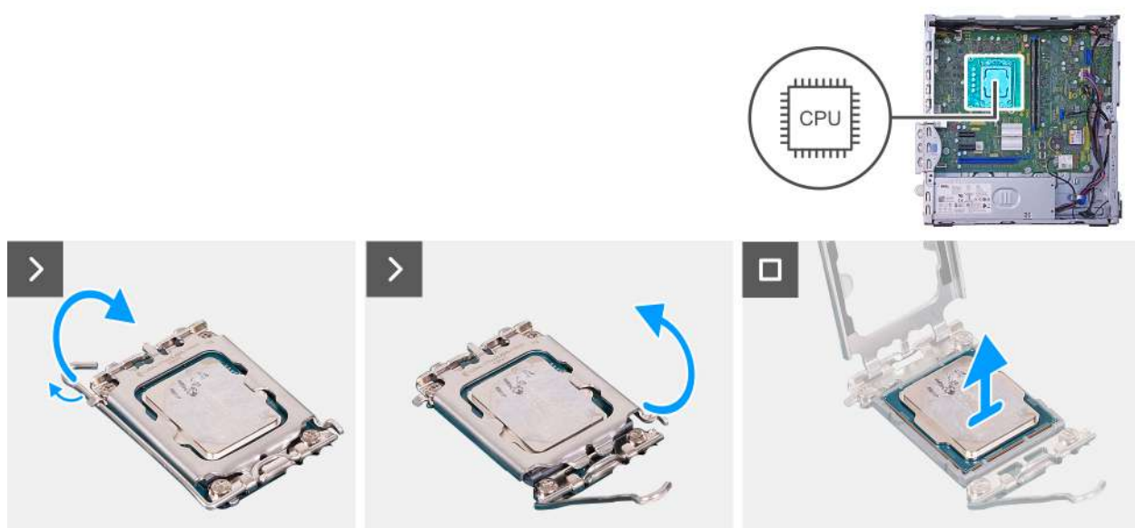
Obrázek 41. Demontáž procesoru
