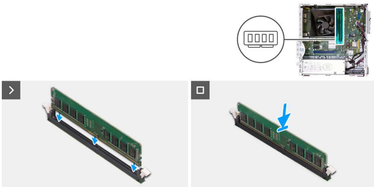
Obrázek 24. Vložení paměťového modulu
