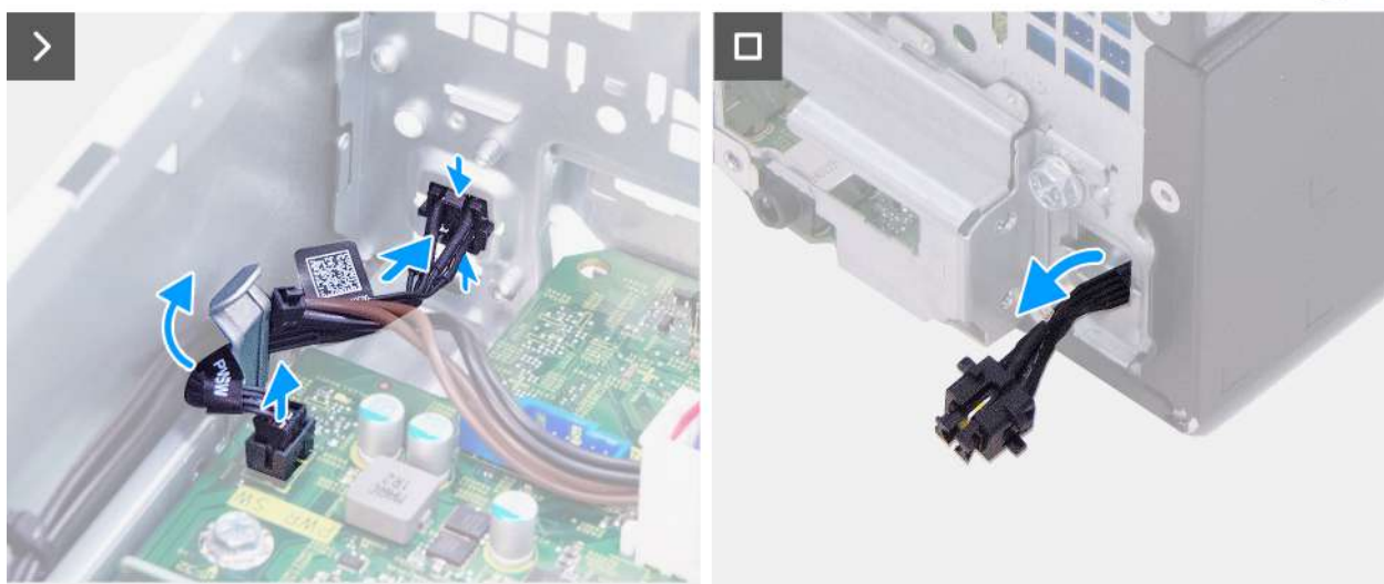
Obrázek 43. Demontáž vypínače
