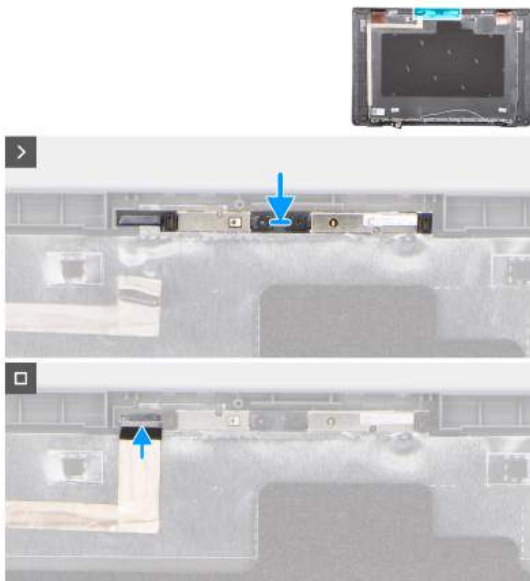
Obrázek 67. Montáž kamery
