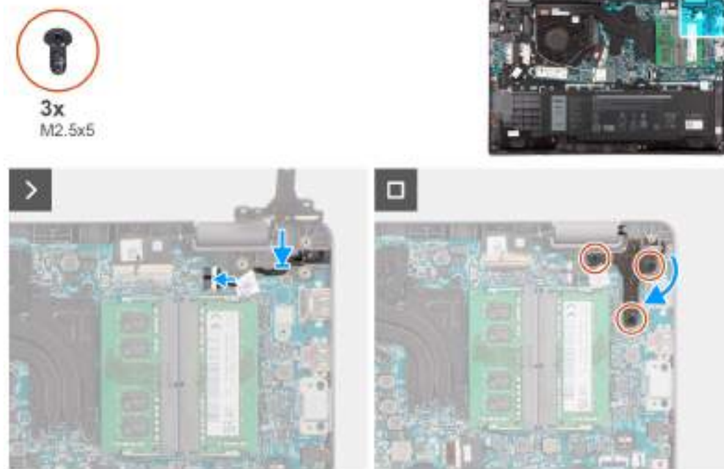
Obrázek 28. Montáž portu napájecího adaptéru
