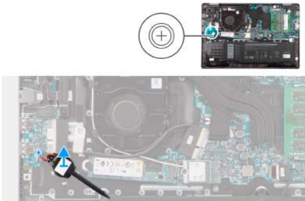
Obrázek 18. Vyjmutí knoflíkové baterie
