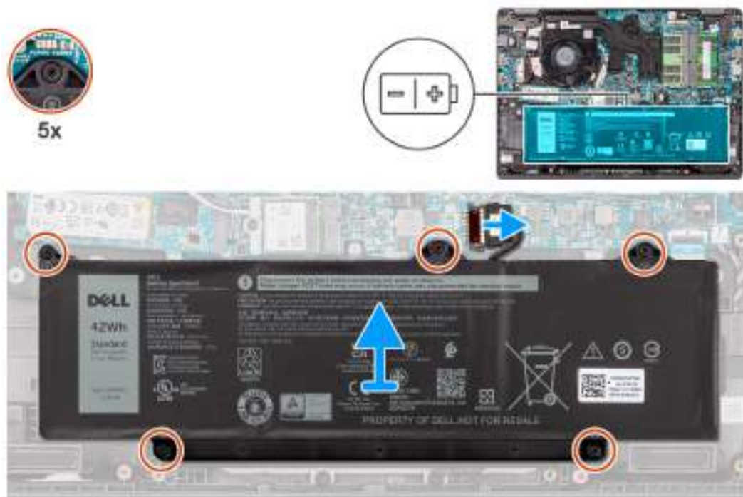
Obrázek 24. Vyjmutí baterie
