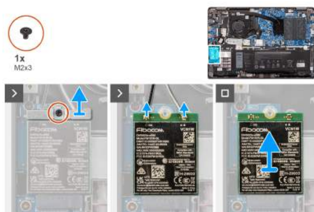
Obrázek 16. Vyjmutí karty sítě WWAN
