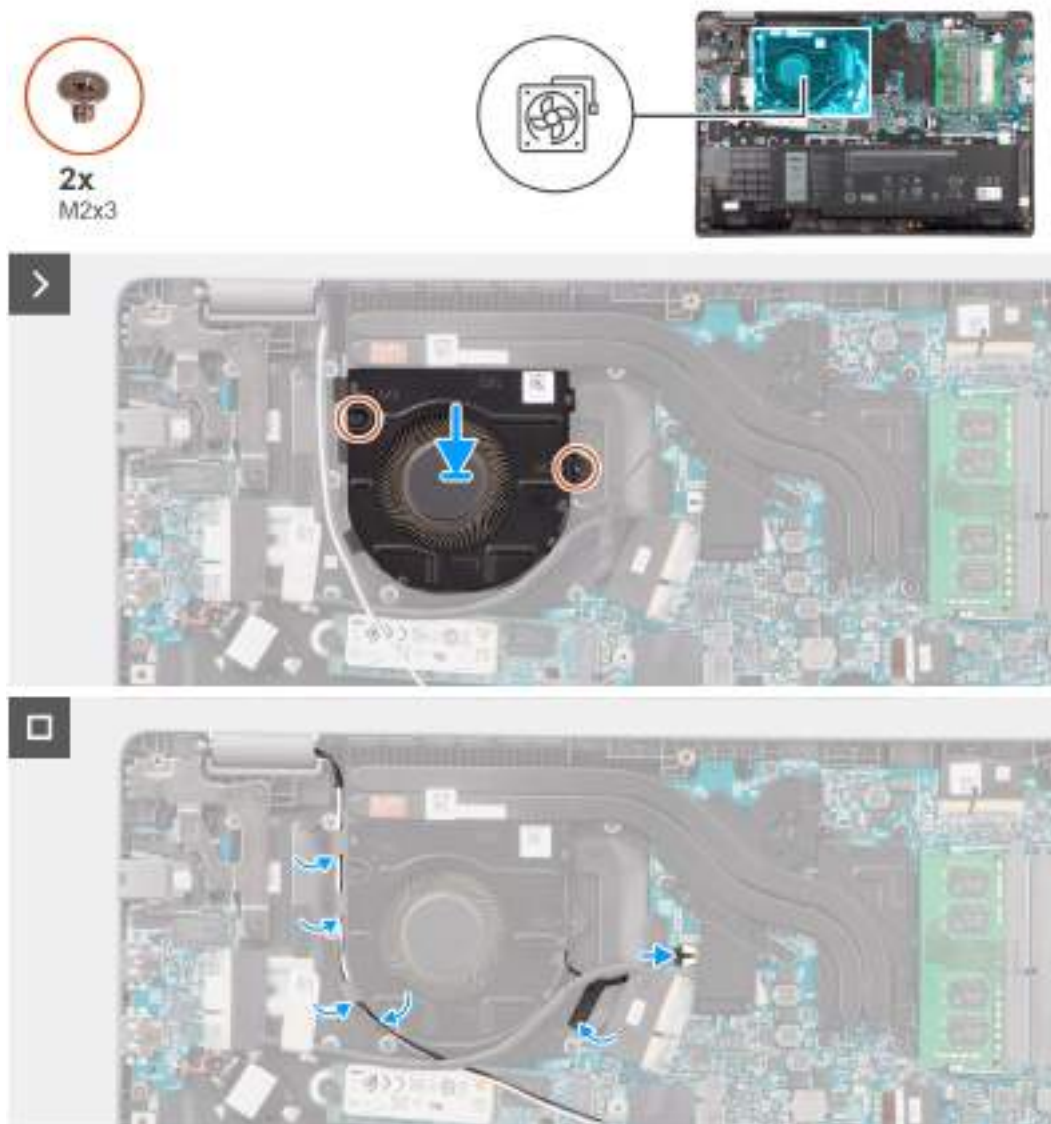
Obrázek 34. Montáž ventilátoru
