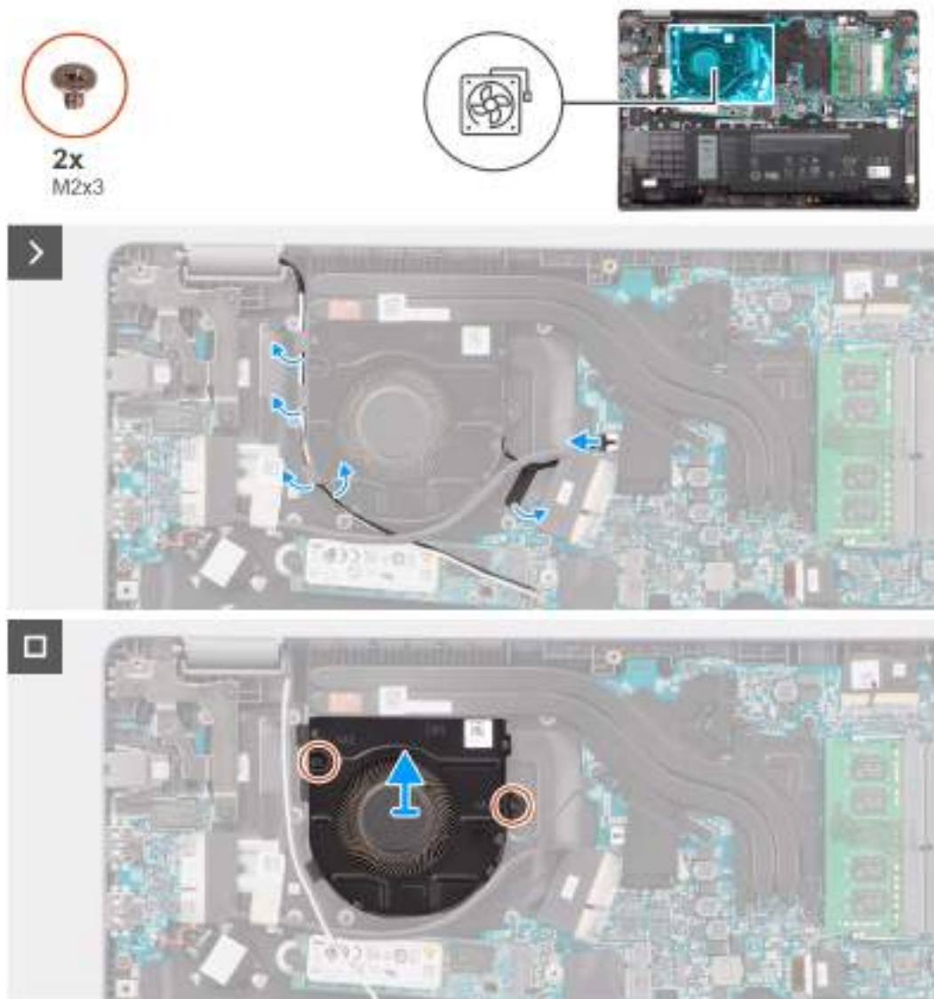
Obrázek 33. Demontáž ventilátoru
