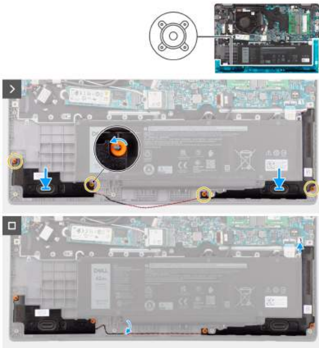
Obrázek 21. Montáž reproduktorů
