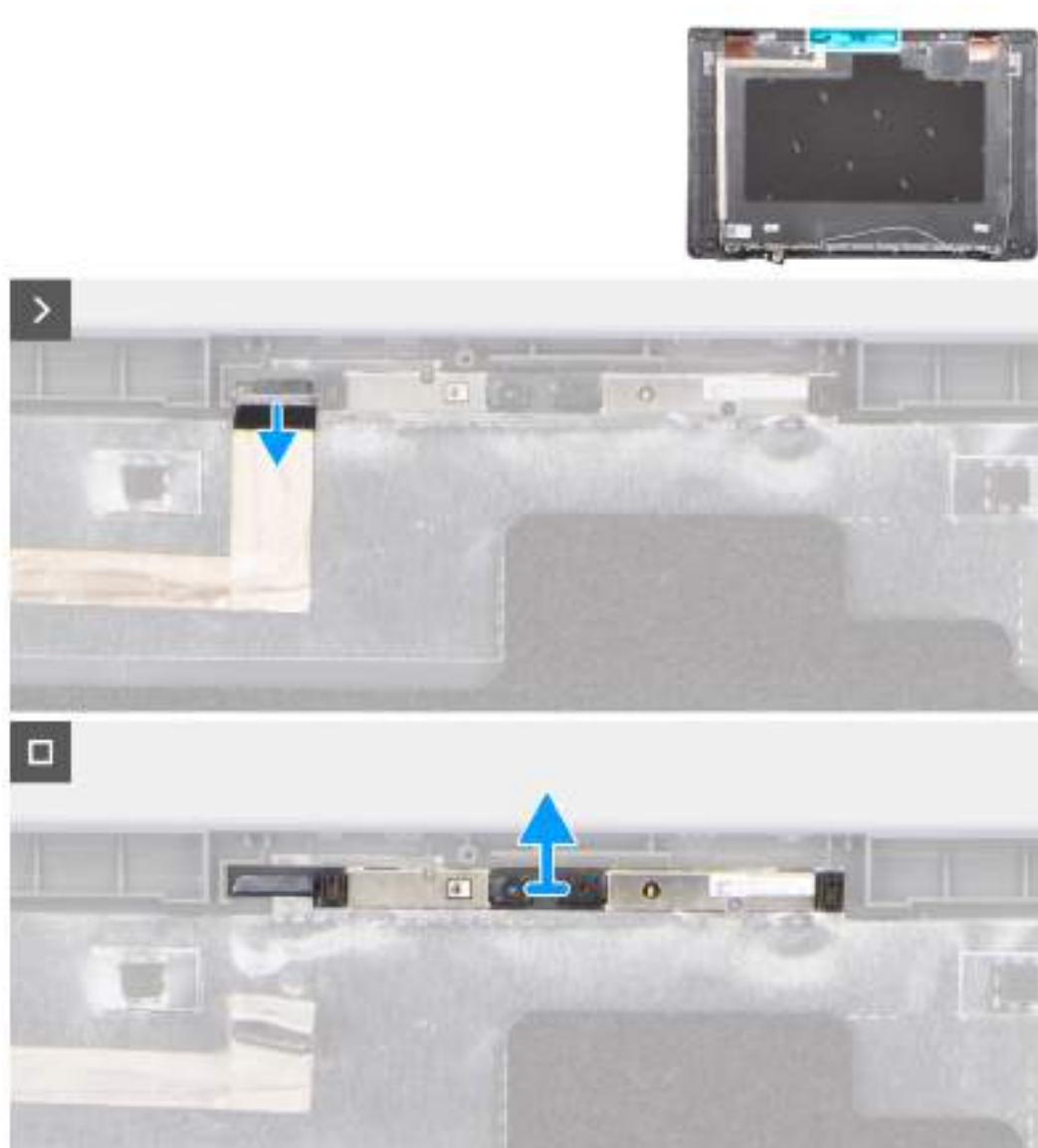
Obrázek 66. Demontáž kamery
