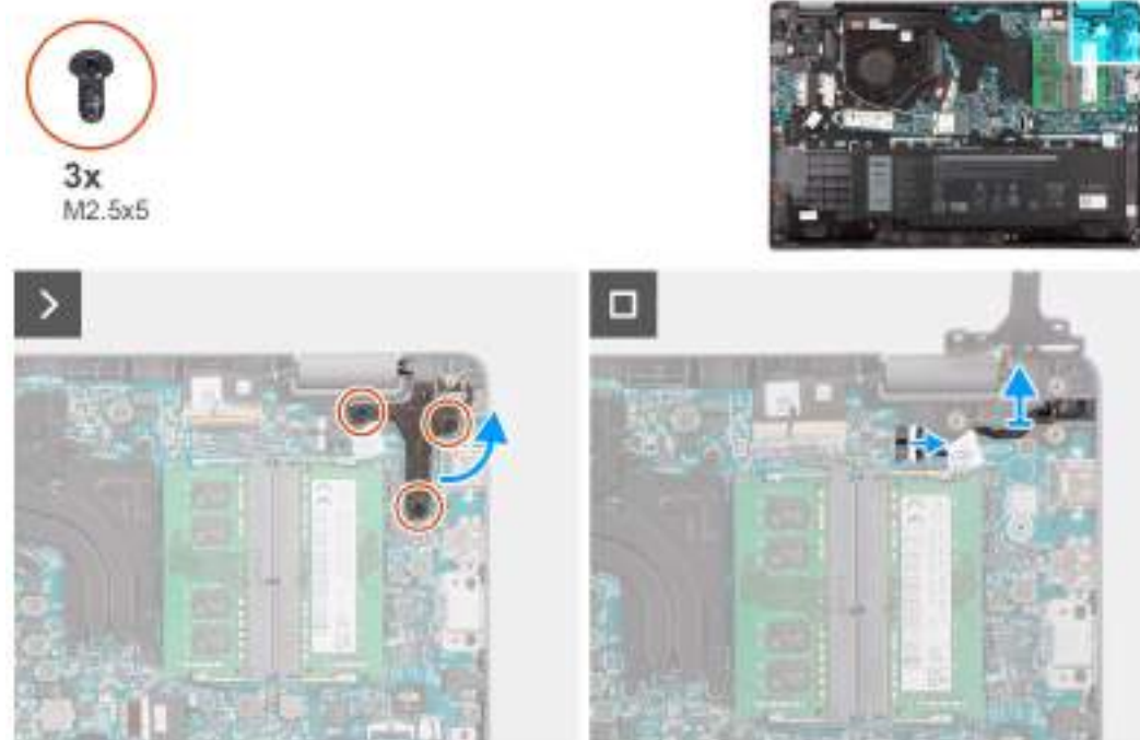
Obrázek 27. Demontáž portu napájecího adaptéru
