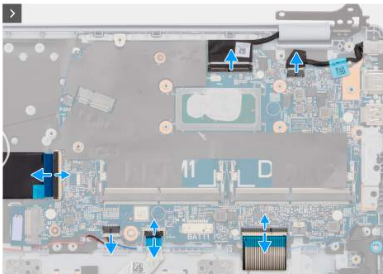
Obrázek 95. Demontáž konektorů kabelů
