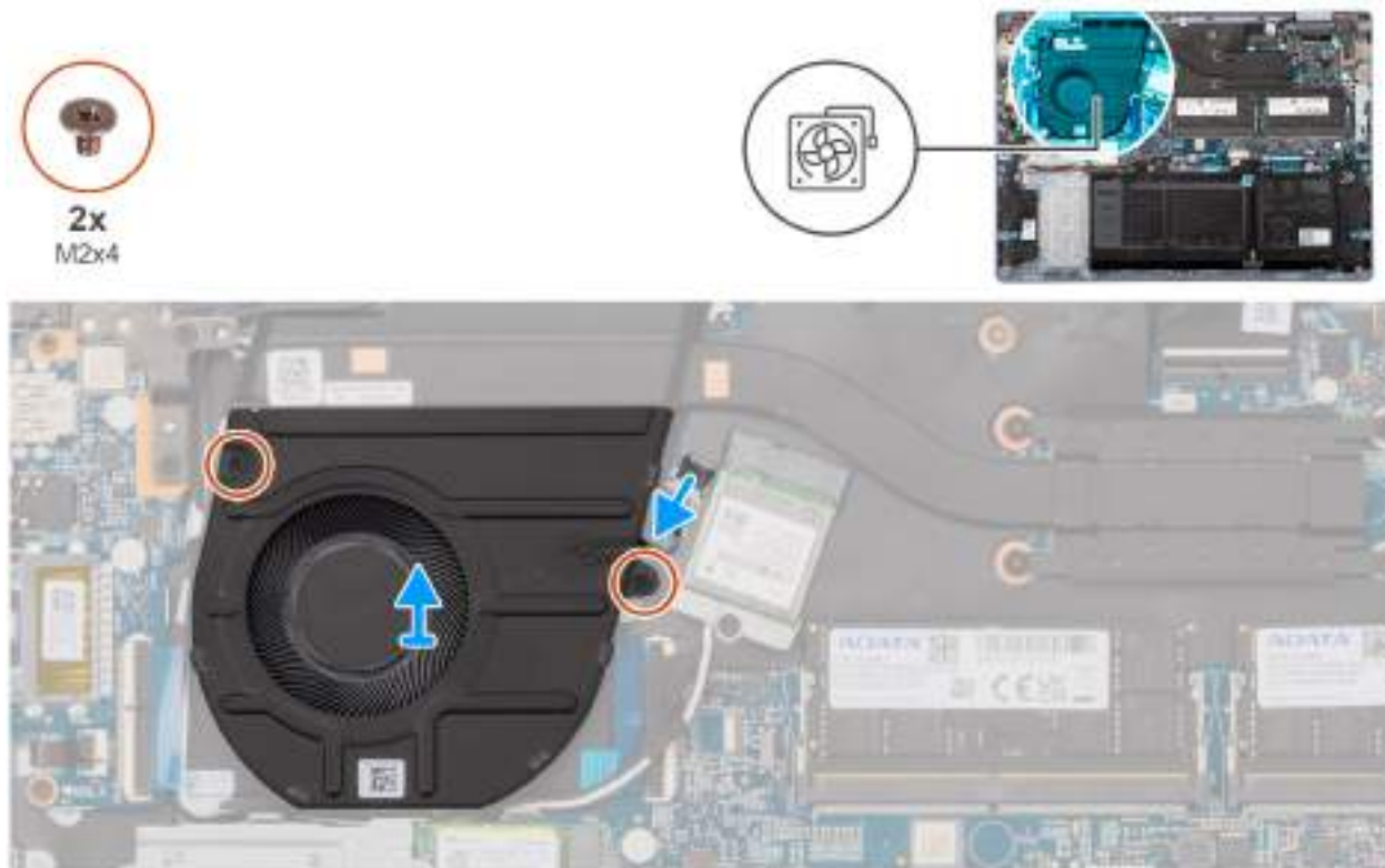
Obrázek 32. Demontáž ventilátoru
