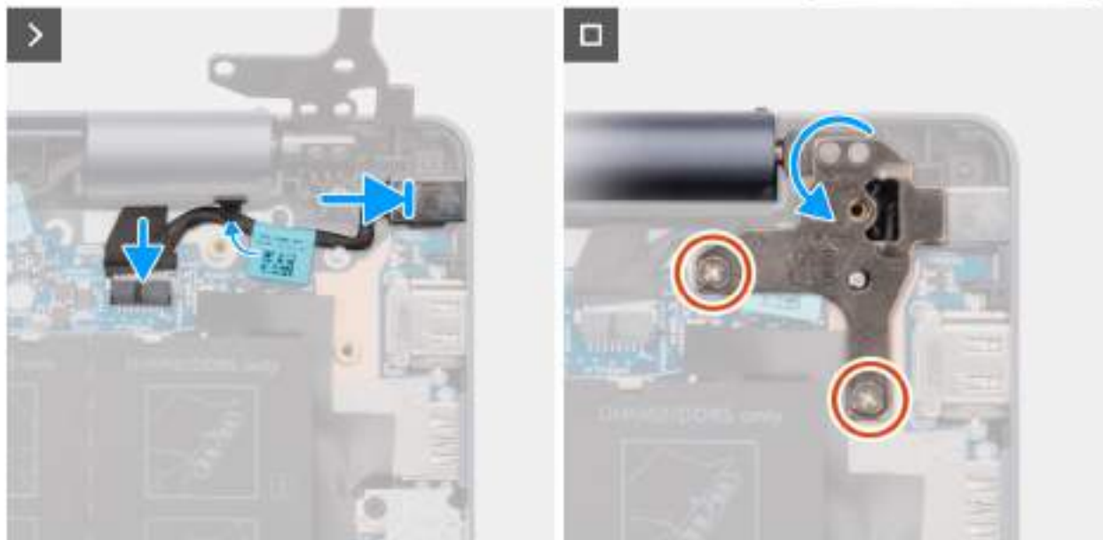
Obrázek 51. Montáž portu napájecího adaptéru
