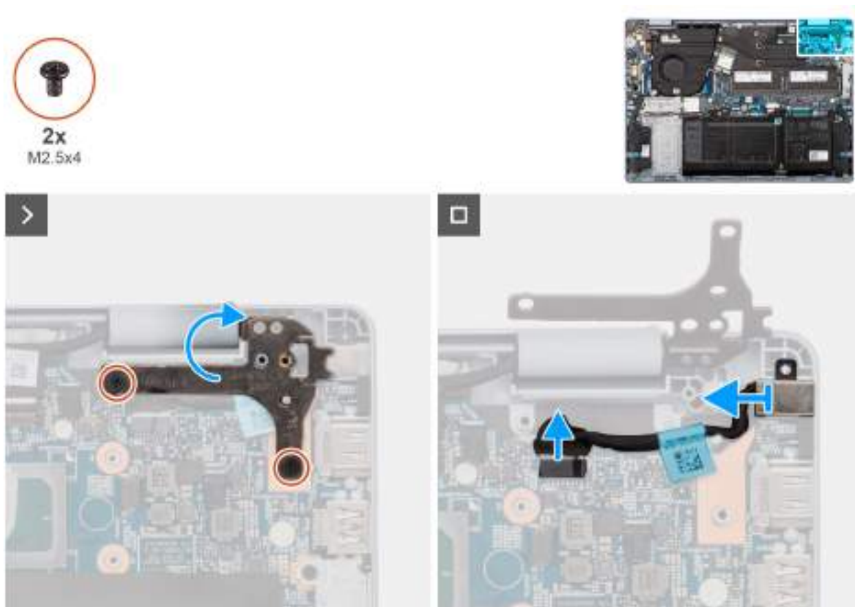
Obrázek 48. Vyjmutí portu napájecího adaptéru
