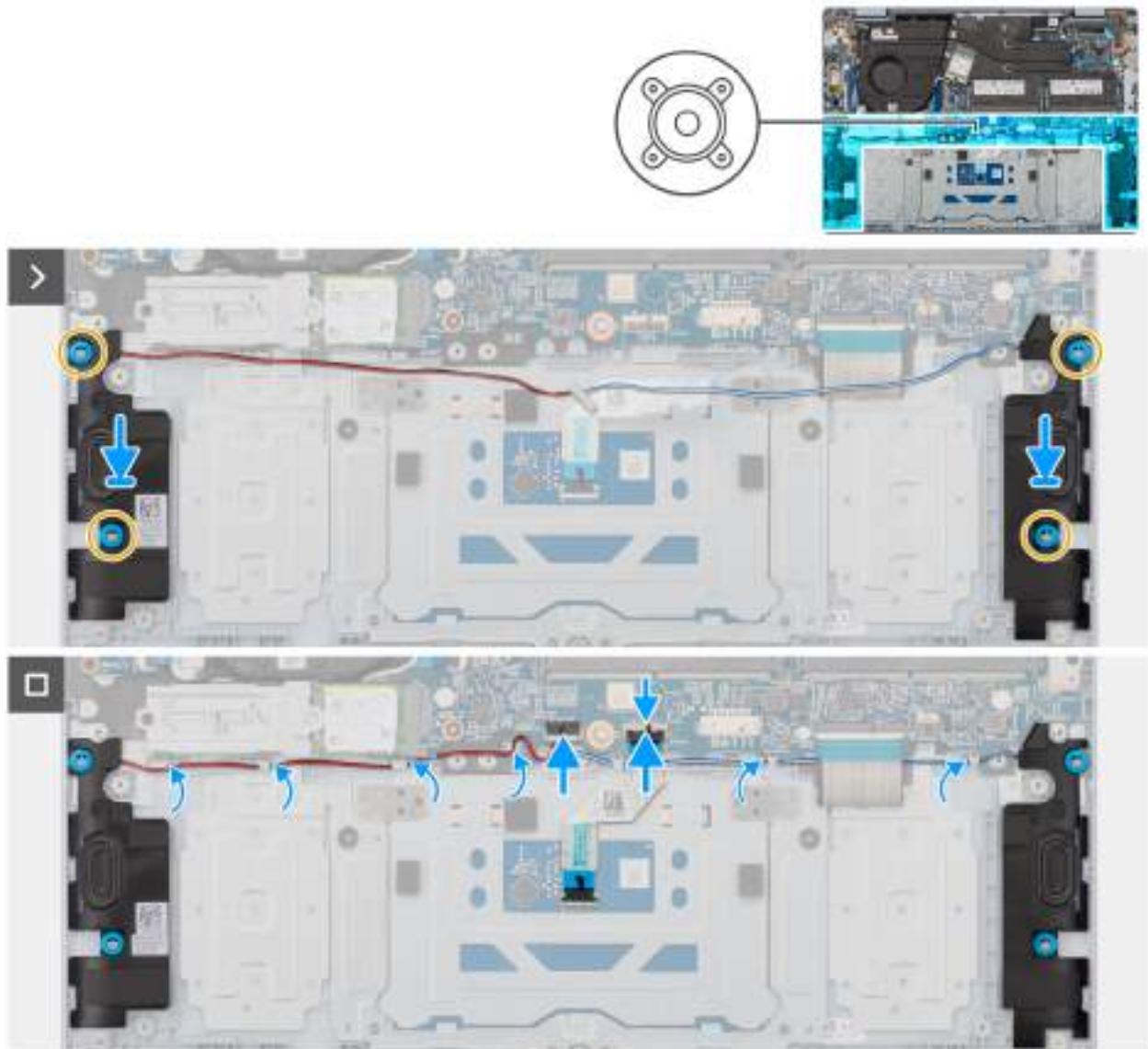
Obrázek 65. Montáž reproduktorů
