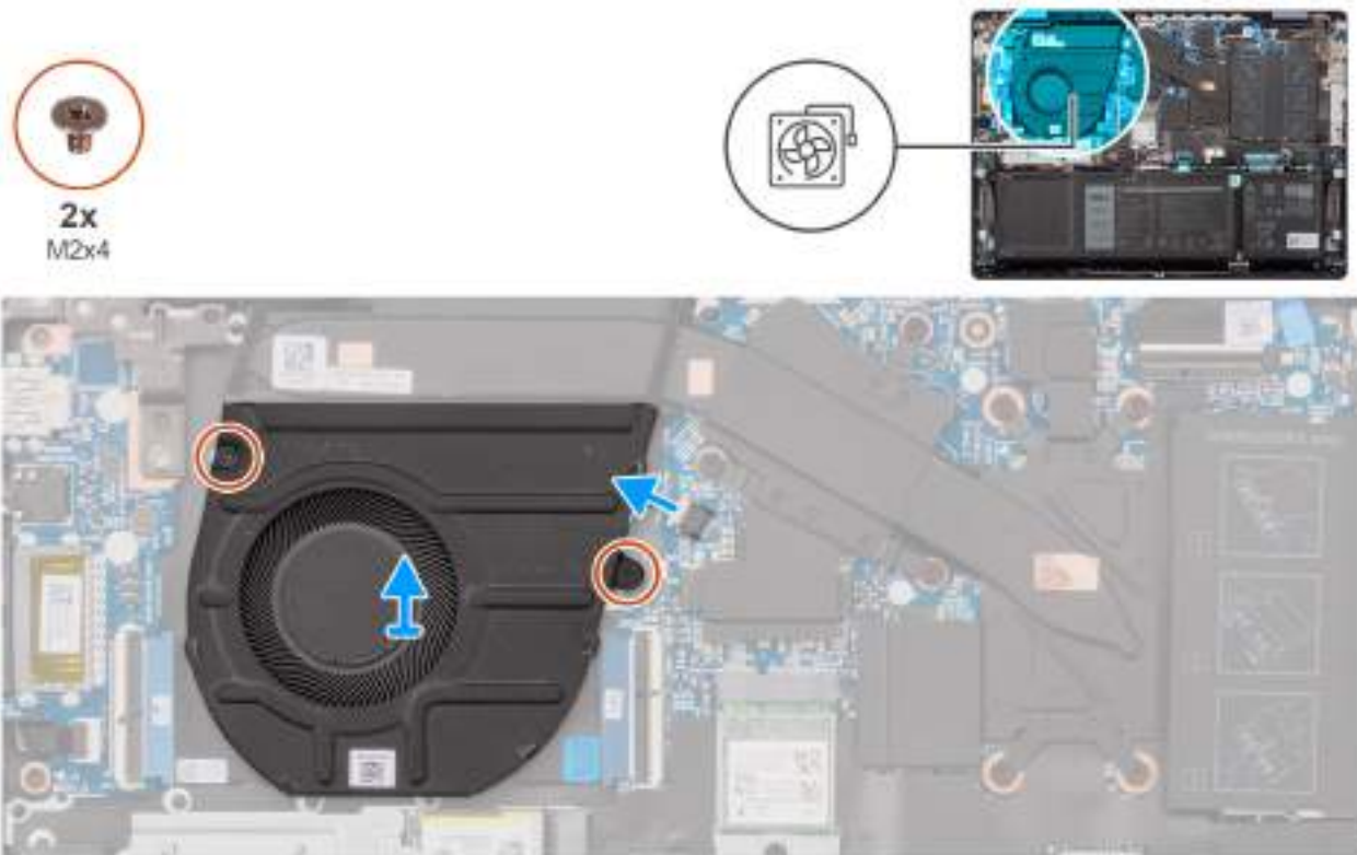
Obrázek 34. Demontáž ventilátoru
