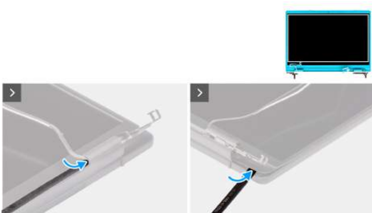
Obrázek 76. Demontáž čelního krytu displeje
