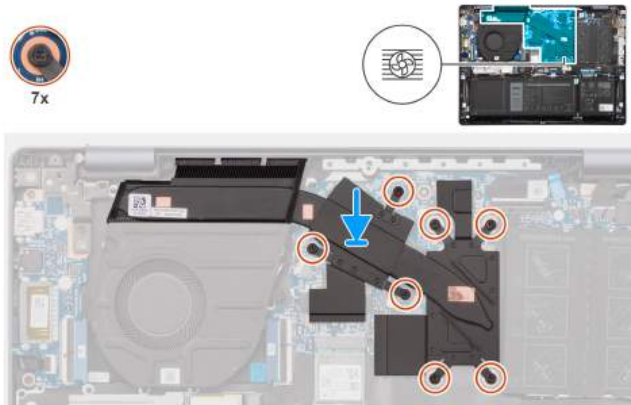
Obrázek 47. Montáž chladiče
