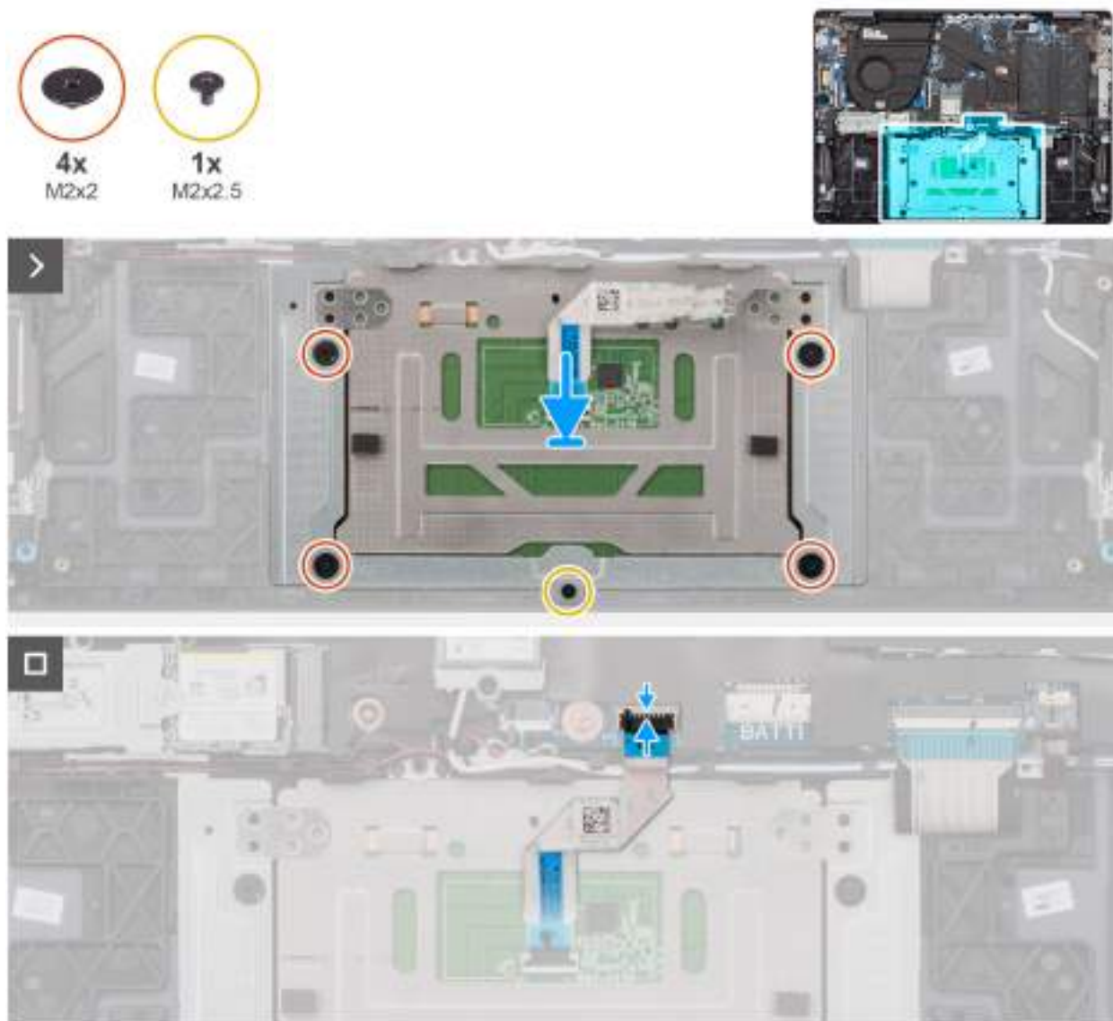
Obrázek 63. Montáž dotykové podložky
