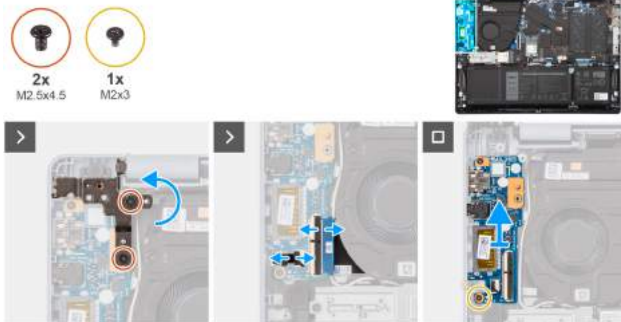
Obrázek 54. Demontáž desky I/O
