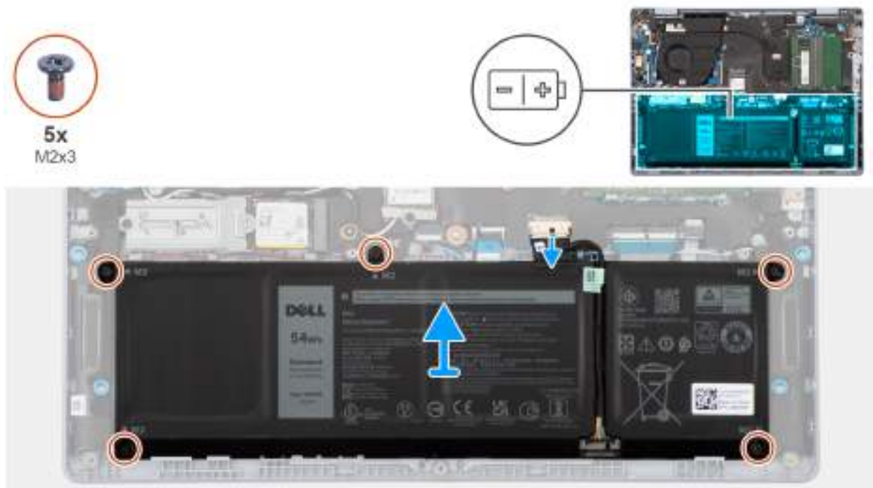
Obrázek 38. Vymutí baterie
