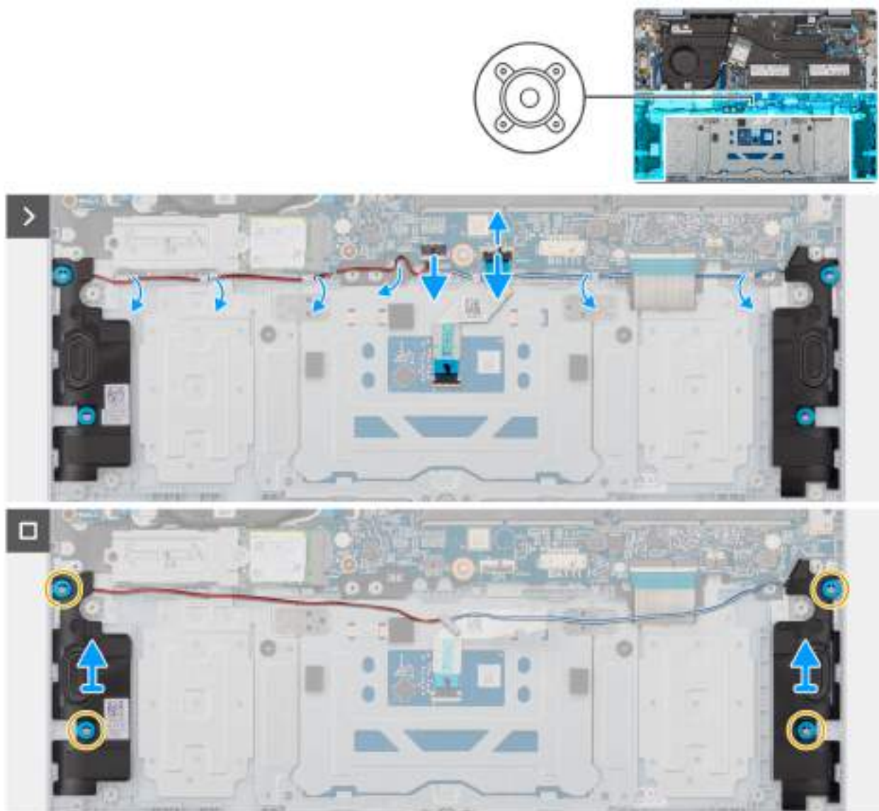
Obrázek 64. Demontáž reproduktorů
