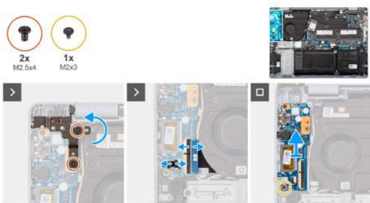
Obrázek 52. Demontáž desky I/O
