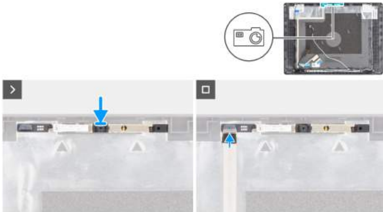
Obrázek 90. Montáž kamery
