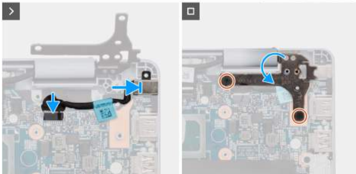
Obrázek 49. Montáž portu napájecího adaptéru
