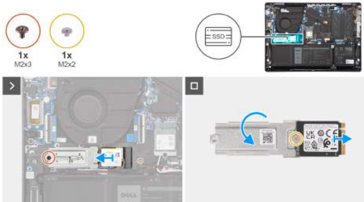
Obrázek 26. Demontáž disku SSD
