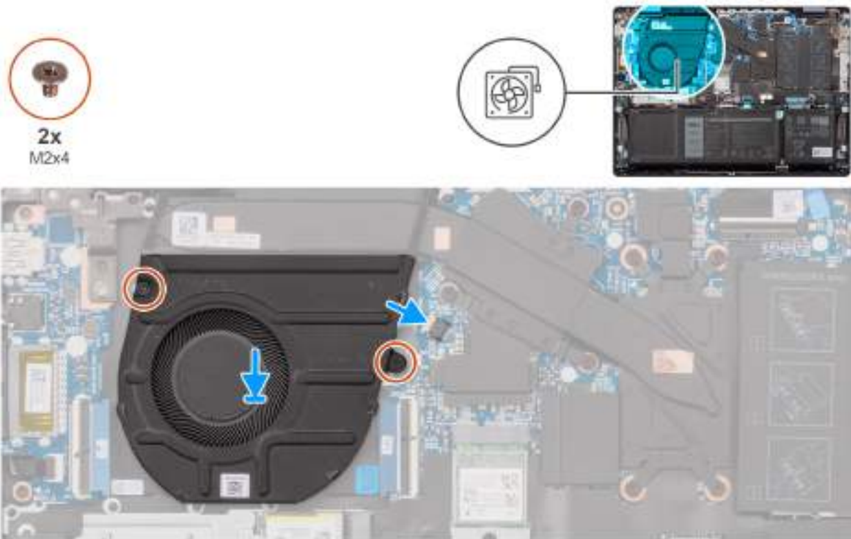
Obrázek 35. Montáž ventilátoru
