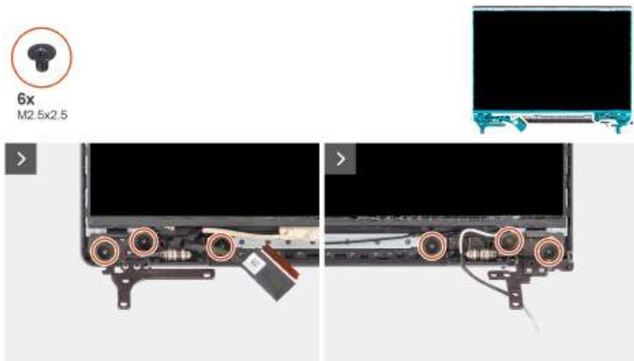
Obrázek 78. Demontáž šroubů obrazovky displeje
