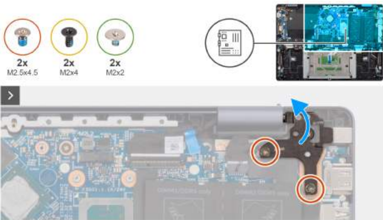
Obrázek 103. Demontáž šroubů pantů
