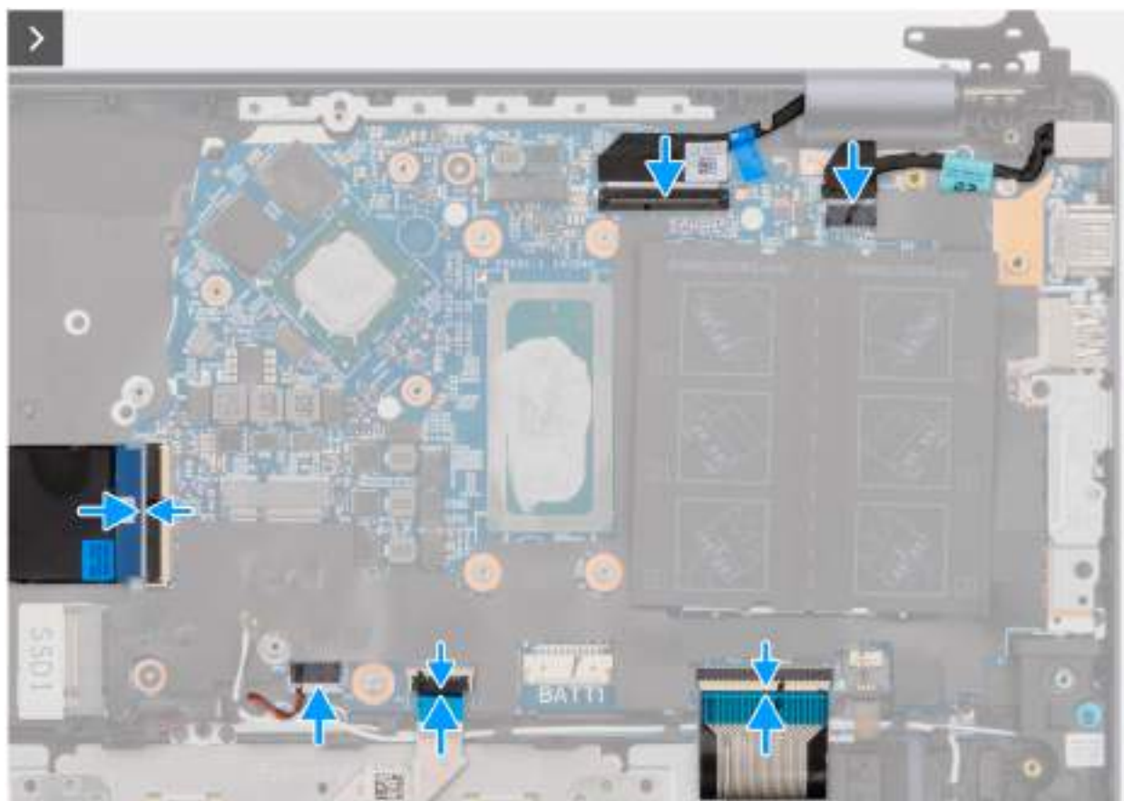
Obrázek 109. Montáž konektorů kabelů
