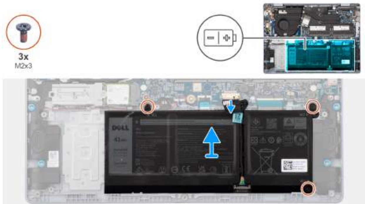
Obrázek 36. Vyjmutí baterie
