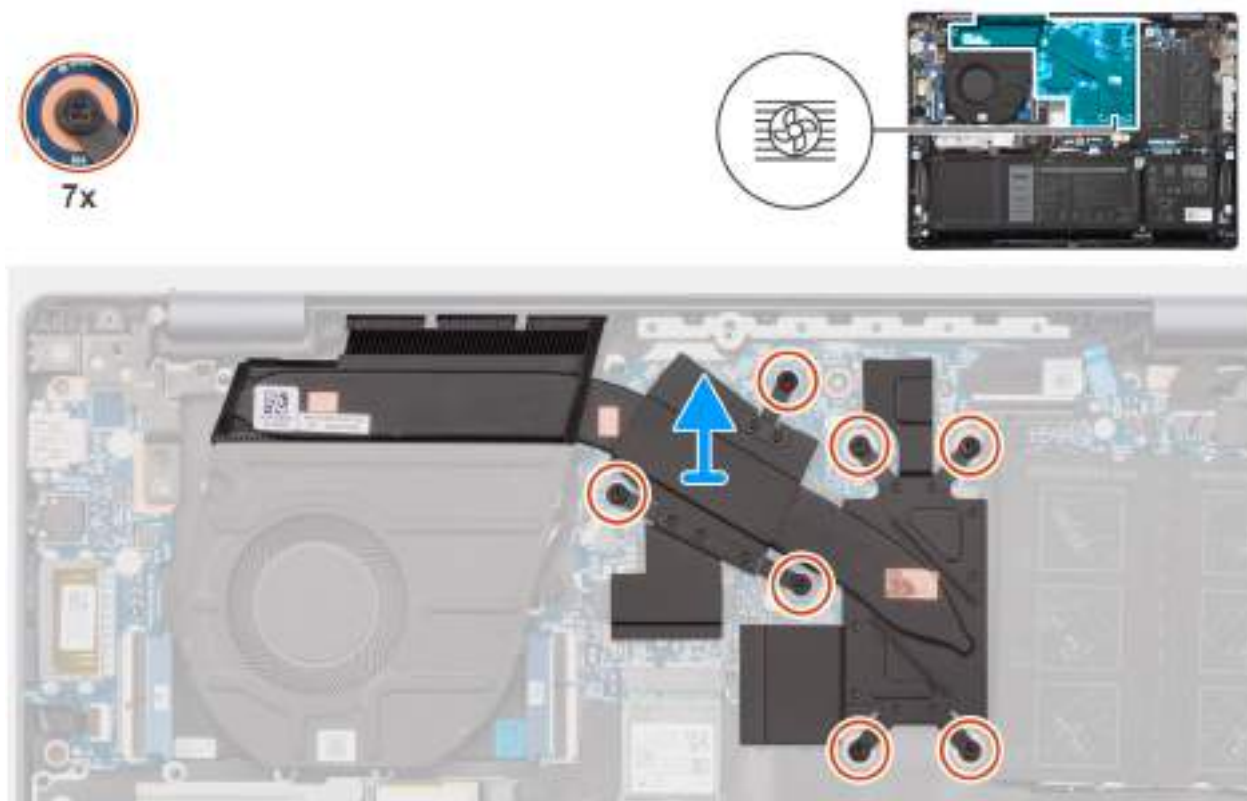
Obrázek 46. Demontáž chladiče
