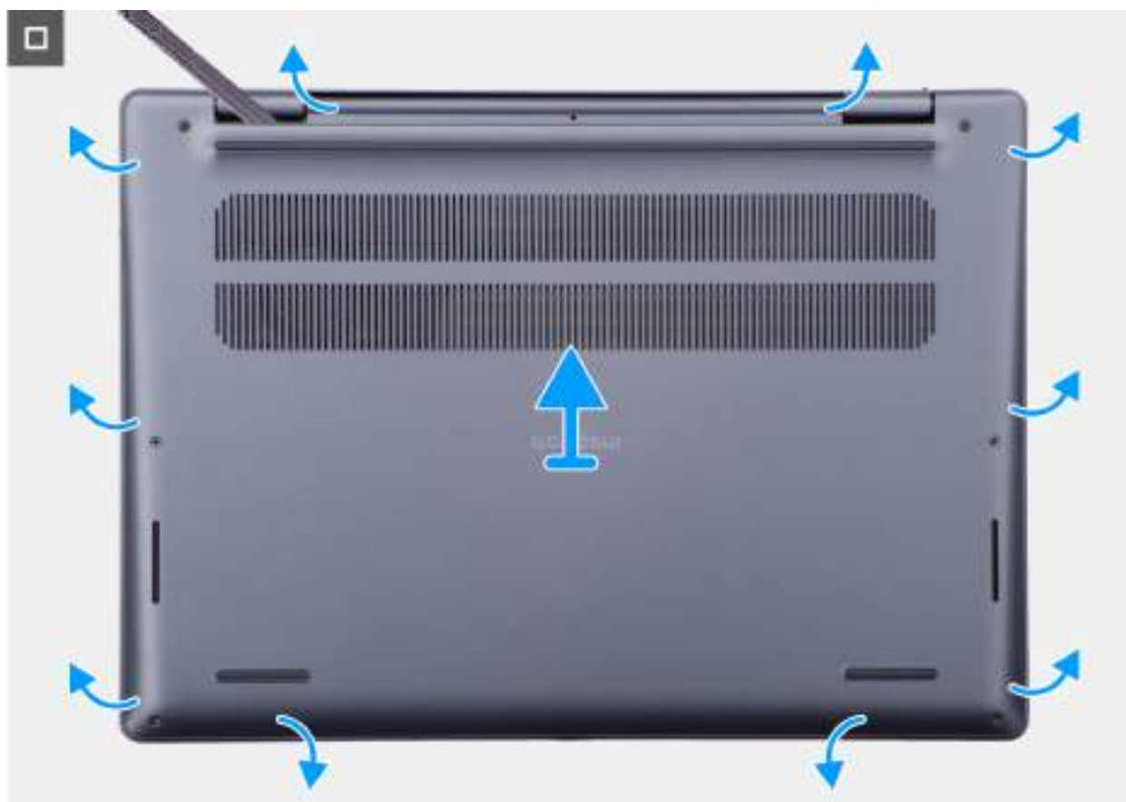
Obrázek 16. Sejmutí spodního krytu
