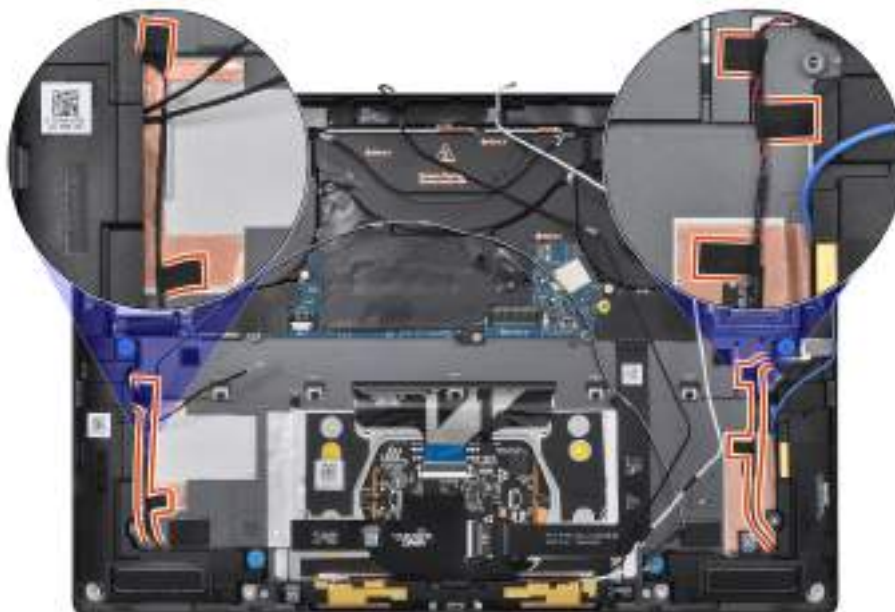
Obrázek 67. Nálepka kabelu reproduktoru
