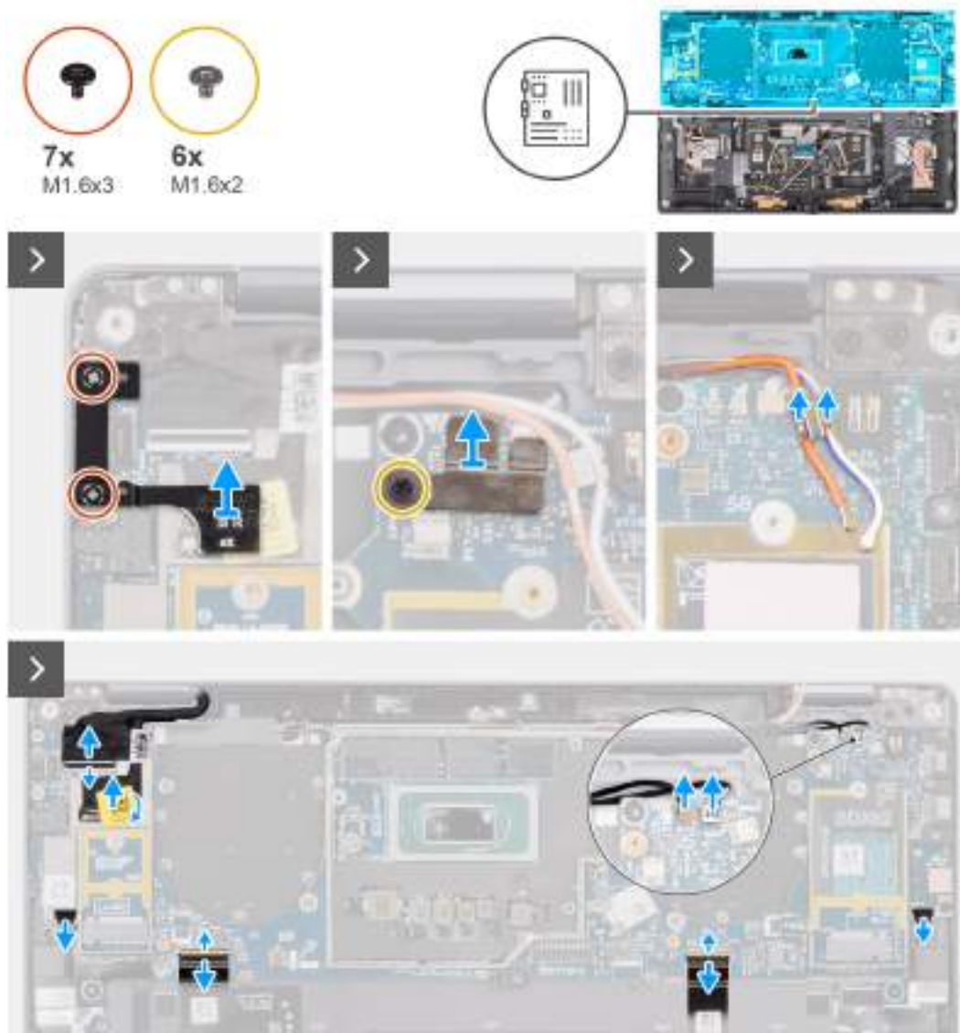
Obrázek 51. Demontáž základní desky
