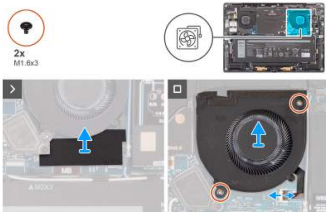
Obrázek 26. Demontáž levého ventilátoru
