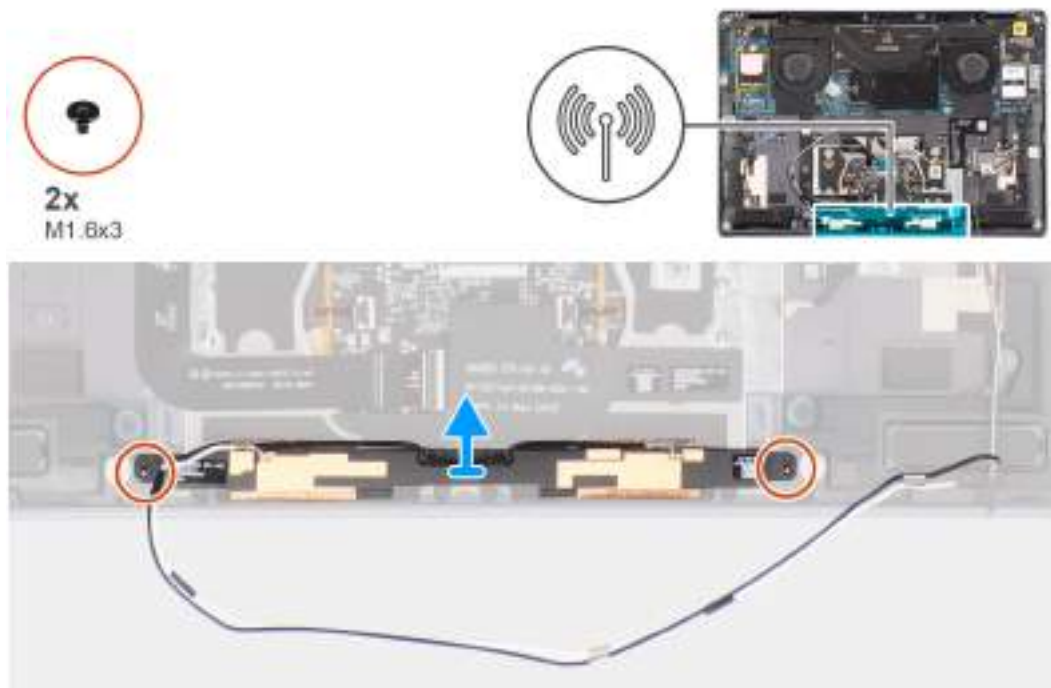
Obrázek 35. Demontáž anténního modulu WLAN
