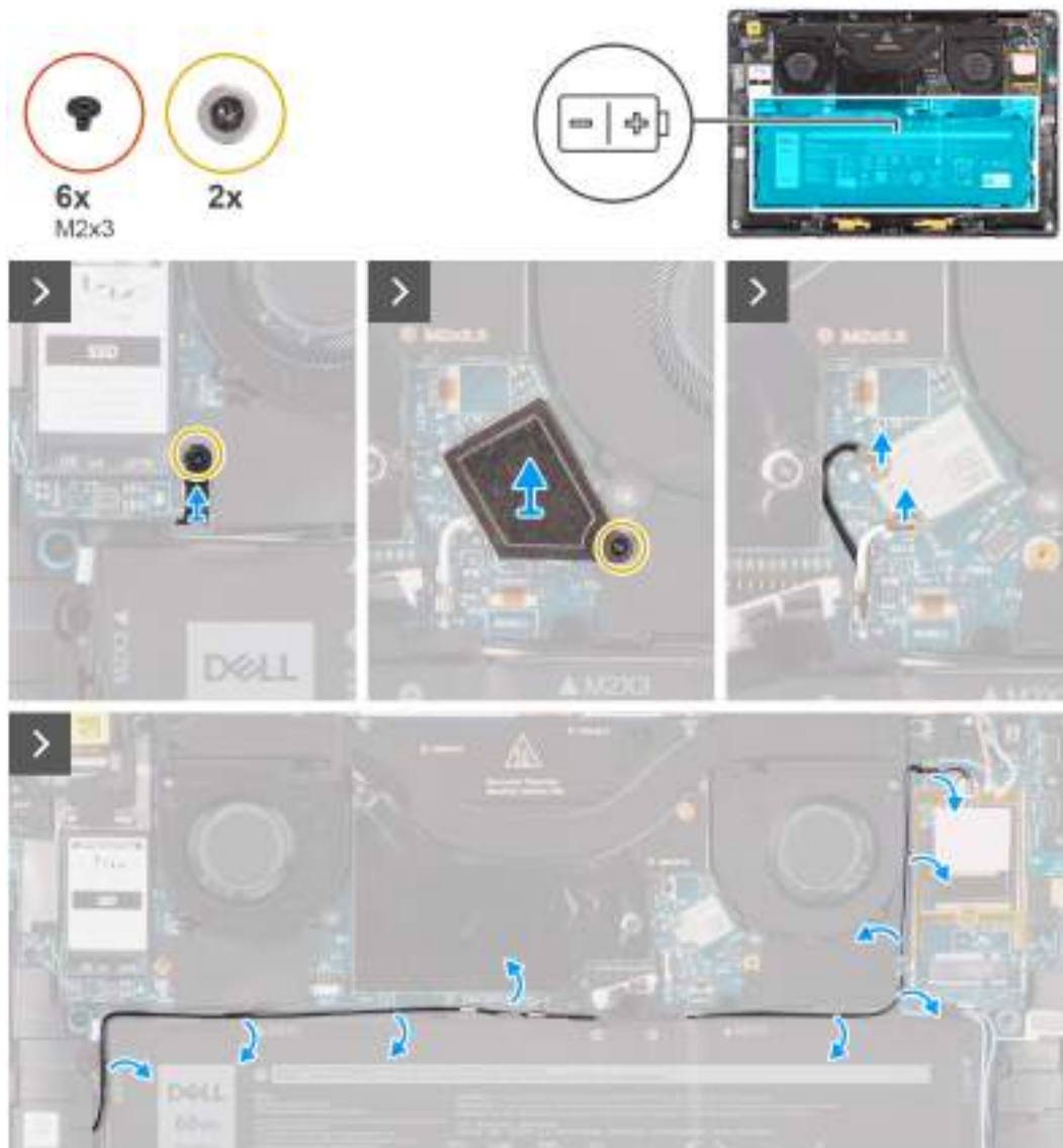
Obrázek 37. Vyjmutí baterie
