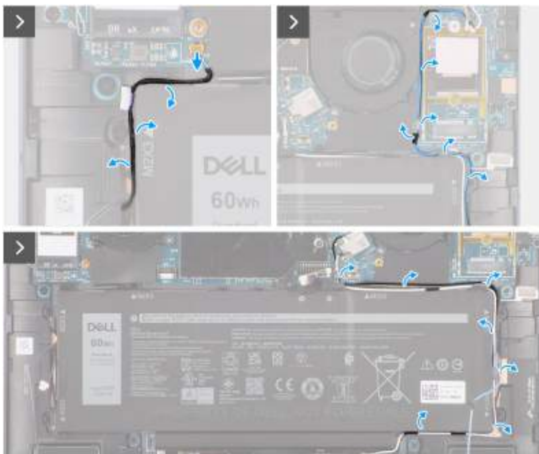
Obrázek 38. Vyjmutí baterie
