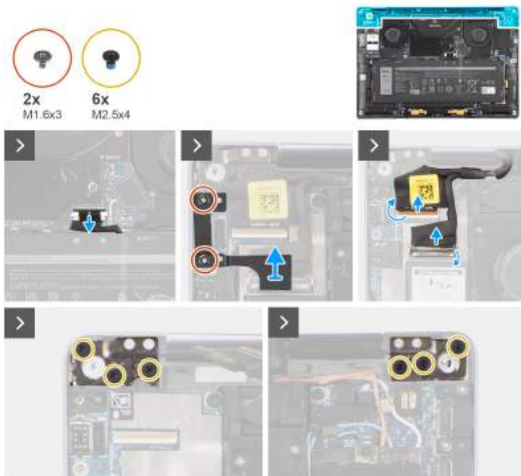
Obrázek 45. Demontáž sestavy displeje
