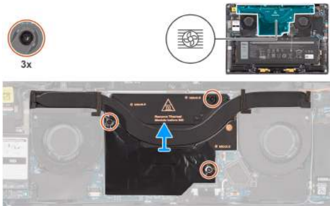
Obrázek 43. Demontáž chladiče
