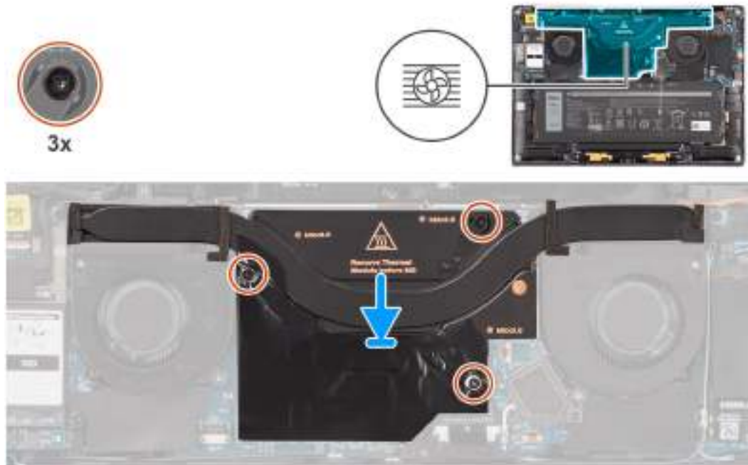
Obrázek 44. Montáž chladiče
