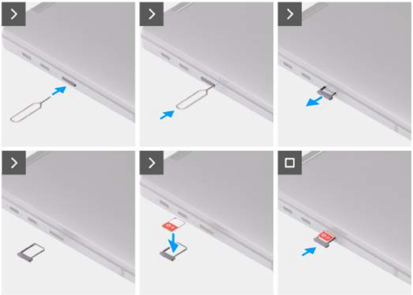
Obrázek 17. Demontáž přihrádky na kartu nano-SIM
