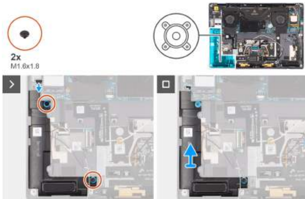
Obrázek 65. Demontáž pravého reproduktoru
