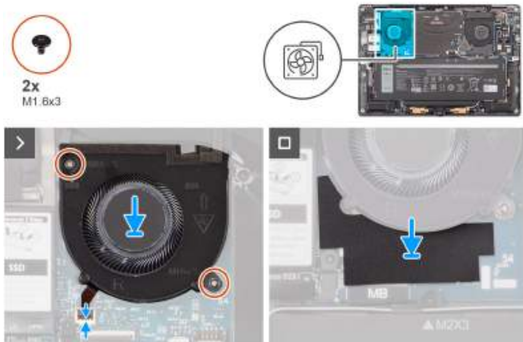
Obrázek 25. Montáž pravého ventilátoru
