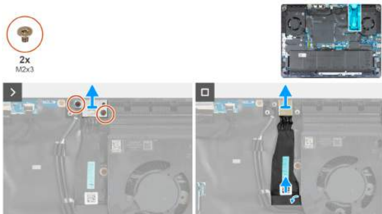
Obrázek 37. Demontáž portu napájecího adaptéru
