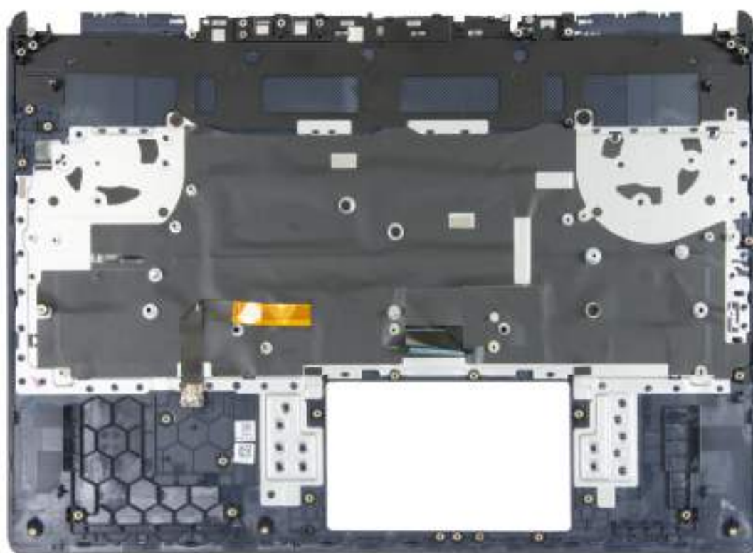
Obrázek 79. Montáž sestavy opěrky pro dlaň a klávesnice
