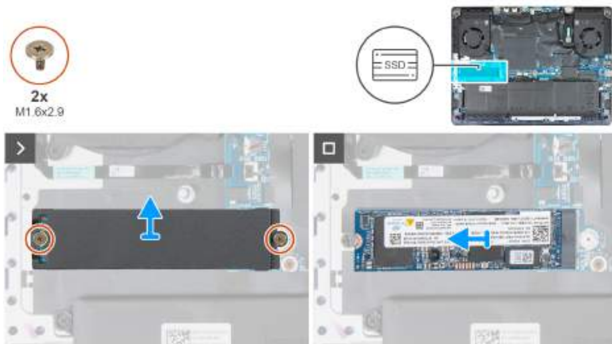
Obrázek 29. Demontáž disku SSD M.2 2280 ze slotu SSD2
