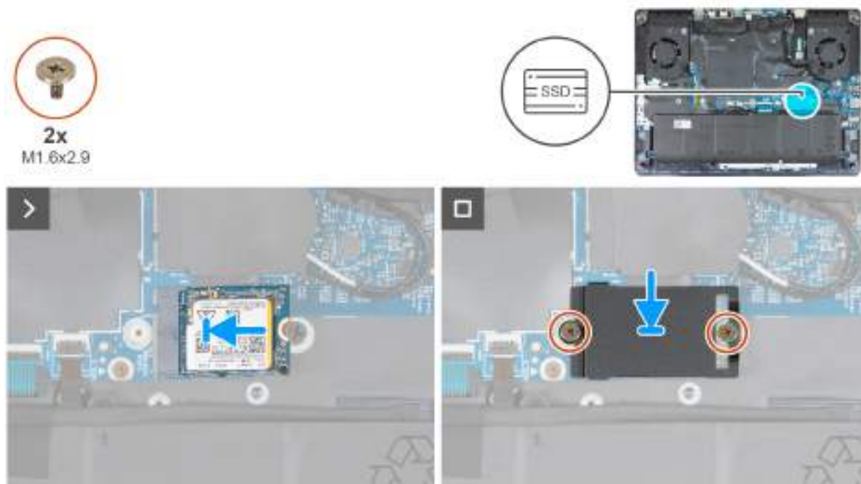
Obrázek 24. Montáž disku SSD M.2 2230 do slotu SSD1
