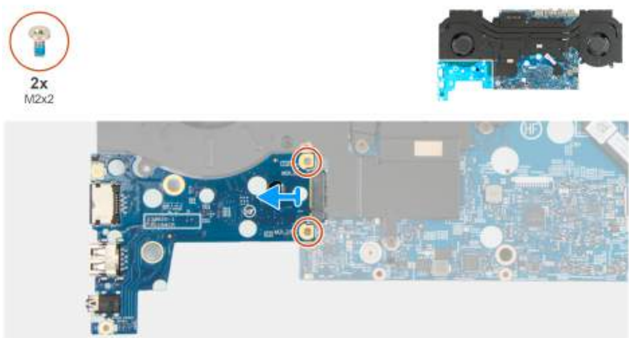
Obrázek 51. Demontáž desky I/O
