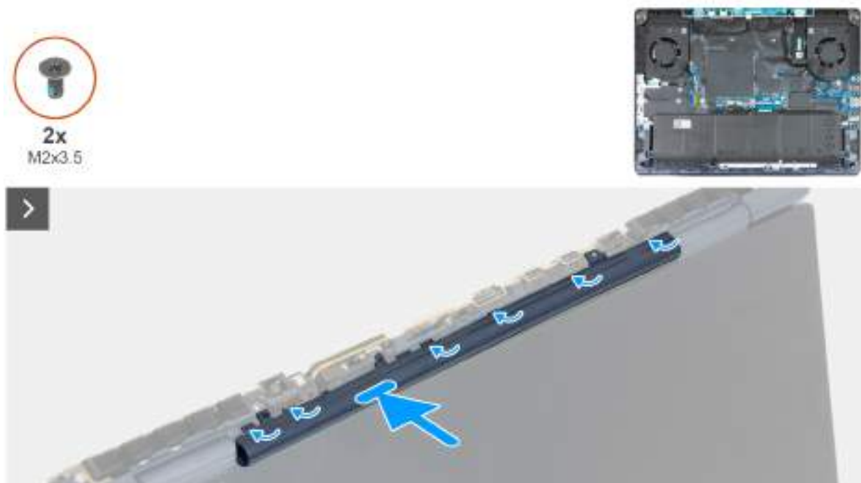
Obrázek 69. Montáž středové lišty
