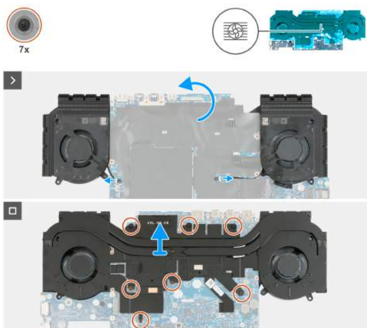
Obrázek 50. Demontáž sestavy základní desky
