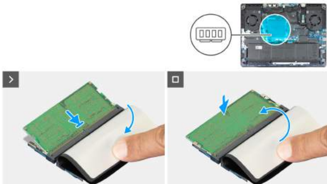
Obrázek 22. Vložení paměťového modulu
