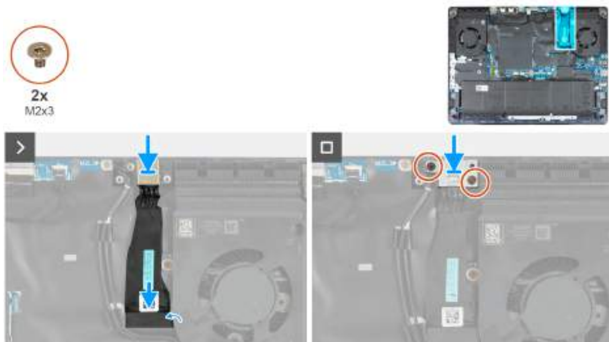
Obrázek 38. Montáž portu napájecího adaptéru
