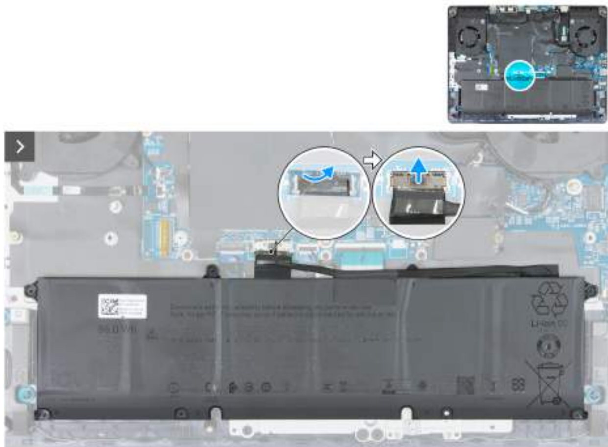
Obrázek 13. Odpojení kabelu baterie
