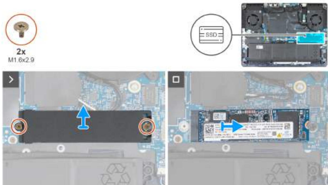
Obrázek 27. Vyjmutí disku SSD M.2 2280 ze slotu SSD1
