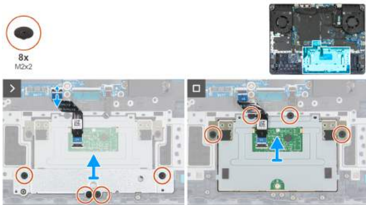
Obrázek 43. Demontáž dotykové podložky
