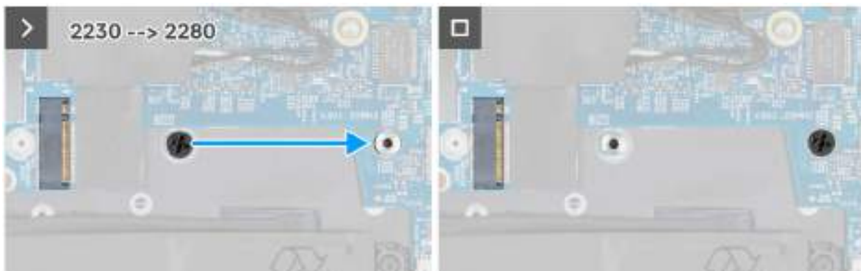
Obrázek 31. Postup přesunutí šroubového držáku pro instalaci M2.2280
