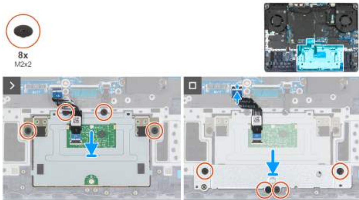
Obrázek 44. Montáž dotykové podložky
