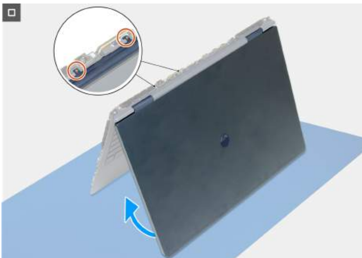
Obrázek 70. Montáž středové lišty
