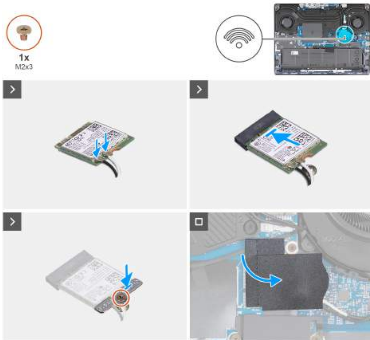
Obrázek 34. Montáž bezdrátové karty
