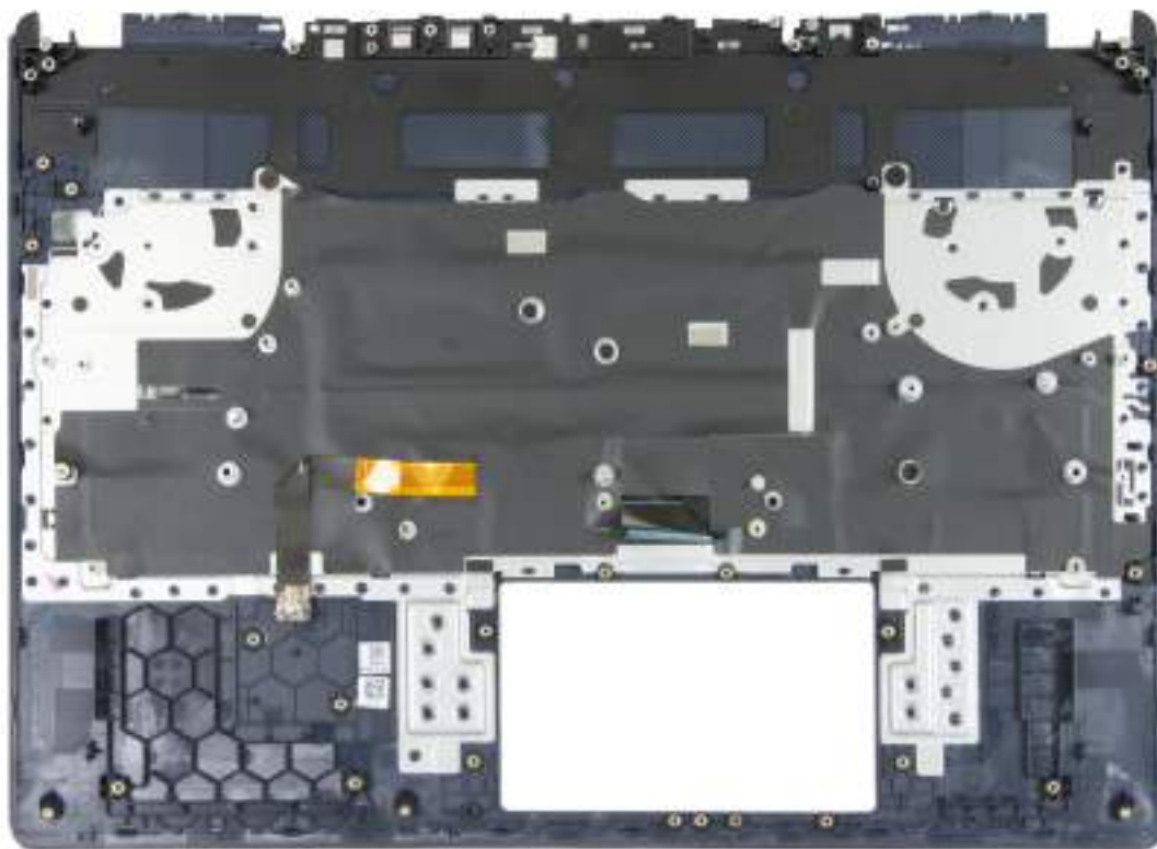
Obrázek 76. Demontáž sestavy opěrky pro dlaň a klávesnice
