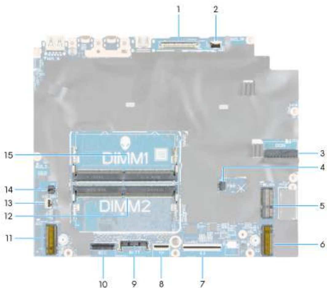
Obrázek 52. Konektory na základní desce
