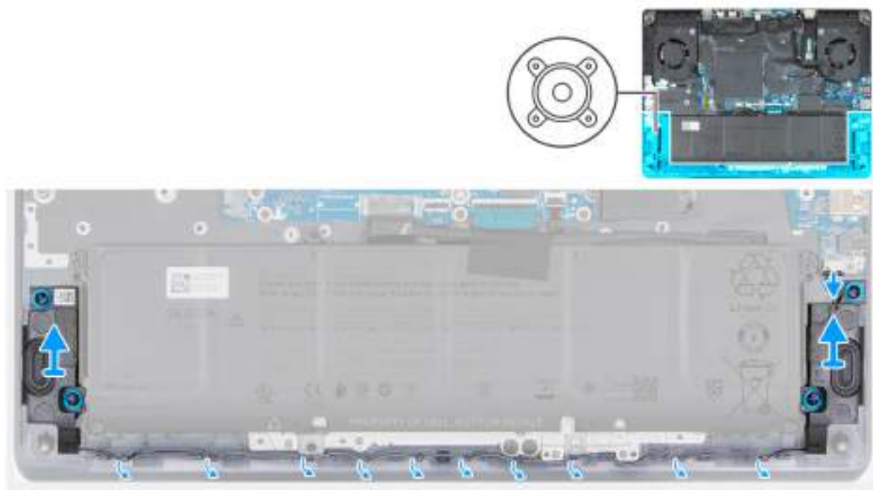
Obrázek 35. Demontáž reproduktorů
