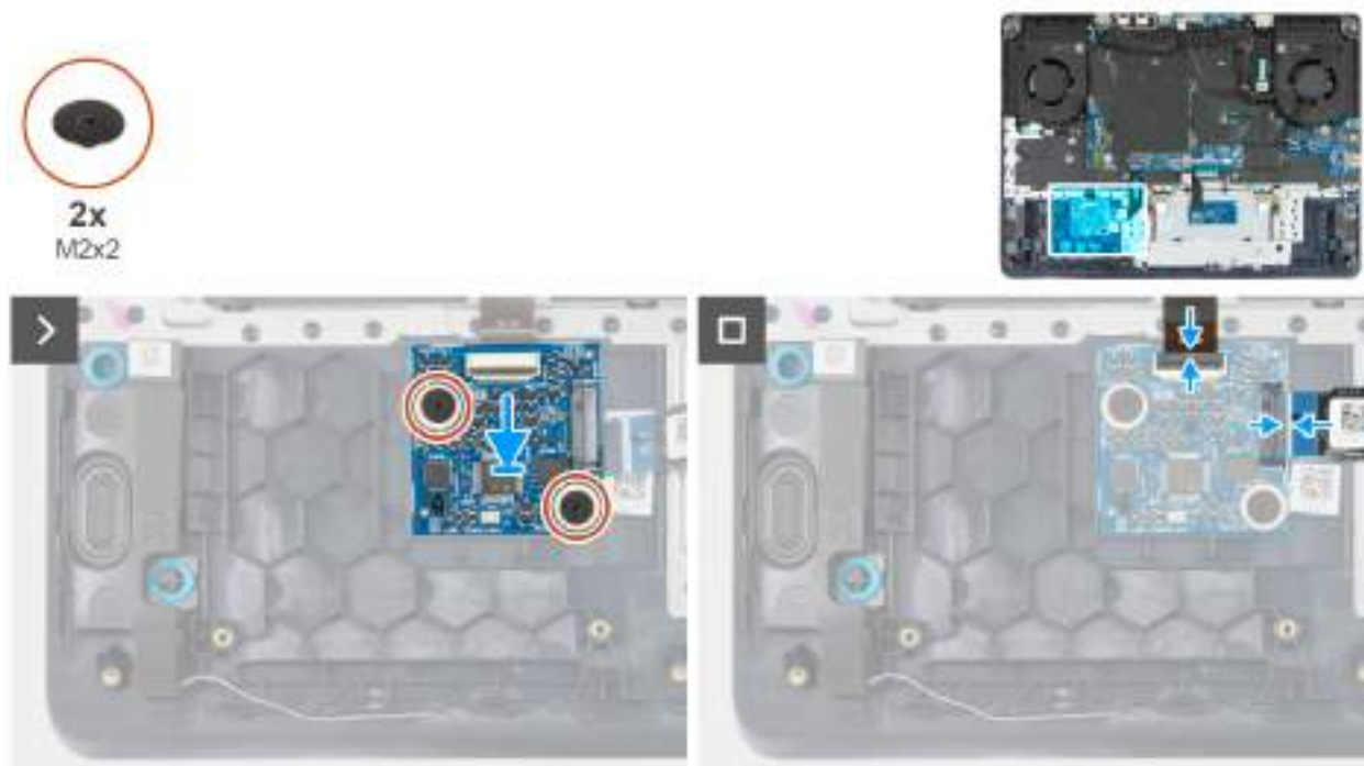
Obrázek 46. Montáž desky řadiče podsvícení klávesnice (ELC)
