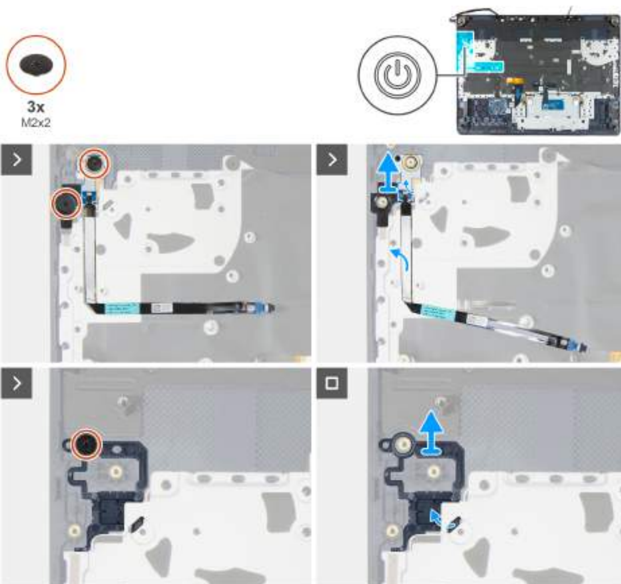
Obrázek 57. Demontáž vypínače a desky vypínače
