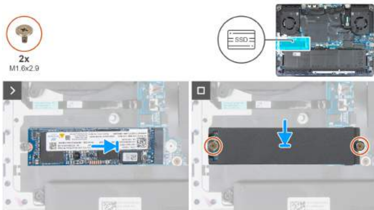
Obrázek 30. Montáž disku SSD M.2 2280 do slotu SSD2
