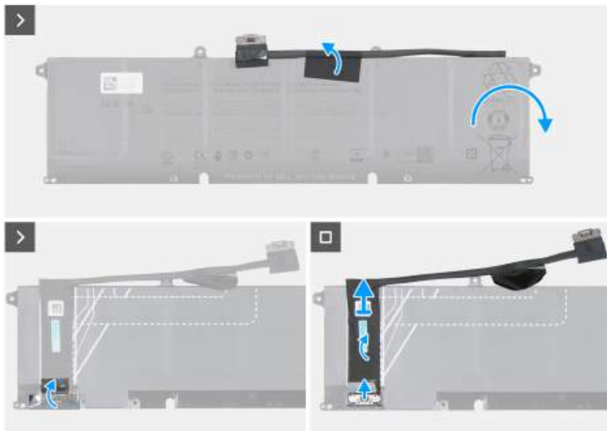
Obrázek 19. Demontáž kabelu baterie
