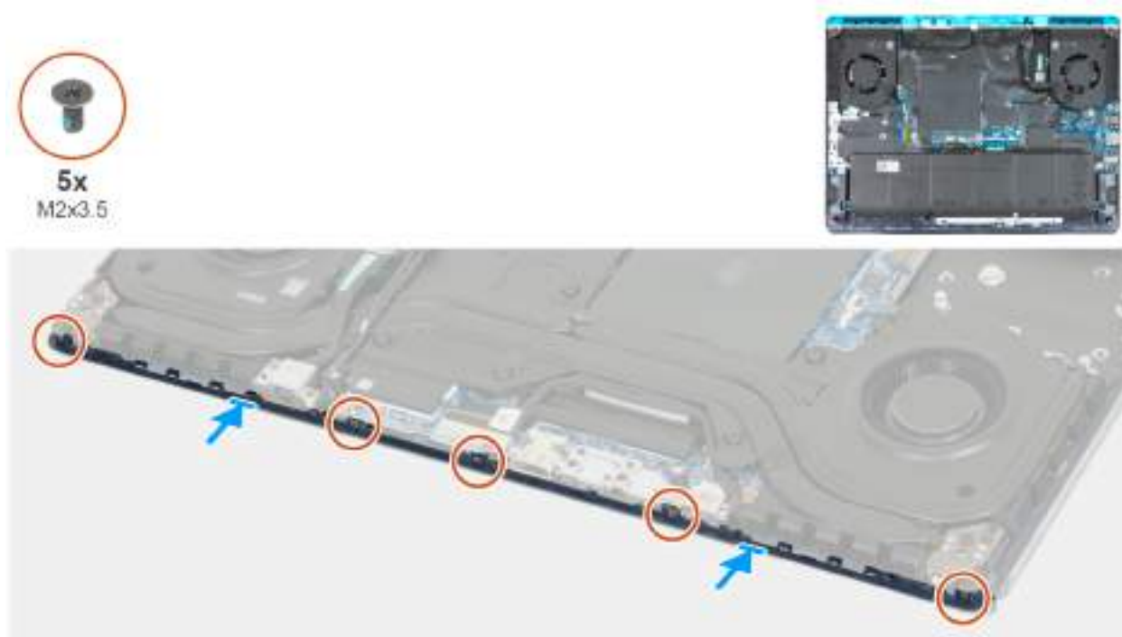
Obrázek 66. Nasazení zadní krytky
