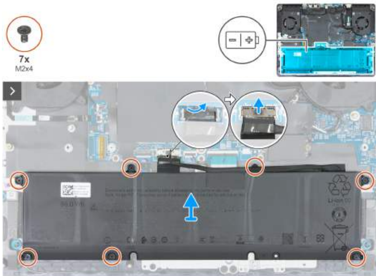
Obrázek 17. Vyjmutí baterie
