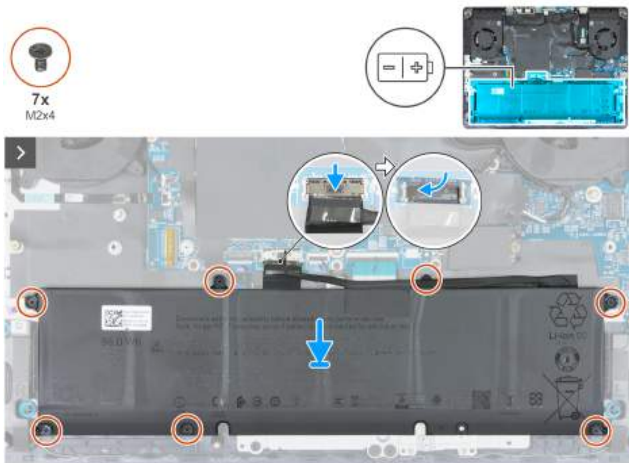
Obrázek 18. Vložení baterie
