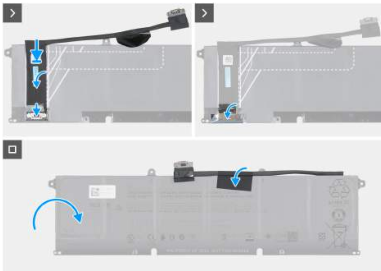
Obrázek 20. Montáž kabelu baterie
