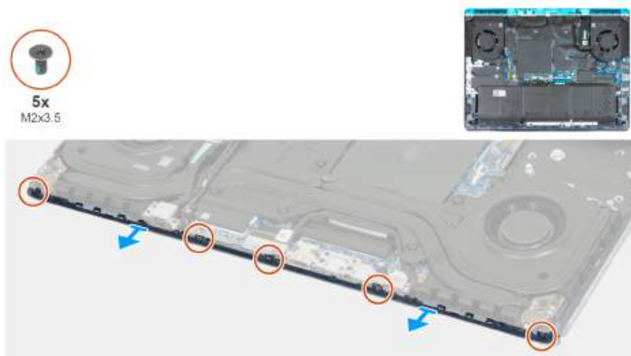
Obrázek 64. Demontáž zadní krytky
