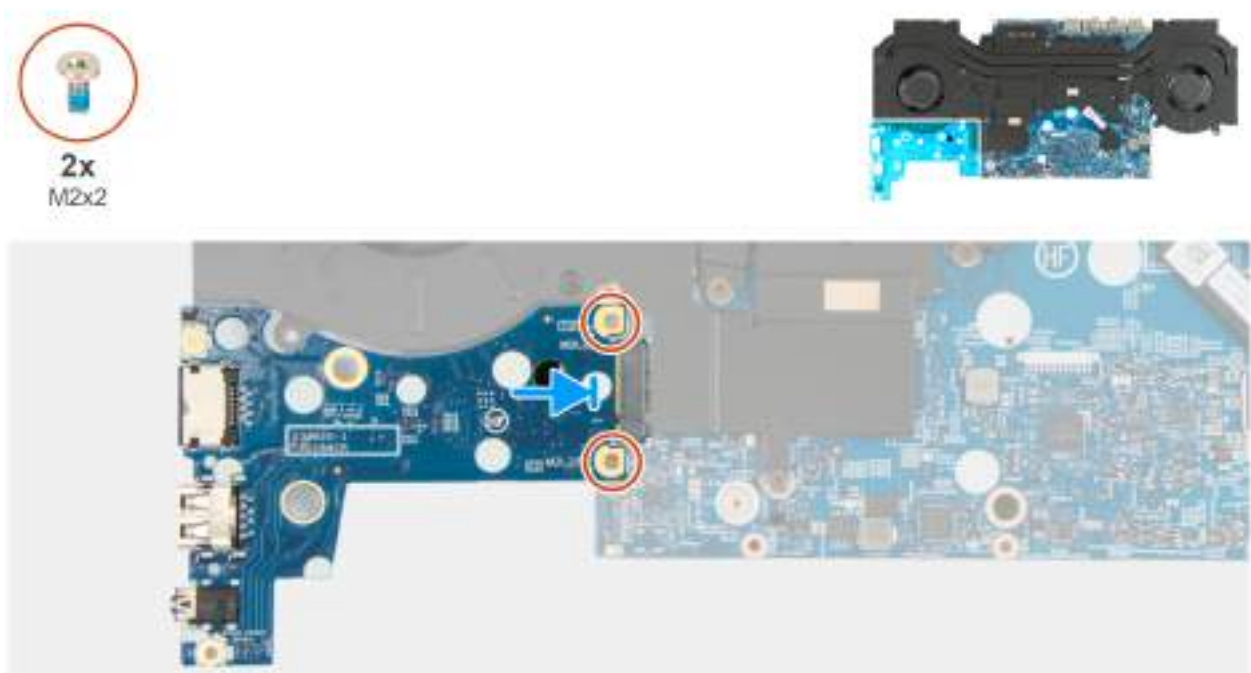
Obrázek 53. Vložení desky I/O
