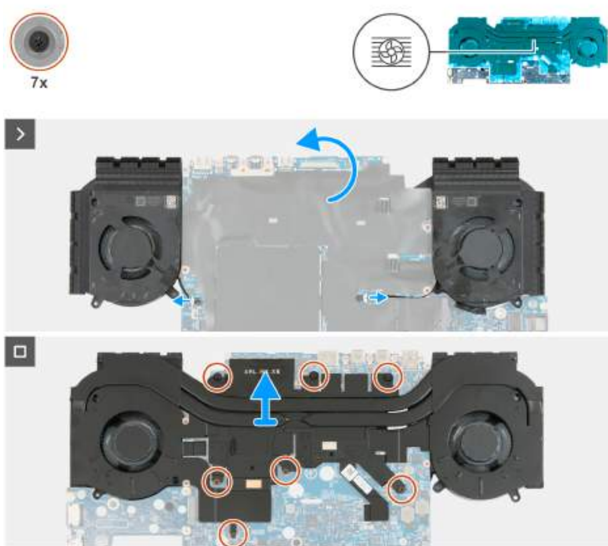
Obrázek 60. Demontáž sestavy ventilátoru a chladiče
