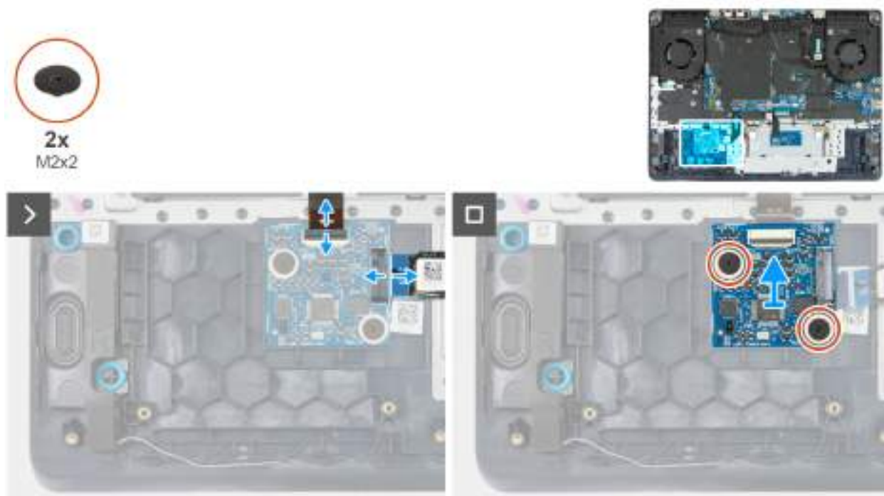
Obrázek 45. Demontáž desky řadiče podsvícení klávesnice (ELC)
