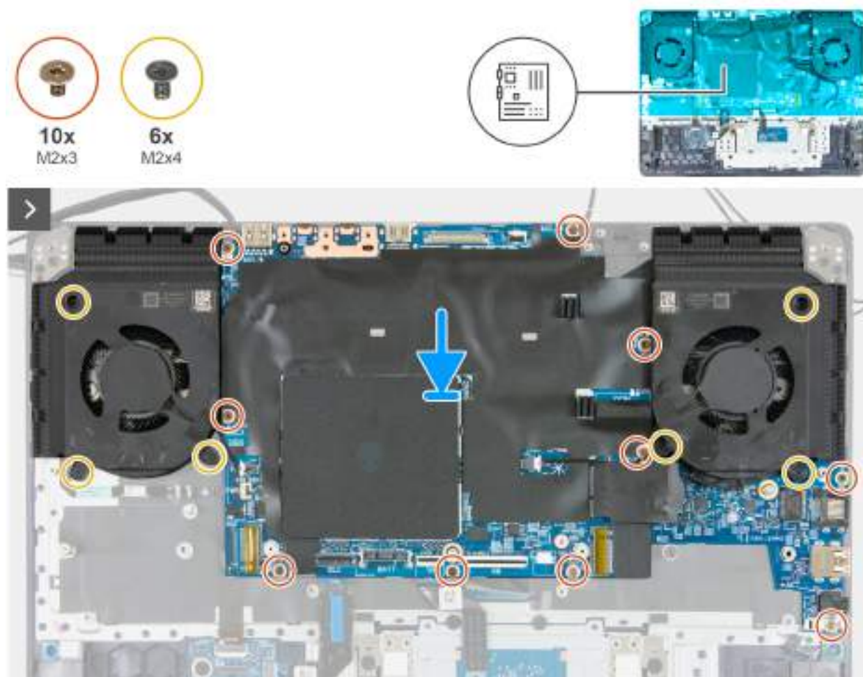
Obrázek 55. Montáž základní desky
