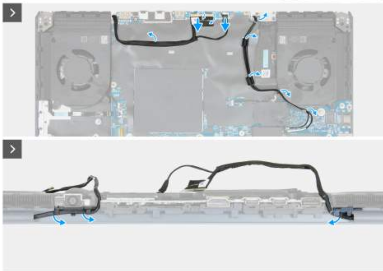
Obrázek 71. Demontáž sestavy displeje
