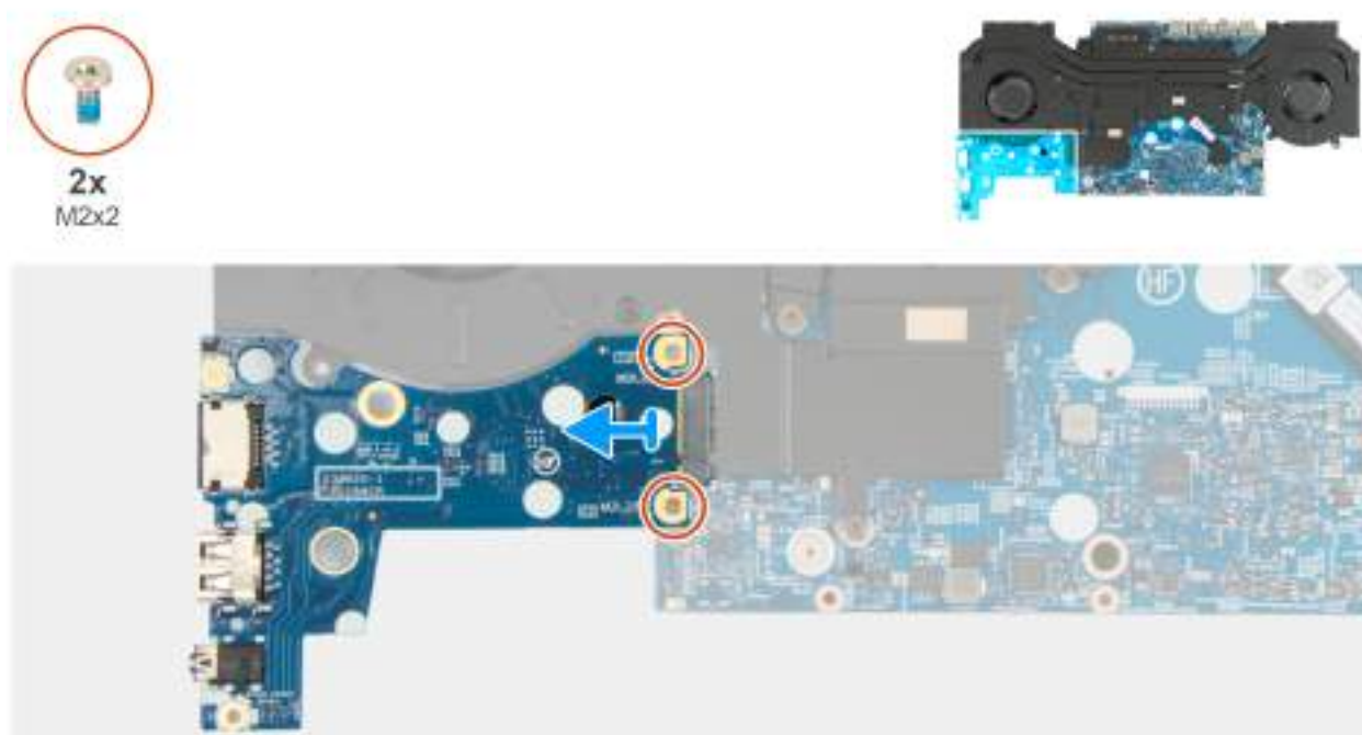
Obrázek 62. Demontáž desky I/O
