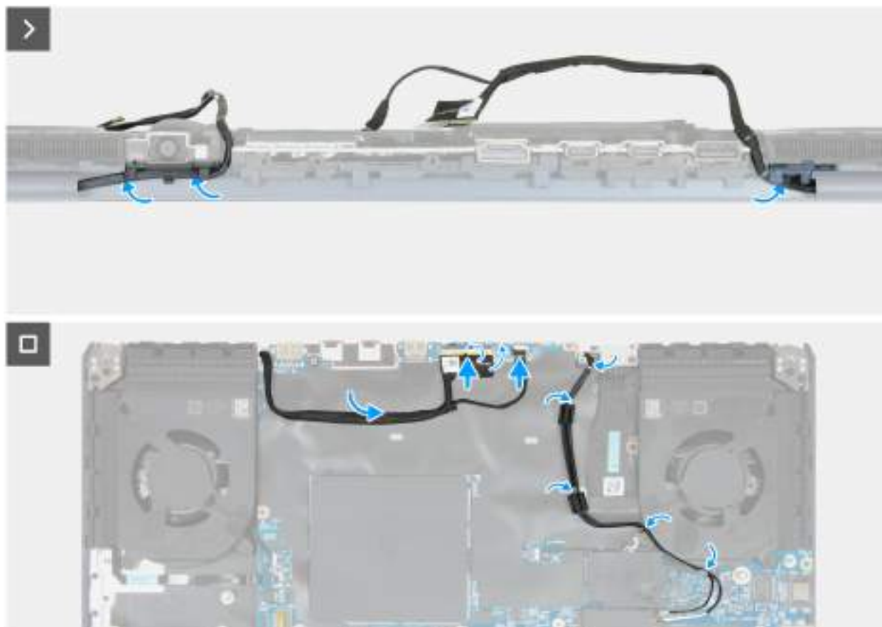
Obrázek 75. Montáž sestavy displeje
