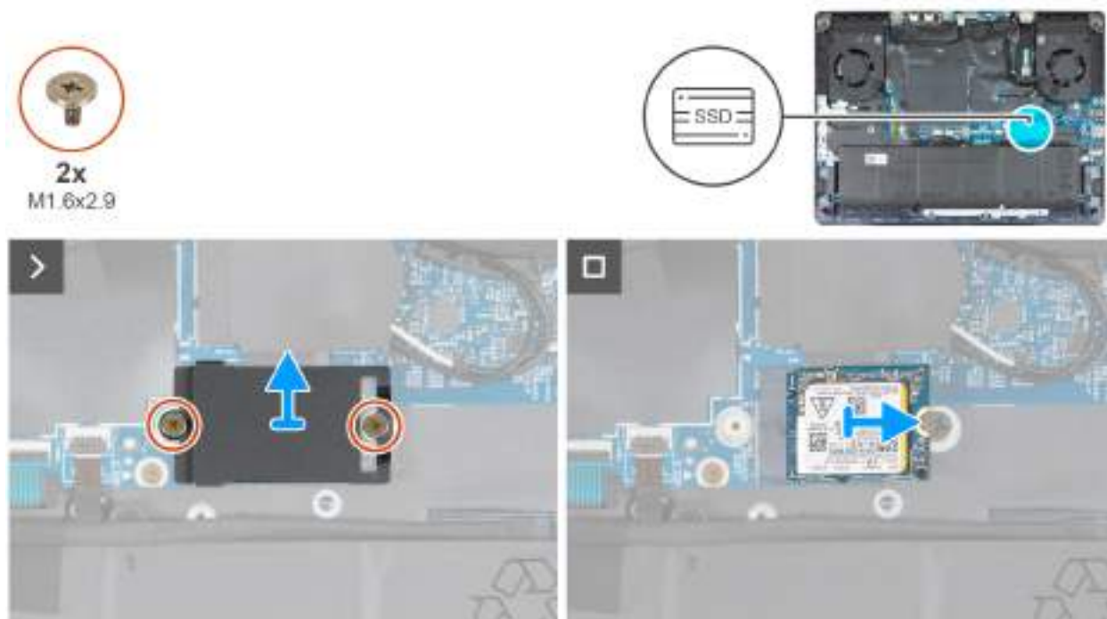
Obrázek 23. Vyjmutí disku SSD M.2 2230 ze slotu SSD1
