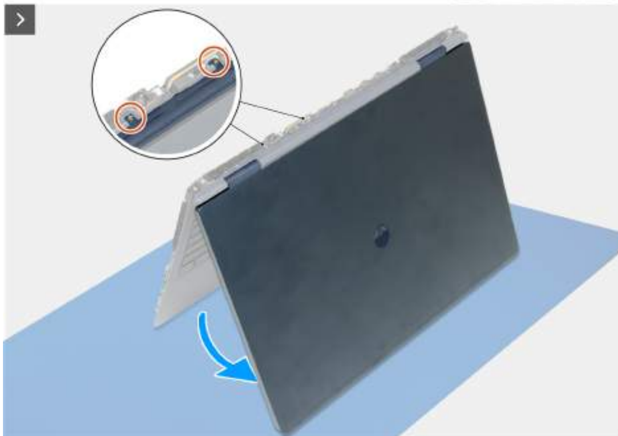
Obrázek 67. Demontáž středového panelu
