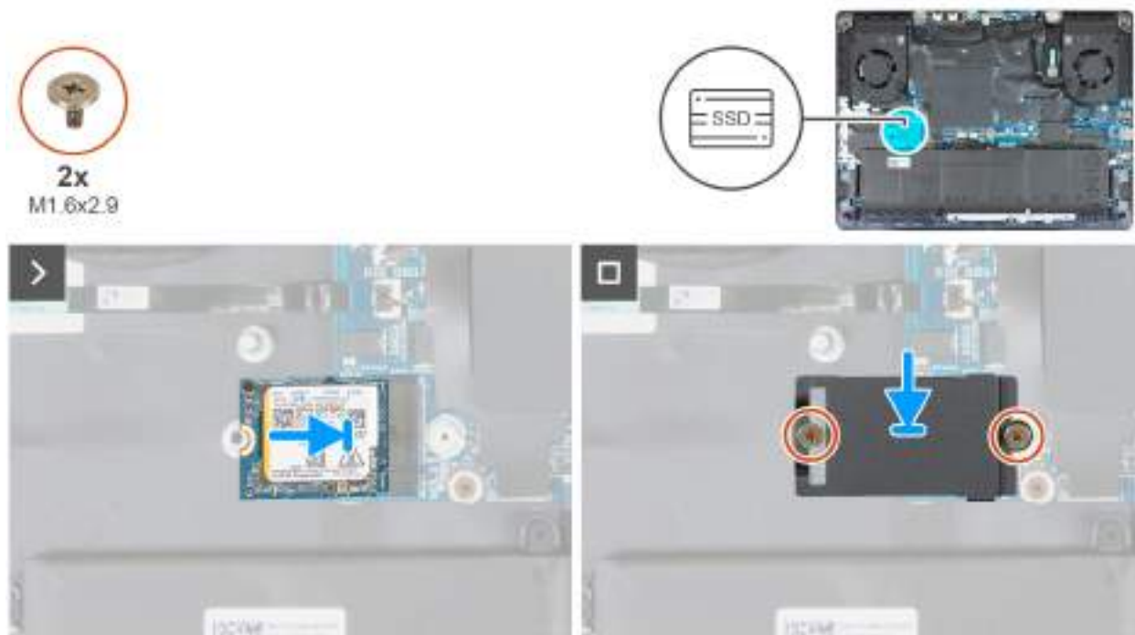
Obrázek 26. Montáž disku SSD M.2 2230 do slotu SSD2
