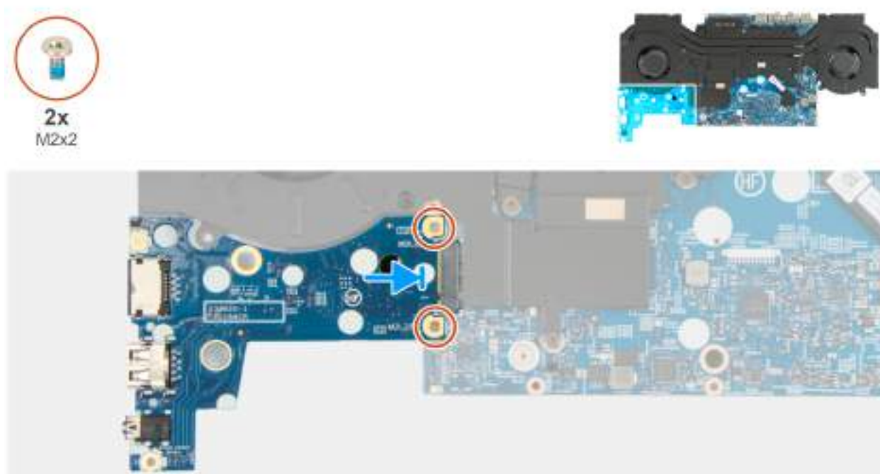
Obrázek 63. Vložení desky I/O
