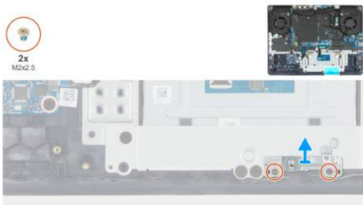
Obrázek 41. Demontáž držáku baterie
