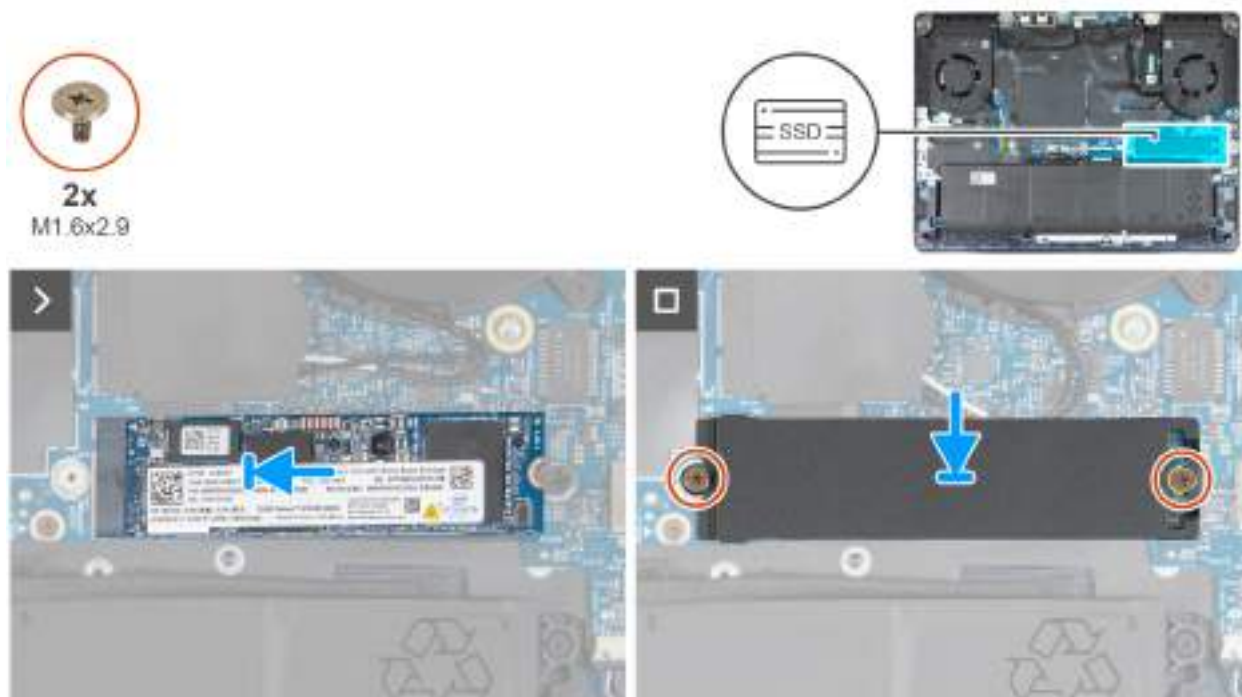
Obrázek 28. Montáž disku SSD M.2 2280 do slotu SSD1
