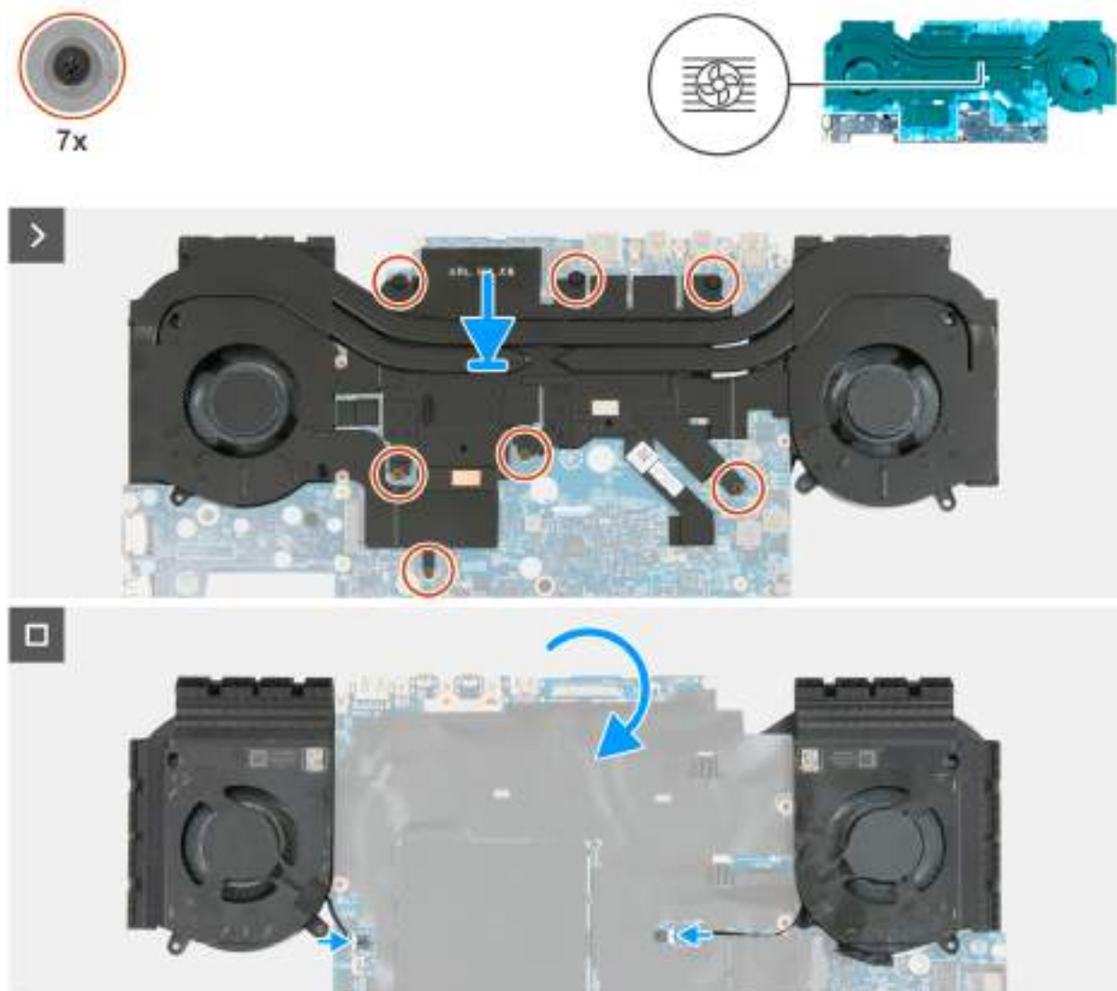
Obrázek 61. Montáž sestavy ventilátoru a chladiče
