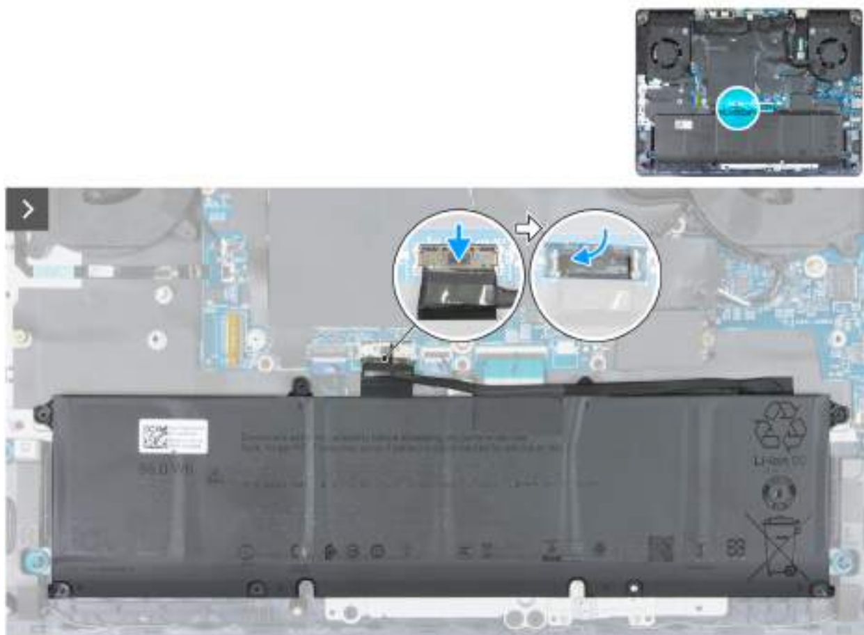
Obrázek 14. Připojení kabelu baterie
