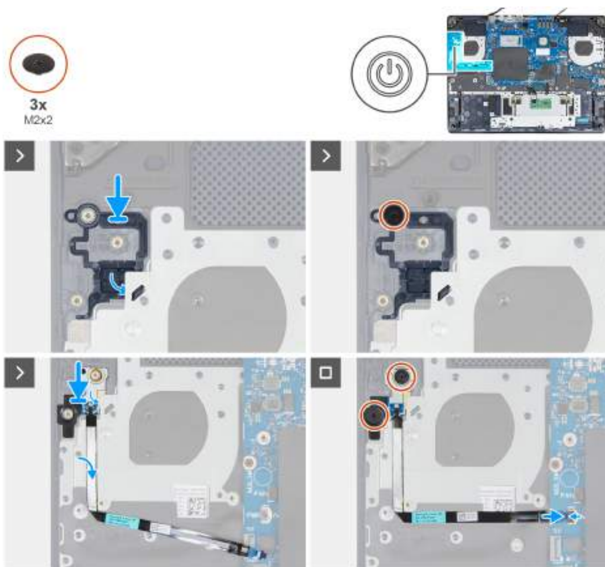
Obrázek 59. Montáž vypínače a desky vypínače
