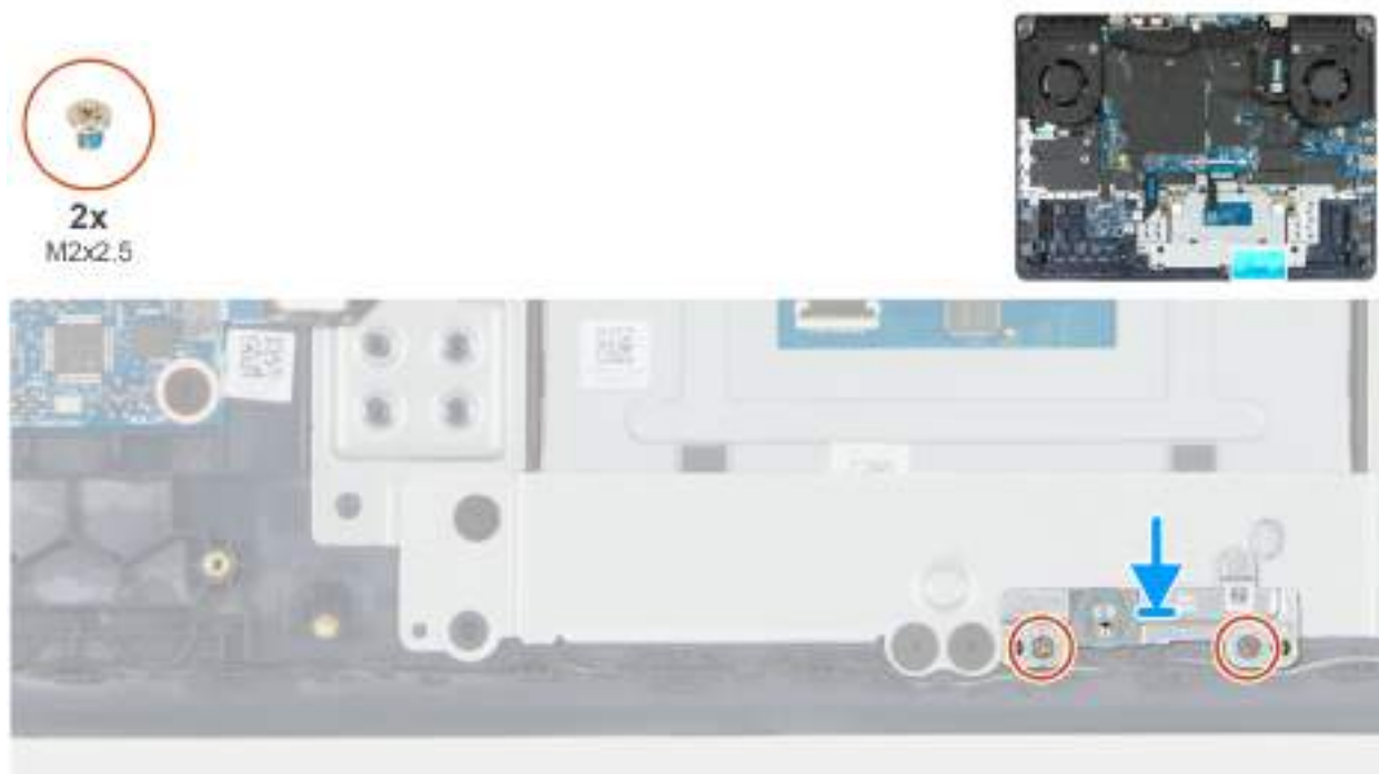
Obrázek 42. Montáž držáku baterie
