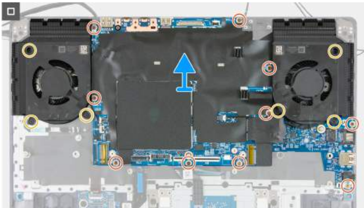
Obrázek 49. Demontáž základní desky
