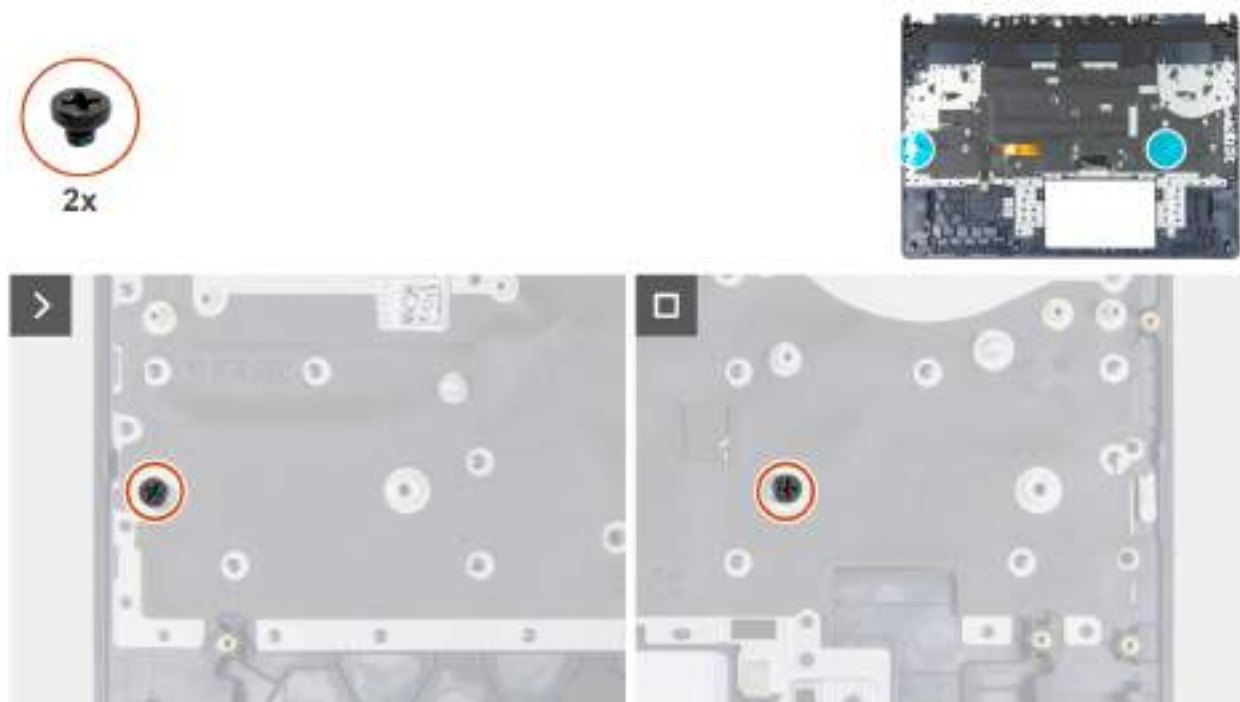
Obrázek 78. Montáž šroubových držáků disku SSD
