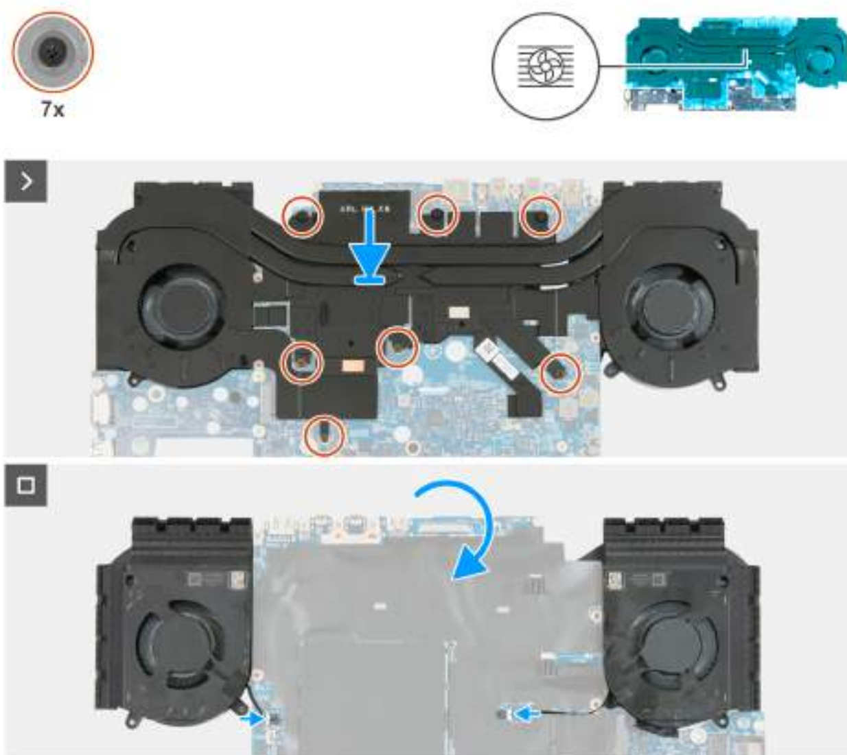
Obrázek 54. Montáž sestavy ventilátoru a chladiče
