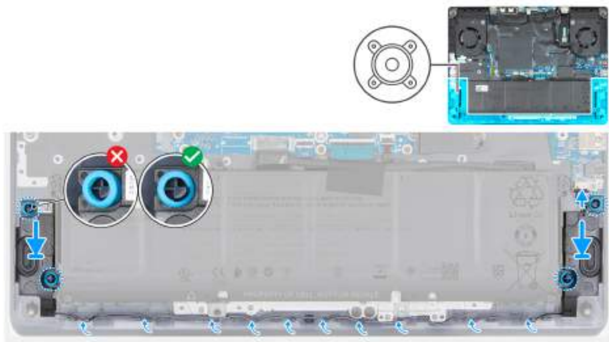
Obrázek 36. Montáž reproduktorů
