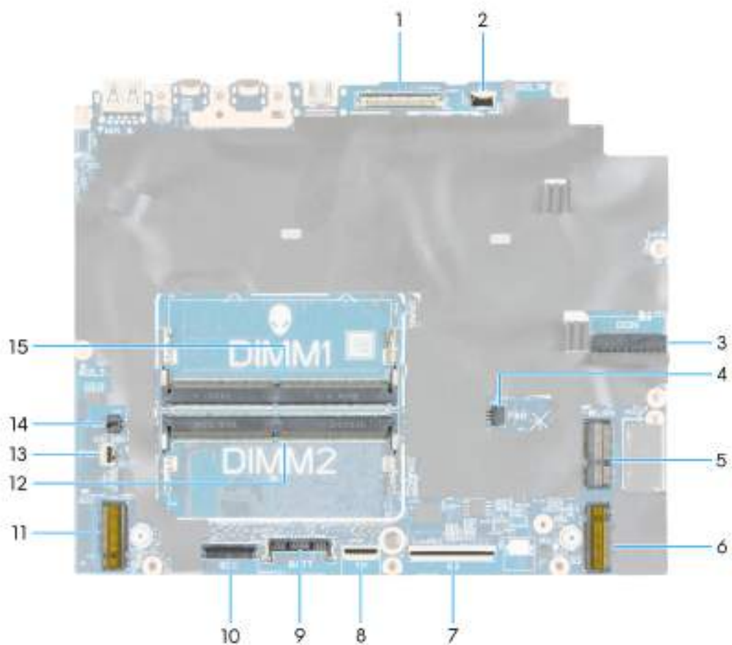
Obrázek 47. Konektory na základní desce
