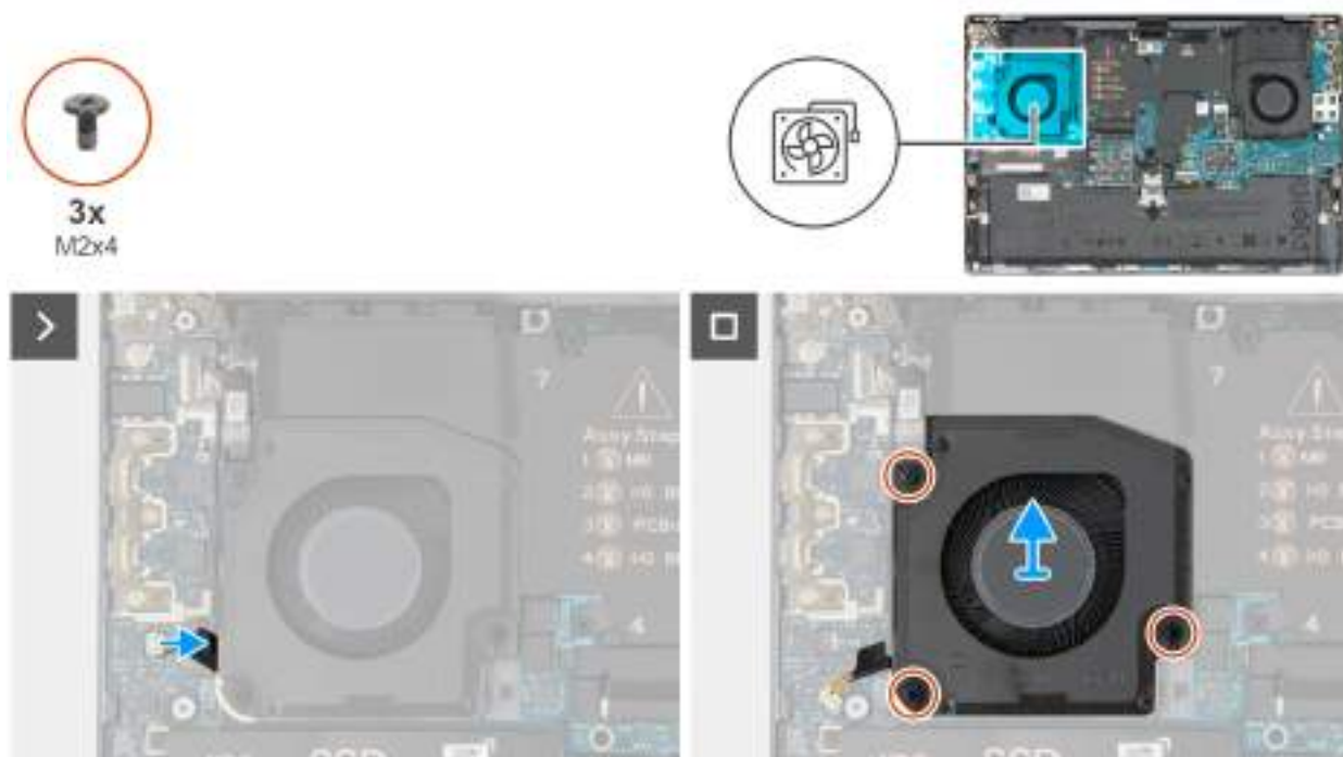
Obrázek 29. Demontáž pravého ventilátoru
