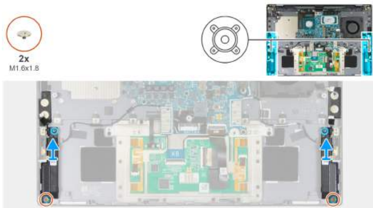
Obrázek 69. Demontáž reproduktorů
