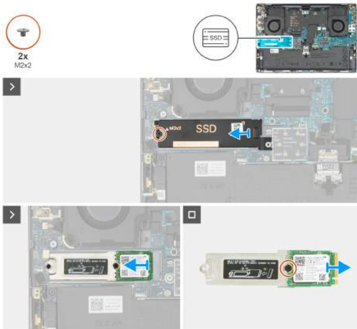
Obrázek 25. Demontáž disku SSD M.2 2230
