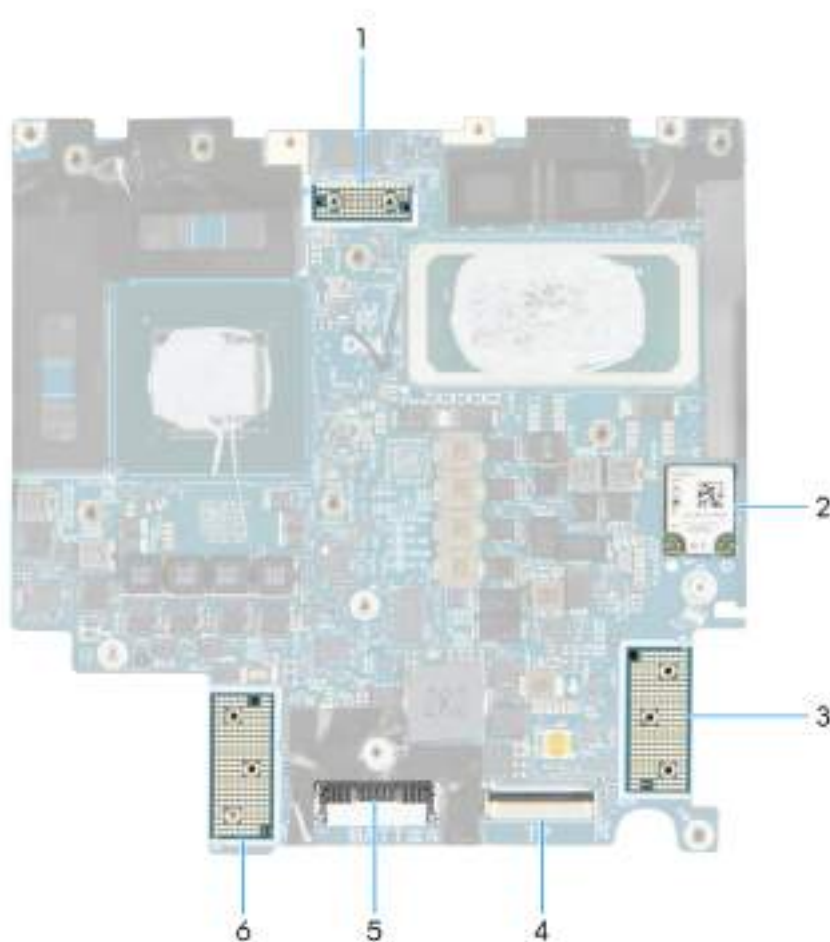
Obrázek 62. Konektory základní desky
