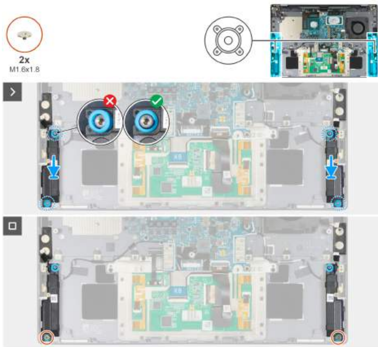
Obrázek 70. Montáž reproduktorů
