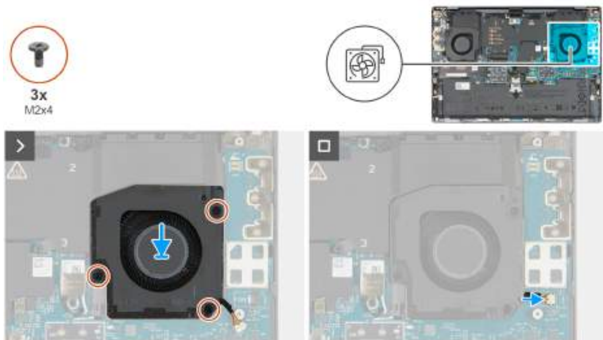
Obrázek 28. Montáž levého ventilátoru
