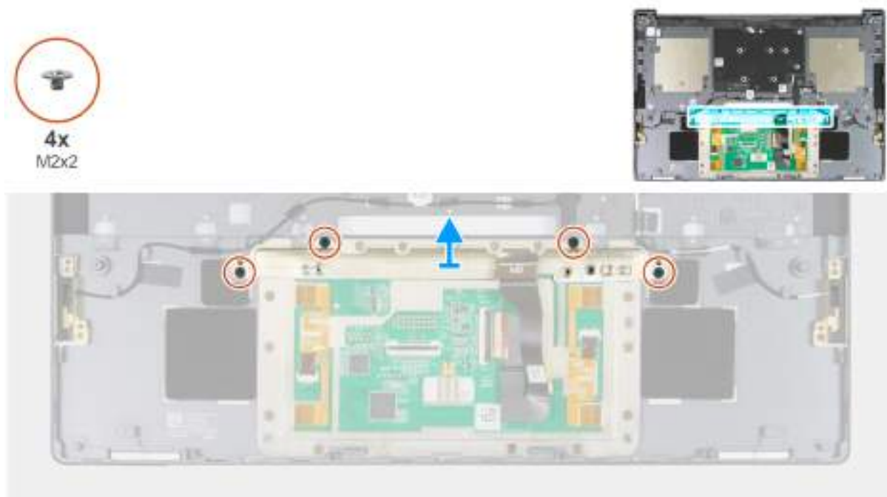
Obrázek 77. Demontáž držáku dotykové podložky
