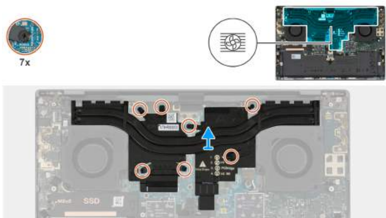
Obrázek 41. Demontáž chladiče
