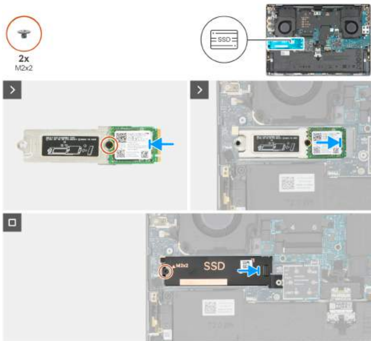
Obrázek 26. Instalace disku SSD M.2 2230
