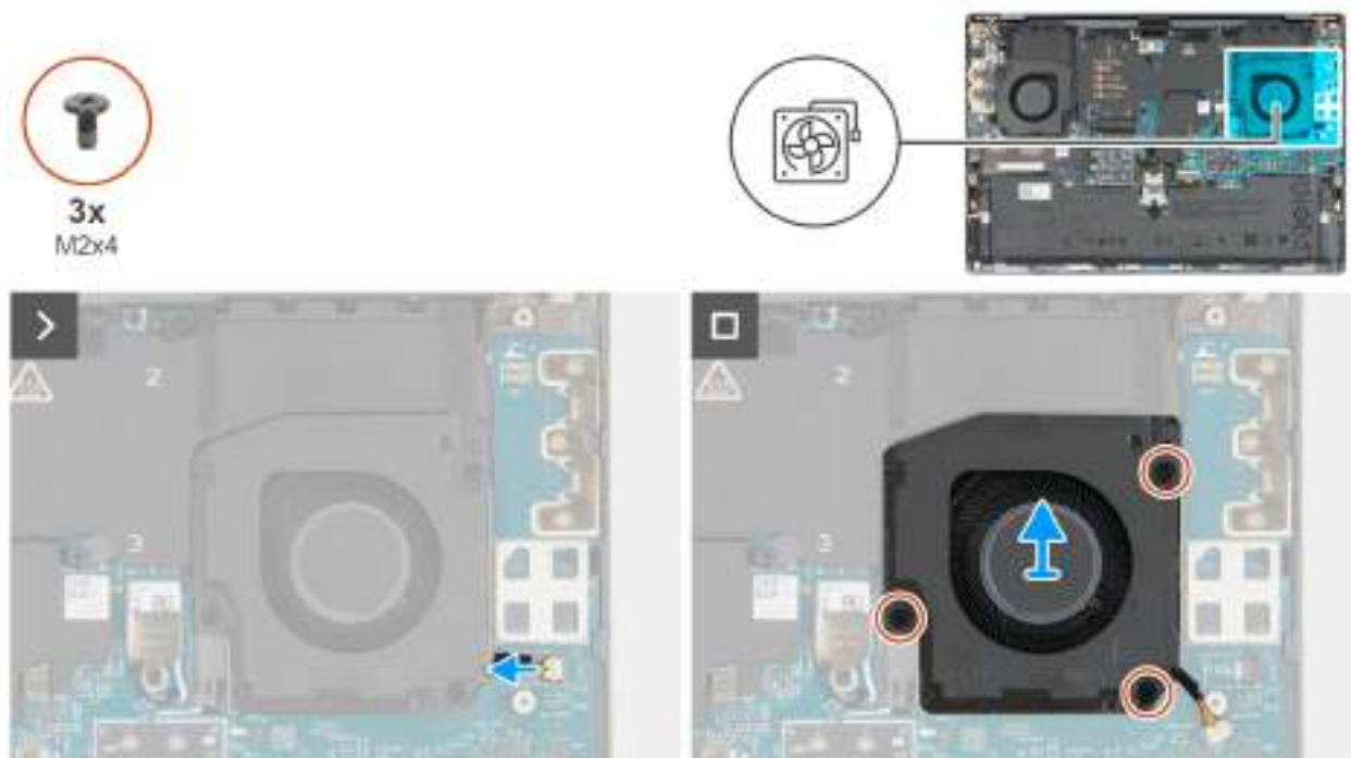
Obrázek 27. Demontáž levého ventilátoru
