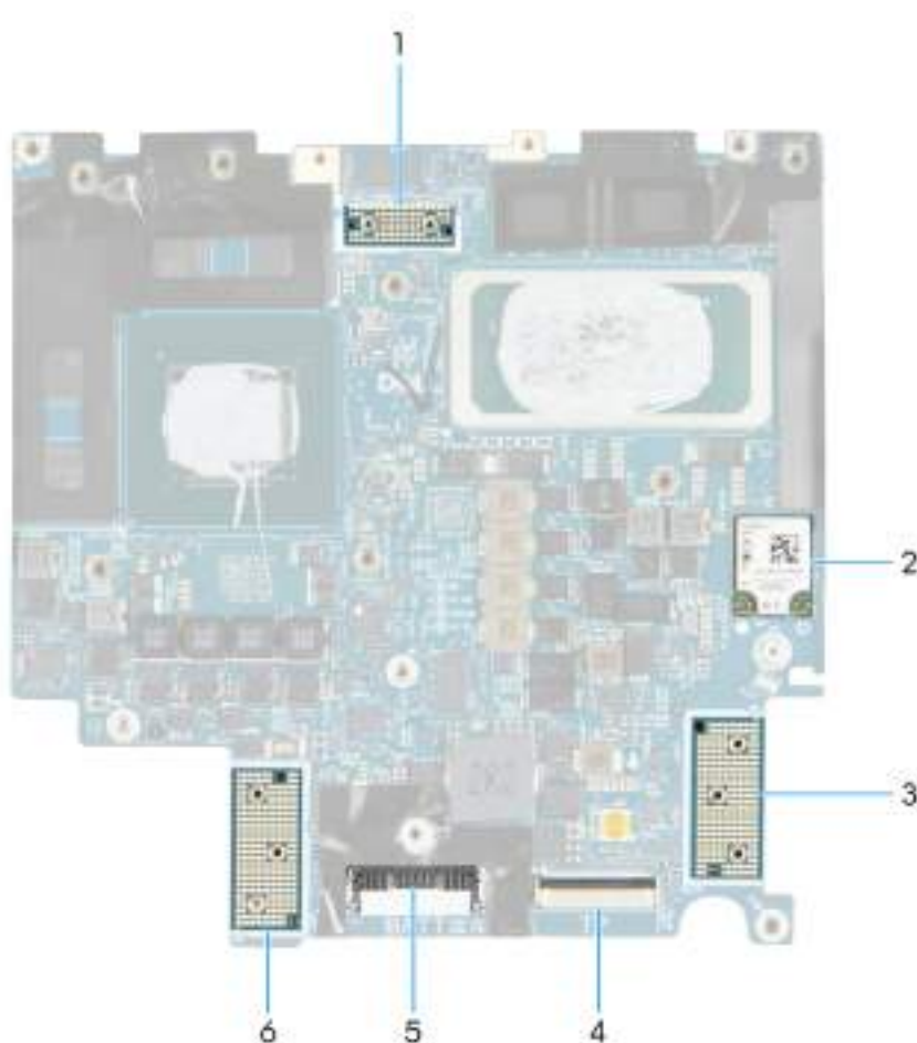
Obrázek 58. Konektory základní desky
