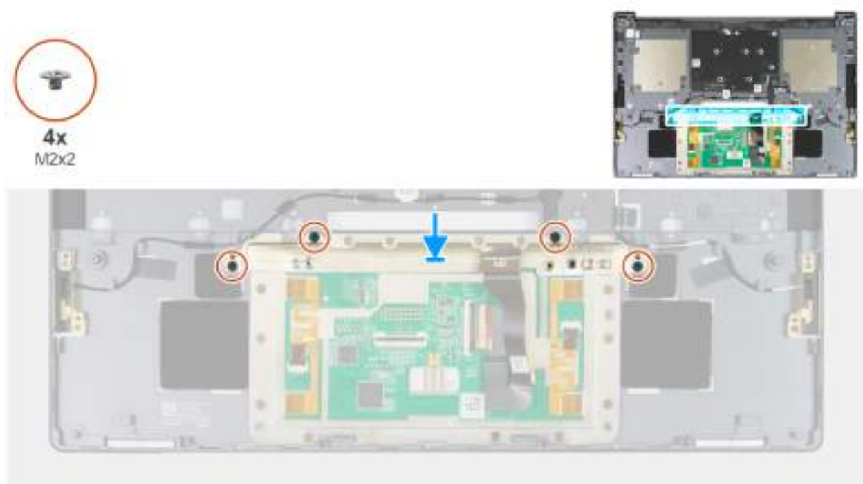
Obrázek 80. Montáž držáku dotykové podložky
