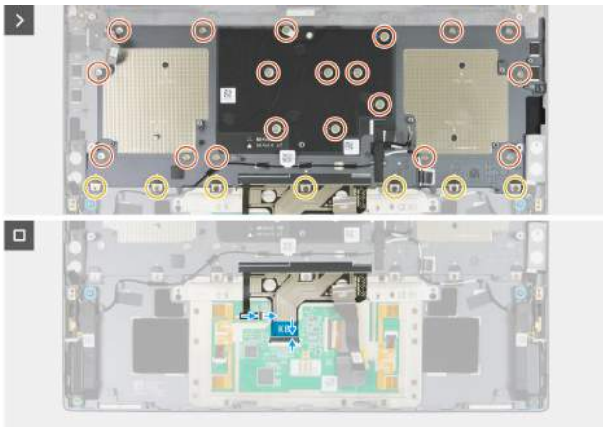
Obrázek 76. Montáž klávesnice
