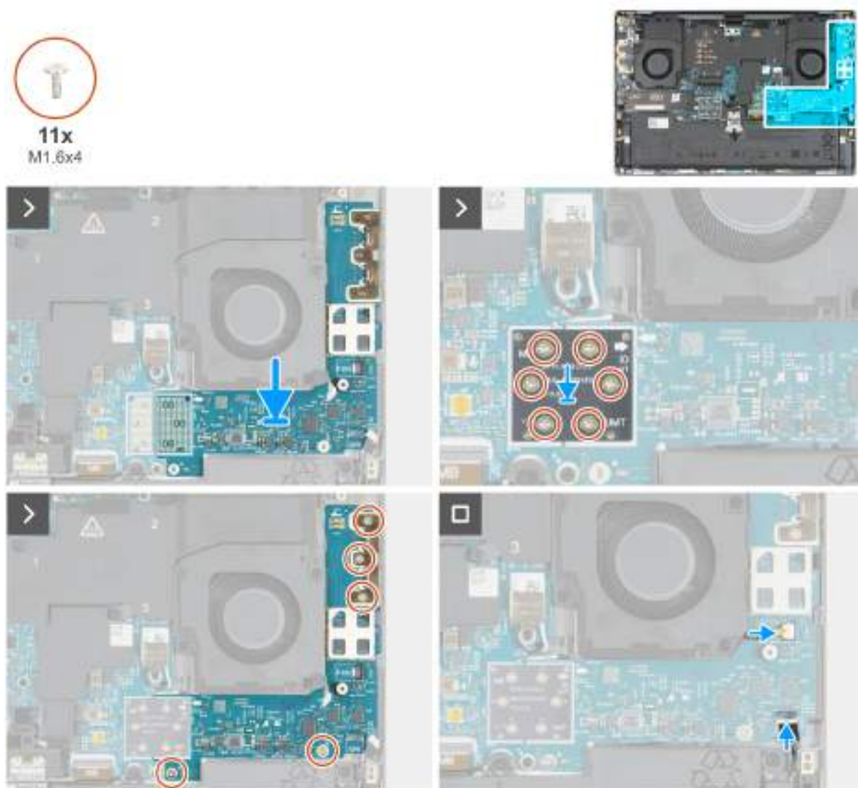
Obrázek 46. Instalace levé desky I/O
