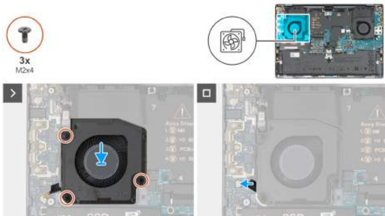
Obrázek 30. Montáž pravého ventilátoru
