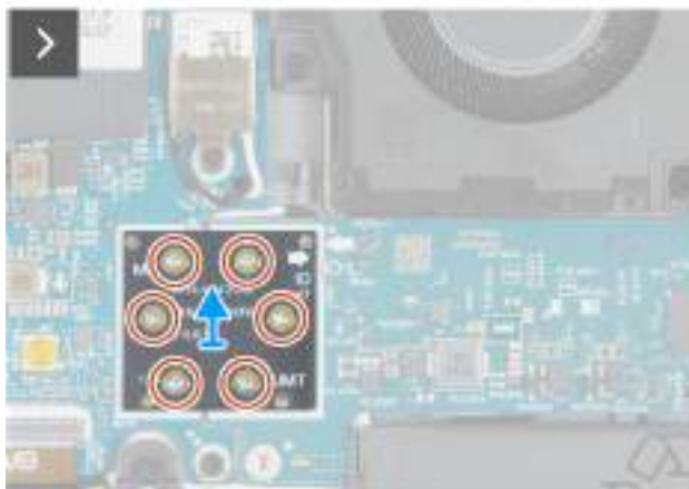
Obrázek 45. Demontáž levé desky I/O
