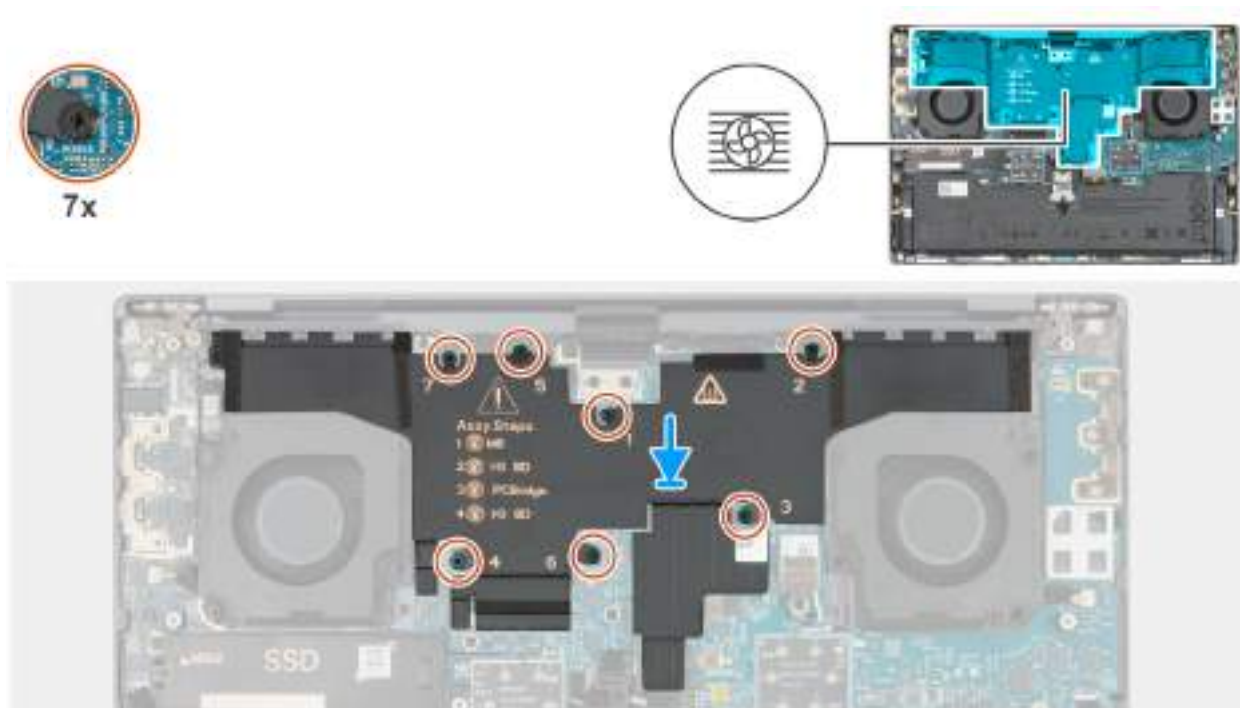
Obrázek 44. Montáž chladiče
