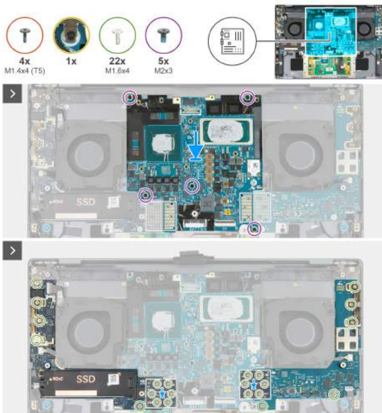
Obrázek 63. Montáž základní desky (samostatná grafická karta)
