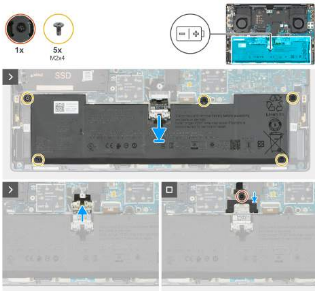
Obrázek 19. Vložení baterie
