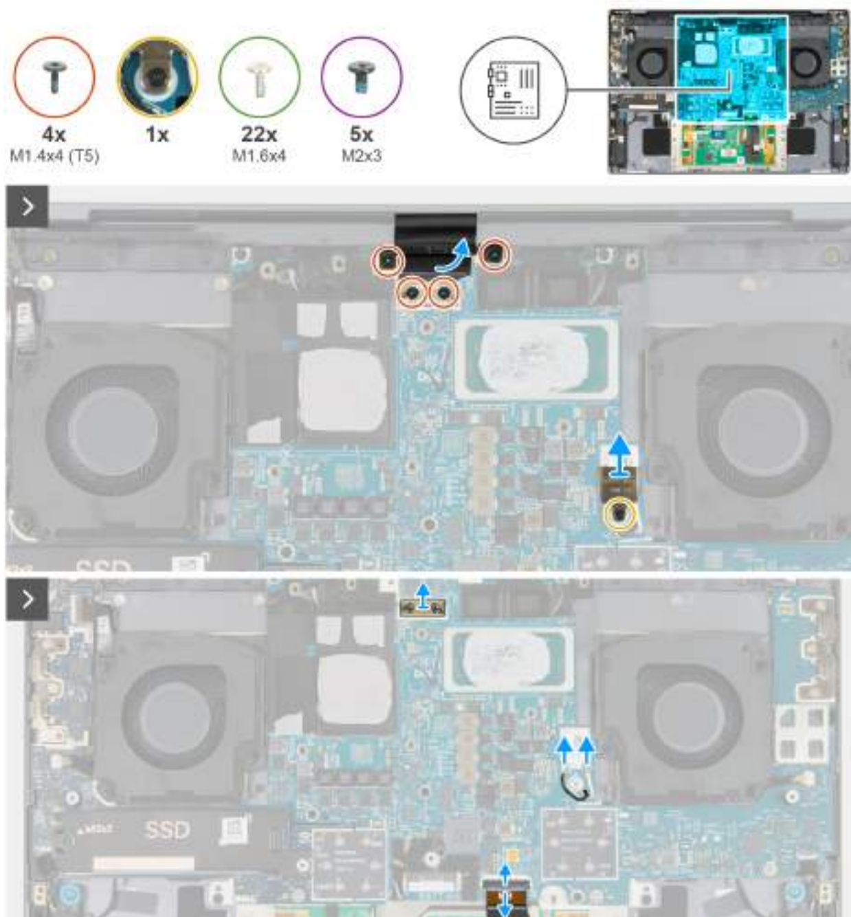
Obrázek 50. Demontáž základní desky (integrovaná grafická karta)
