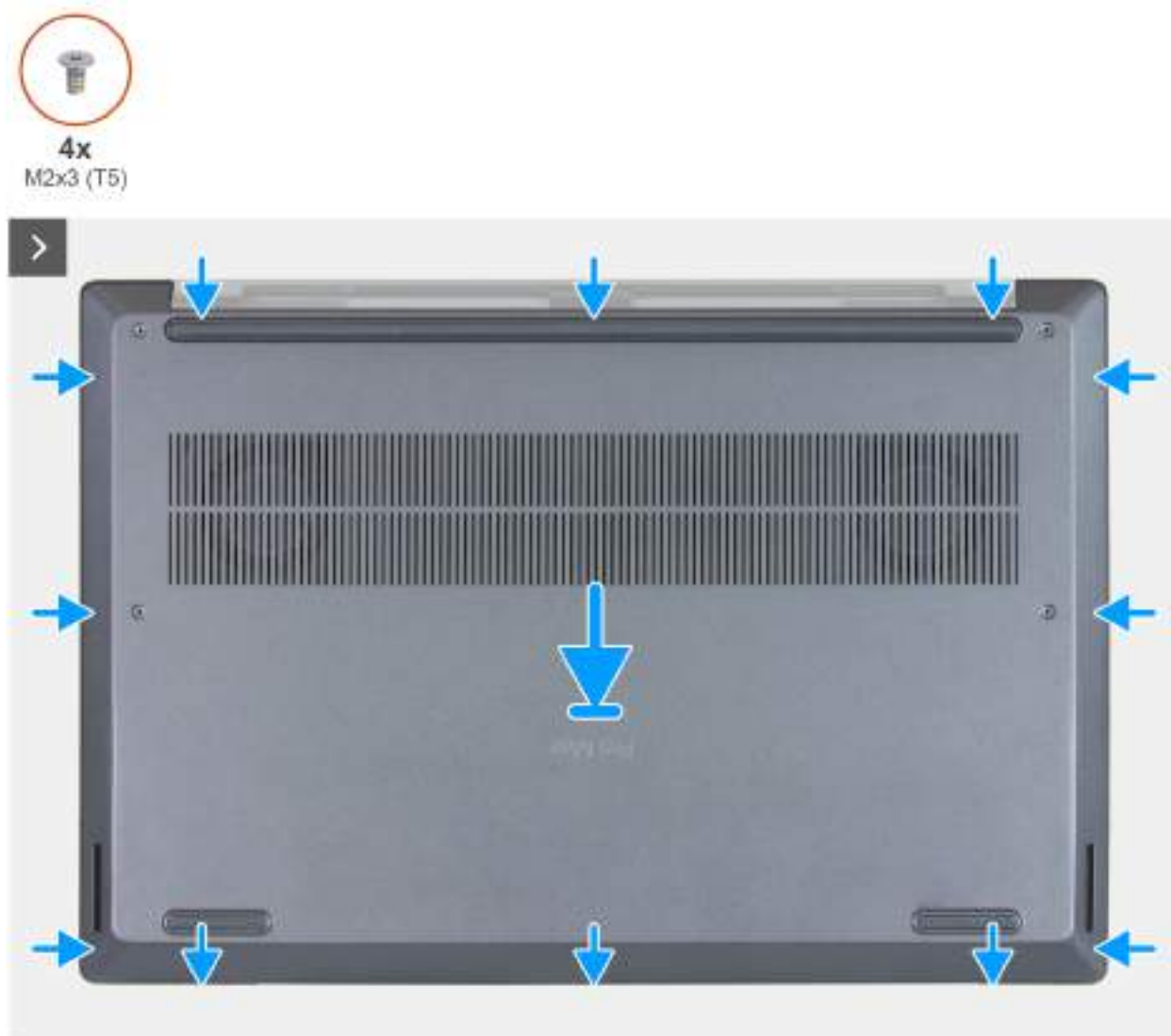
Obrázek 14. Nasazení spodního krytu
