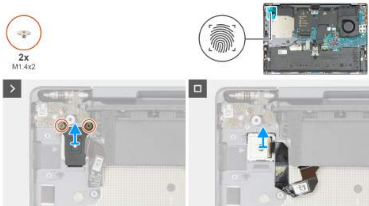
Obrázek 67. Demontáž vypínače nebo čtečky otisků prstů
