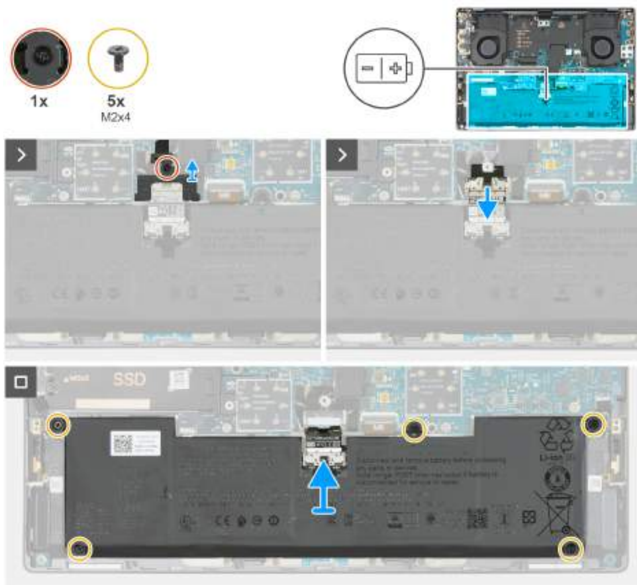
Obrázek 17. Vyjmutí baterie
