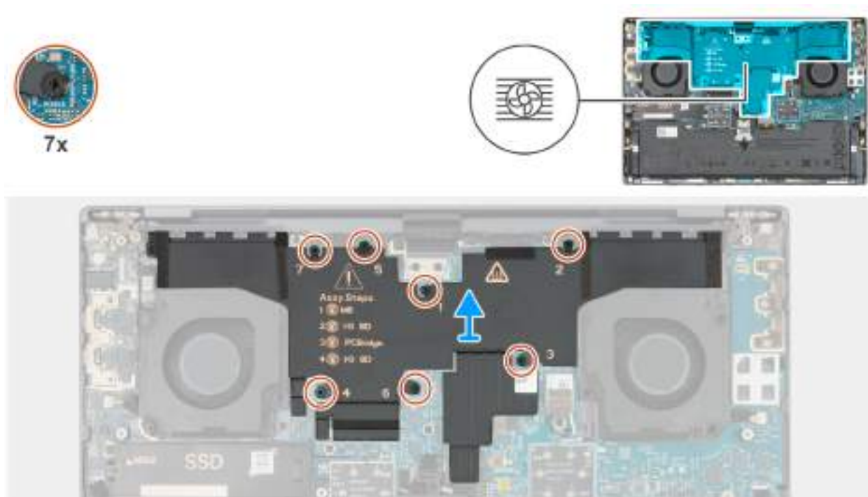
Obrázek 43. Demontáž chladiče
