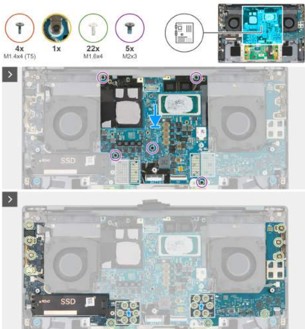
Obrázek 54. Montáž základní desky (integrovaná grafická karta)
