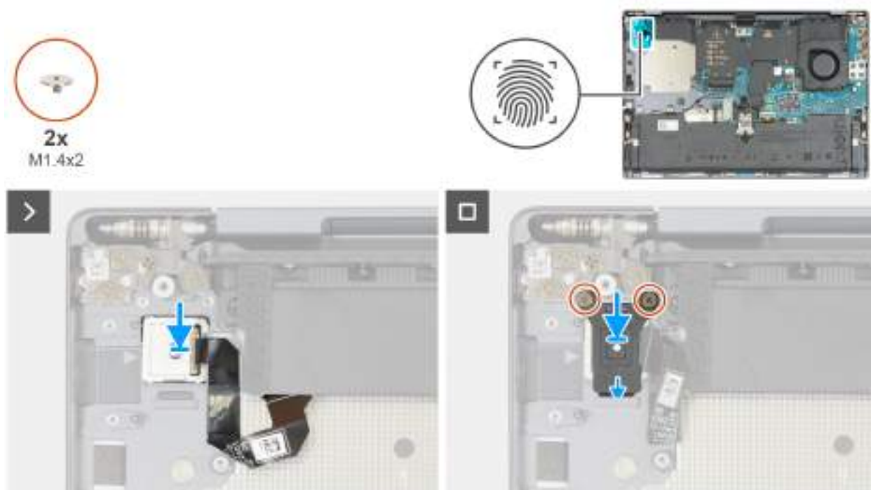
Obrázek 68. Montáž vypínače nebo čtečky otisků prstů
