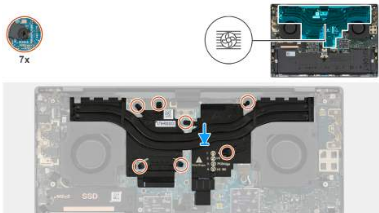
Obrázek 42. Montáž chladiče
