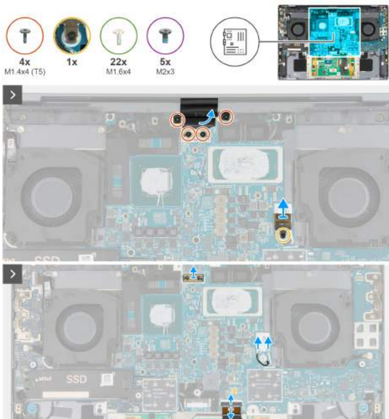
Obrázek 59. Demontáž základní desky (samostatná grafická karta)
