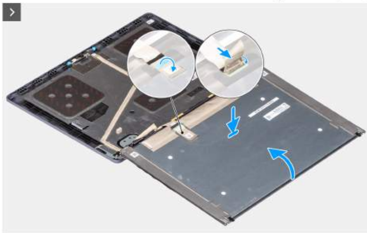
Obrázek 60. Montáž obrazovky displeje
