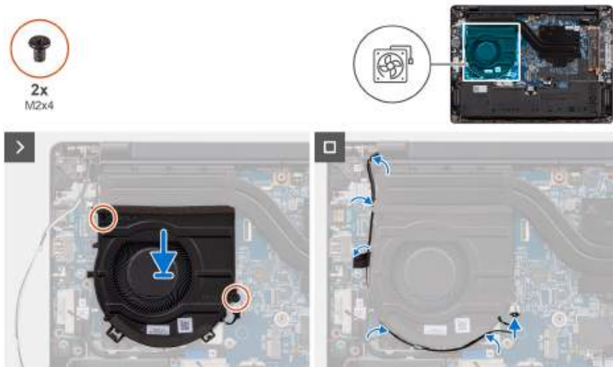
Obrázek 30. Montáž ventilátoru
