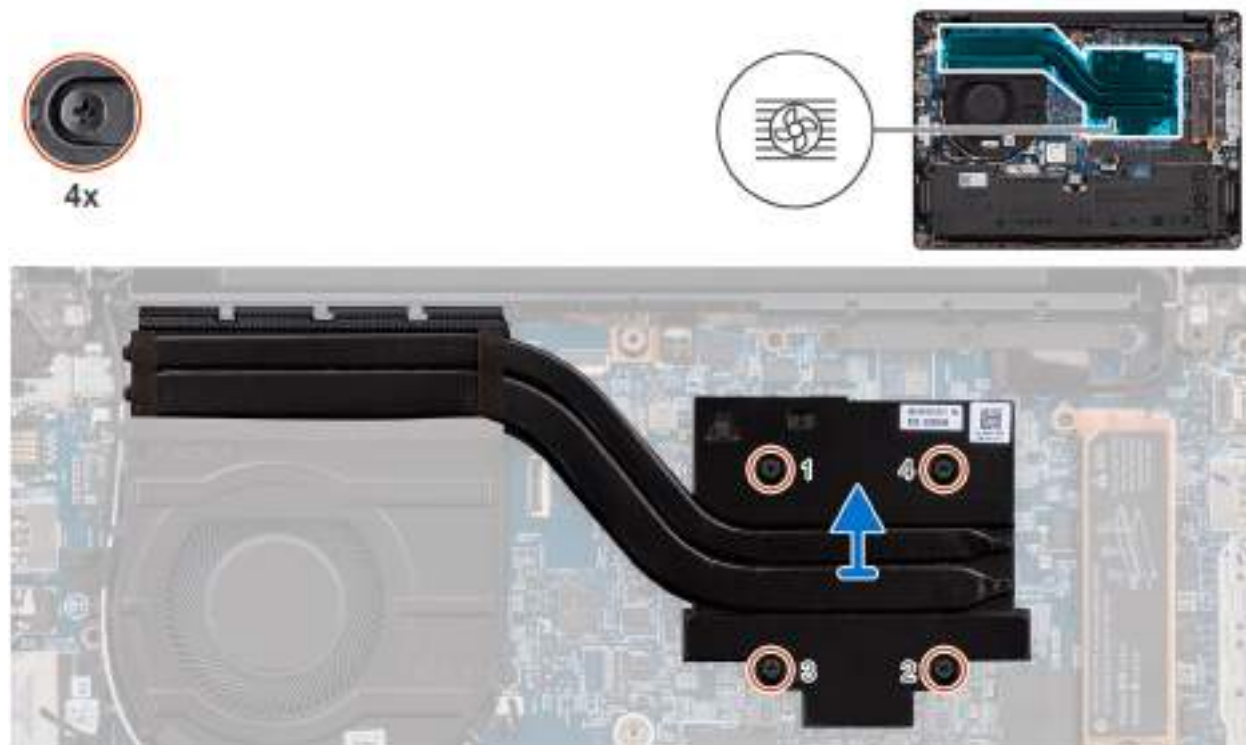
Obrázek 37. Demontáž chladiče
