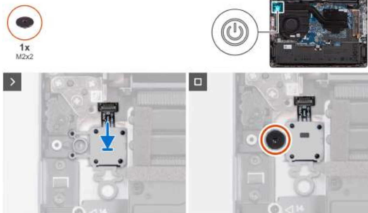
Obrázek 42. Montáž vypínače
