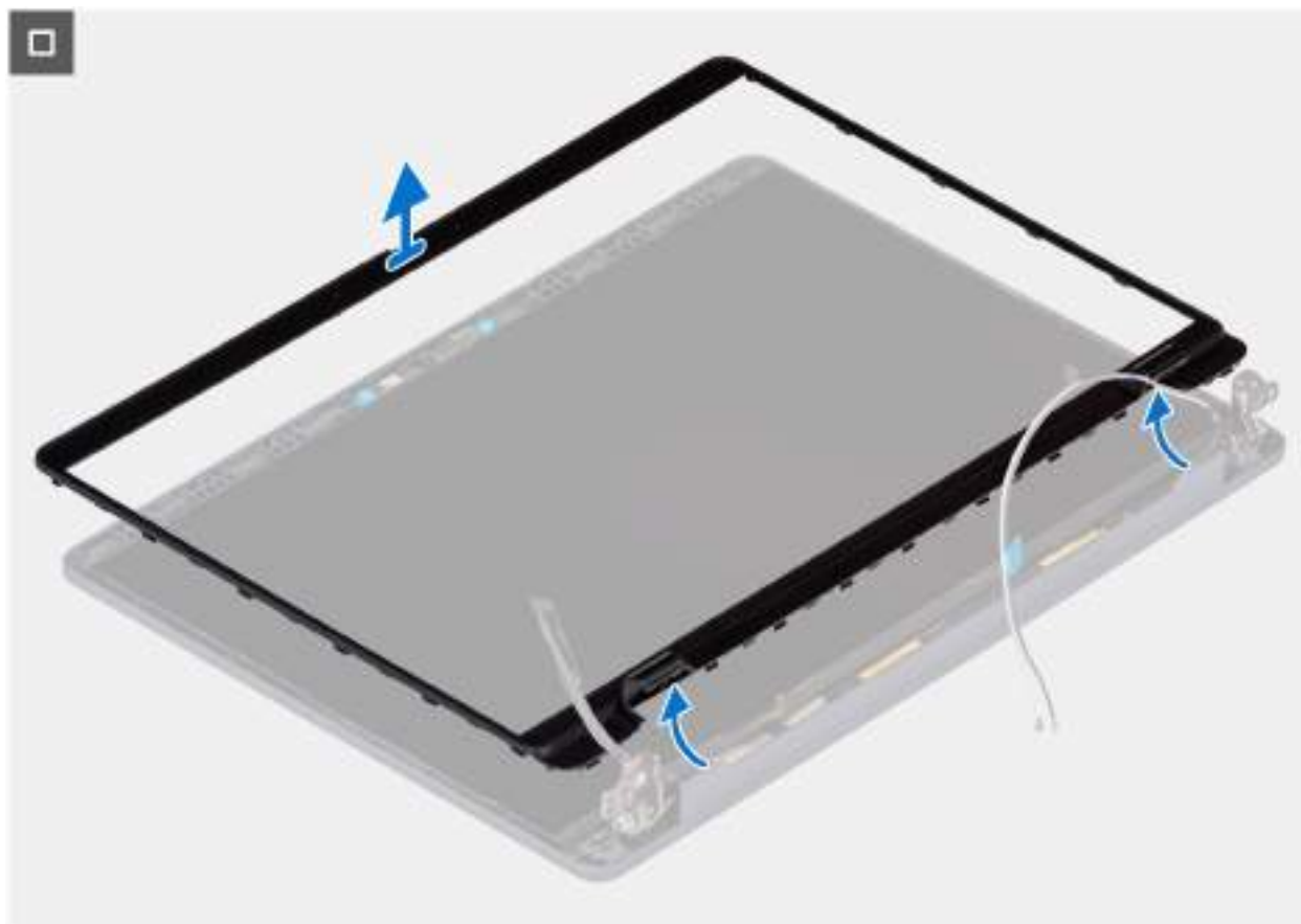
Obrázek 53. Demontáž čelního krytu displeje
