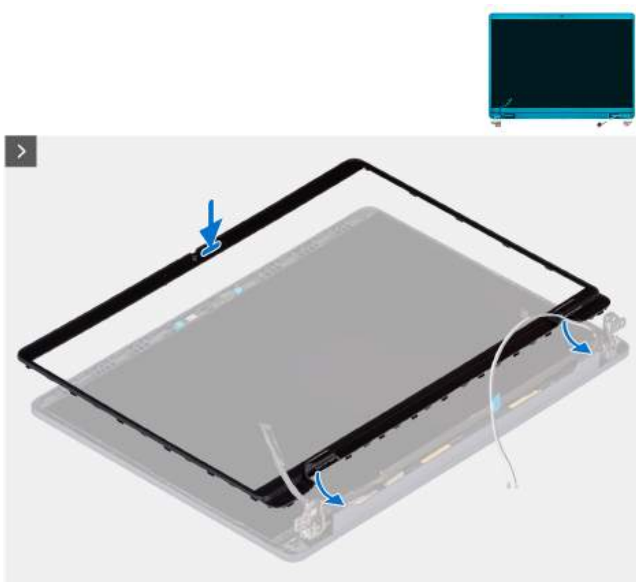
Obrázek 54. Montáž čelního krytu displeje
