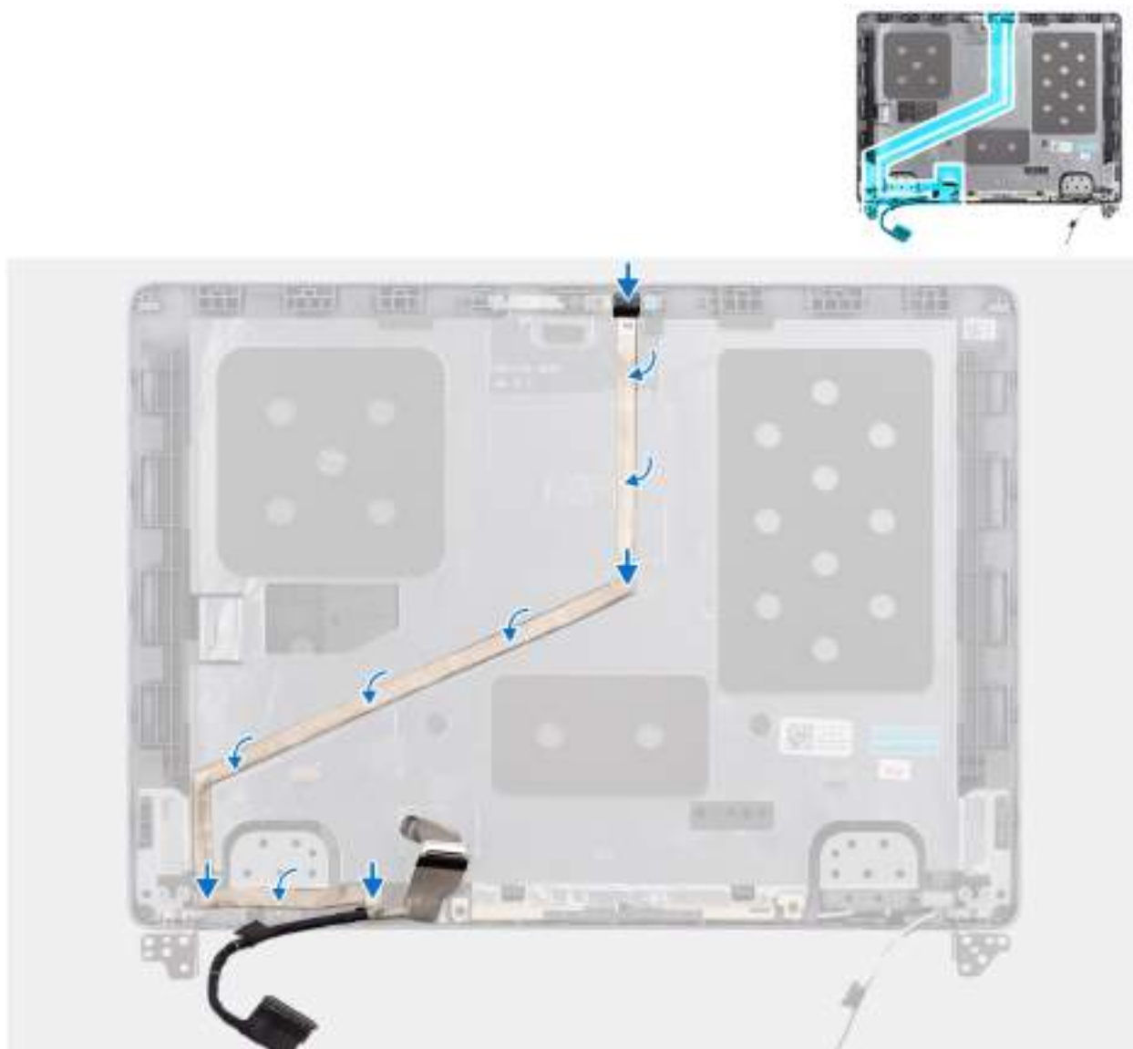
Obrázek 65. Vložení kabelu displeje
