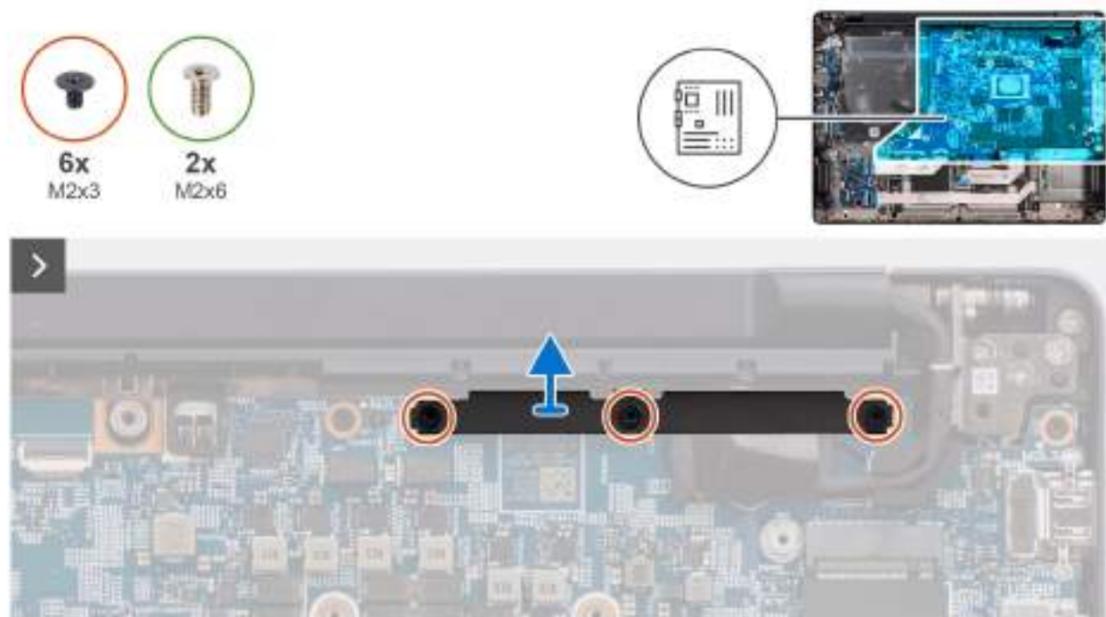
Obrázek 71. Demontáž základní desky
