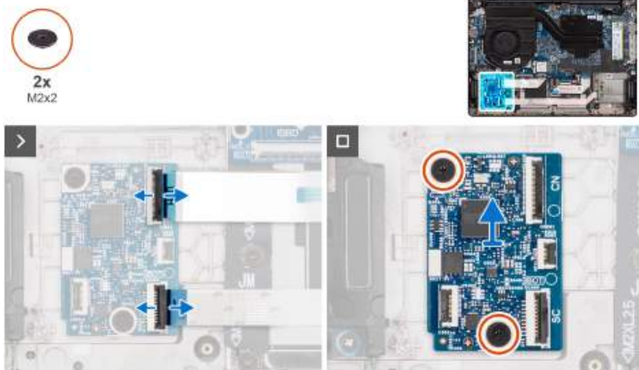
Obrázek 33. Demontáž desky USH
