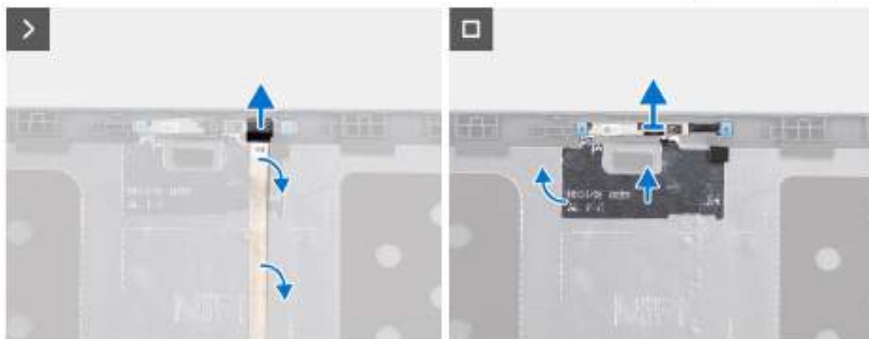
Obrázek 66. Demontáž kamery
