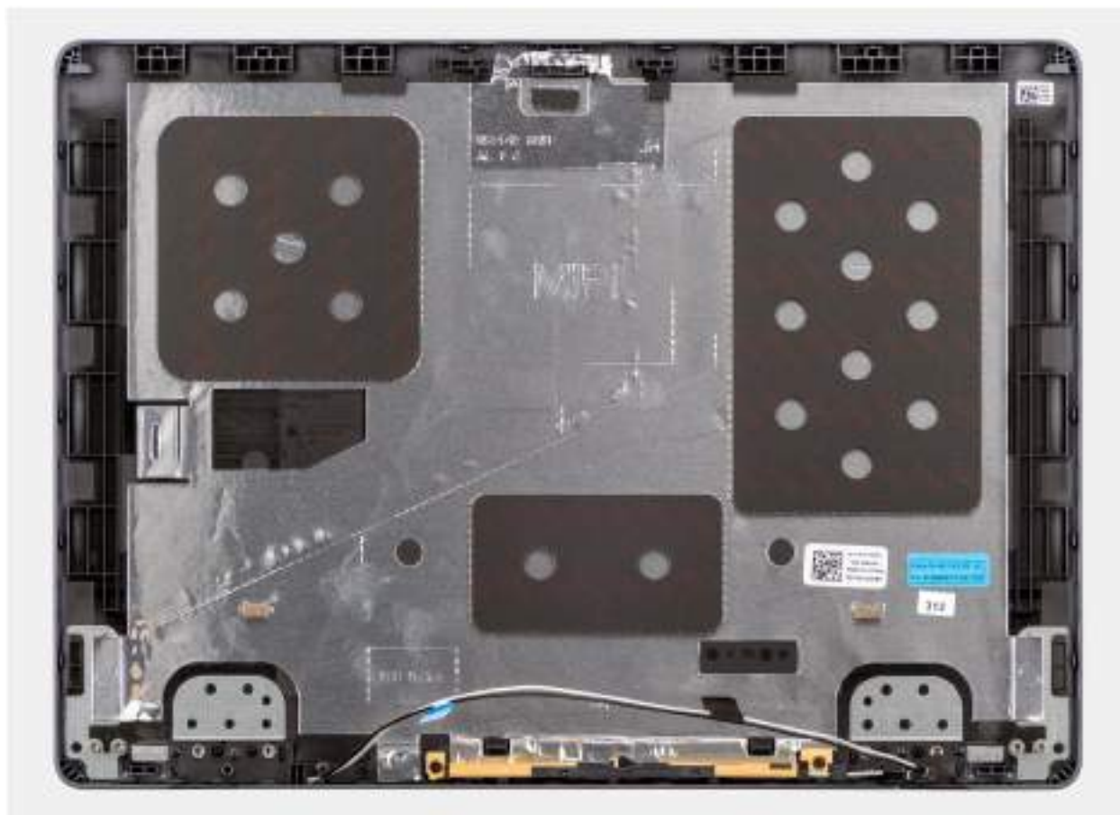
Obrázek 69. Zadní kryt displeje a sestava antény
