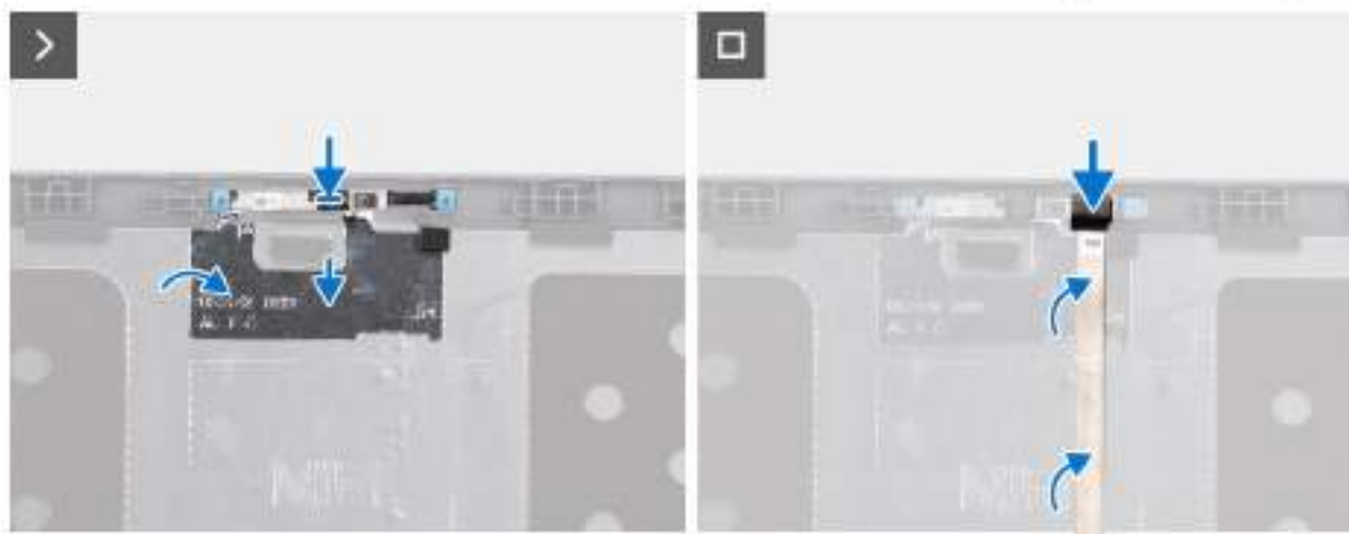
Obrázek 67. Montáž kamery
