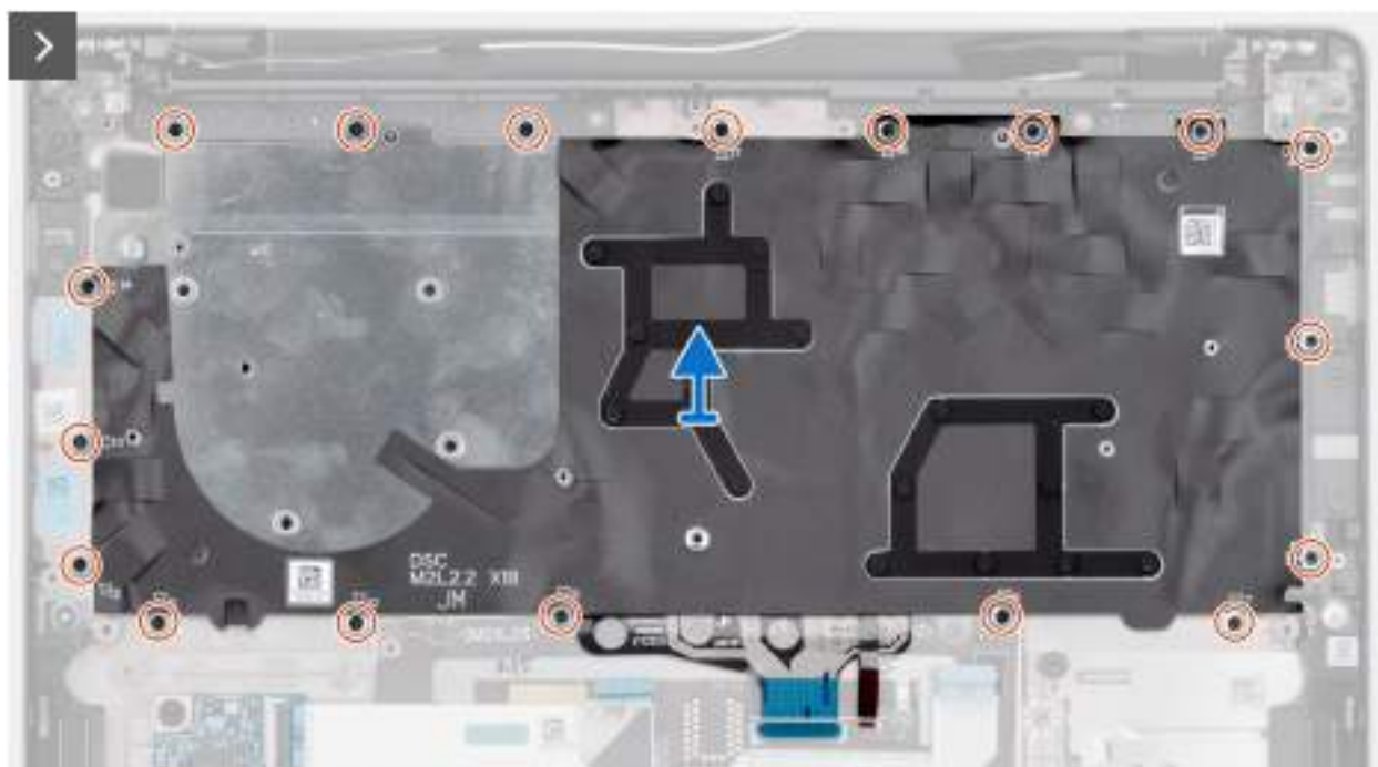
Obrázek 81. Demontáž klávesnice
