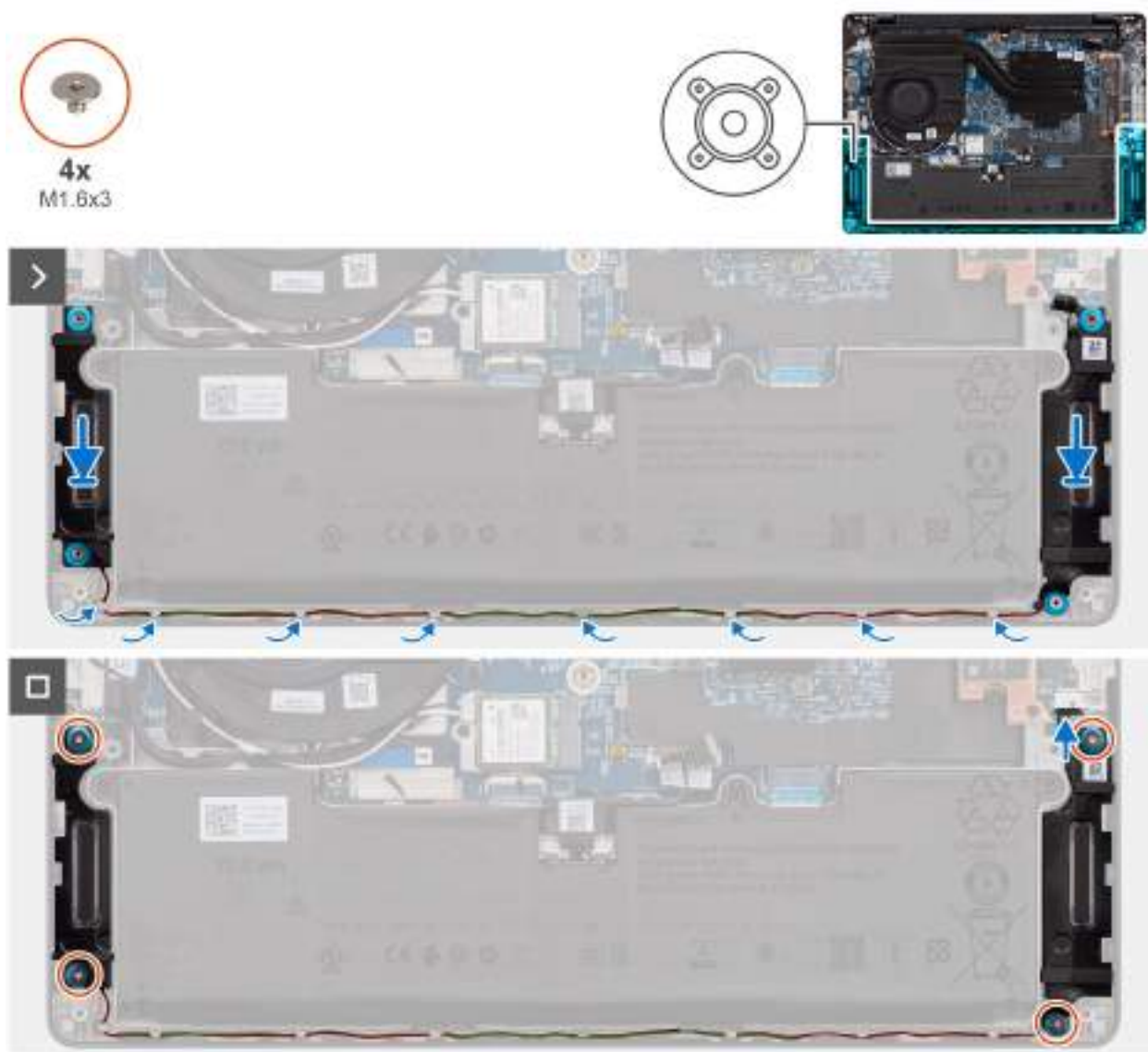
Obrázek 27. Montáž reproduktorů
