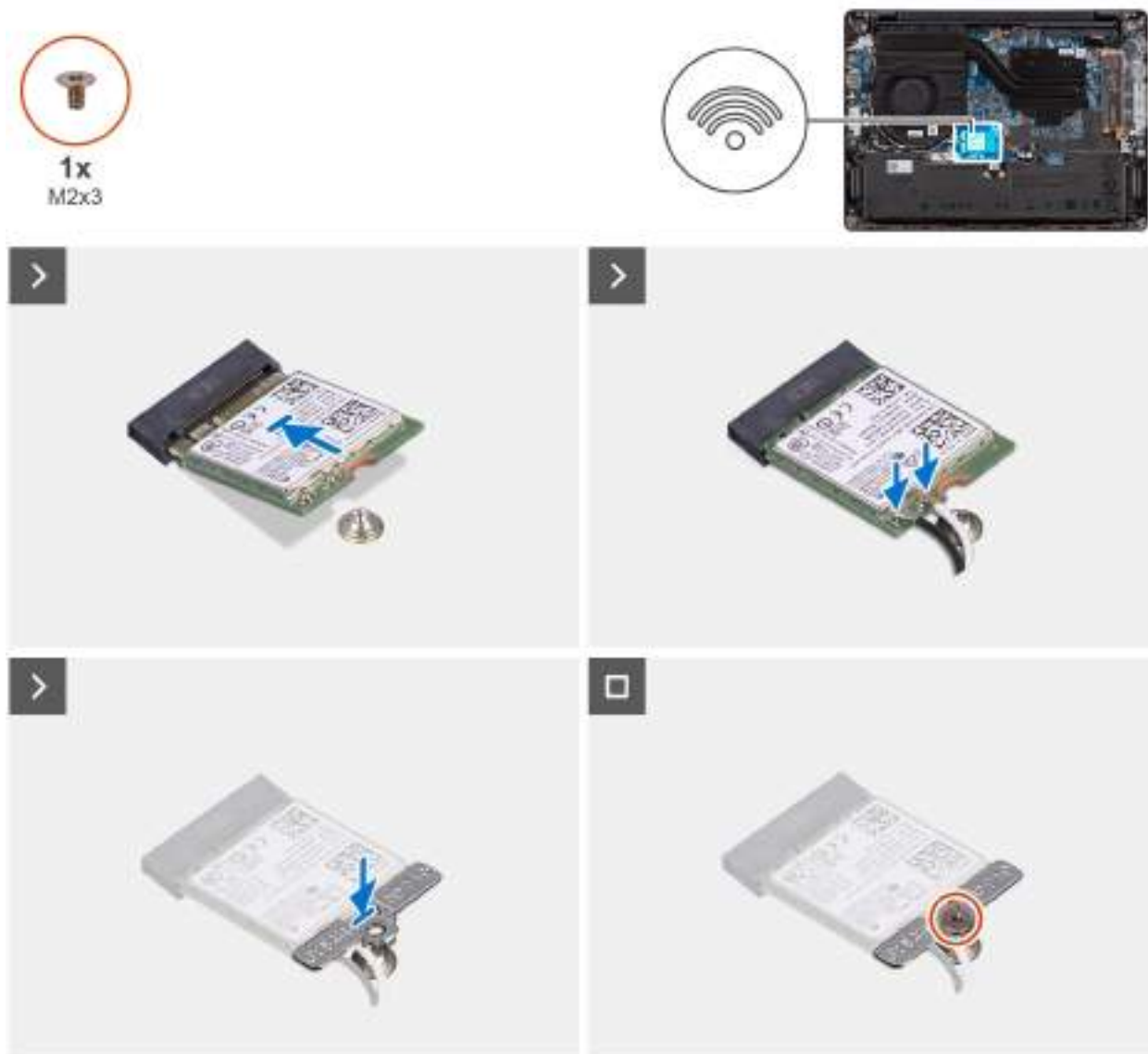
Obrázek 25. Montáž bezdrátové karty
