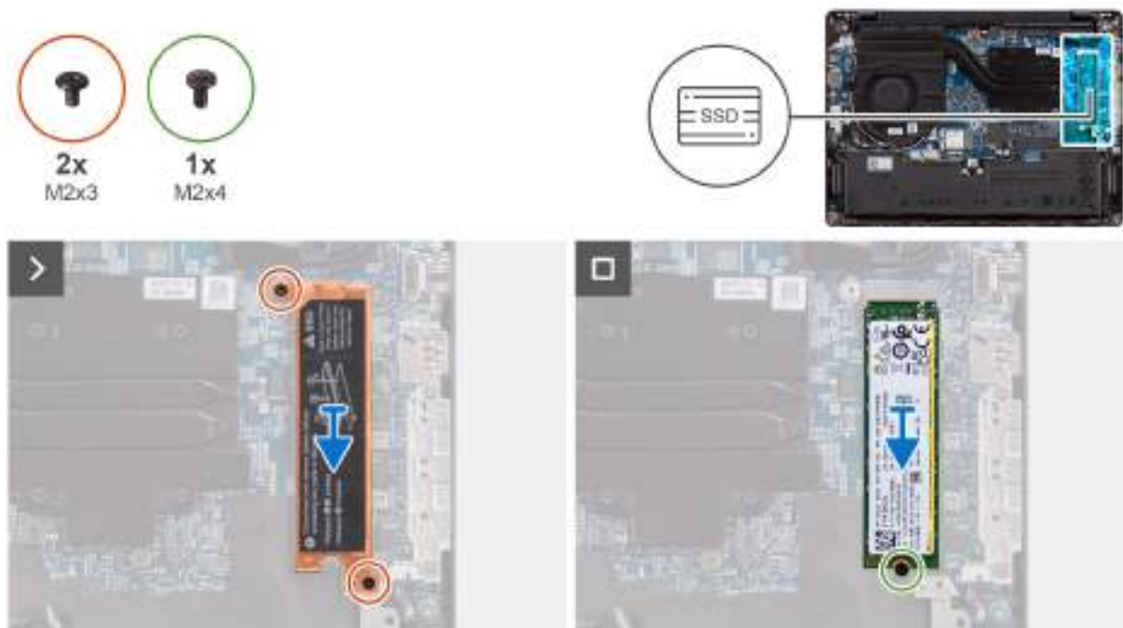
Obrázek 22. Demontáž disku SSD M.2 2280
