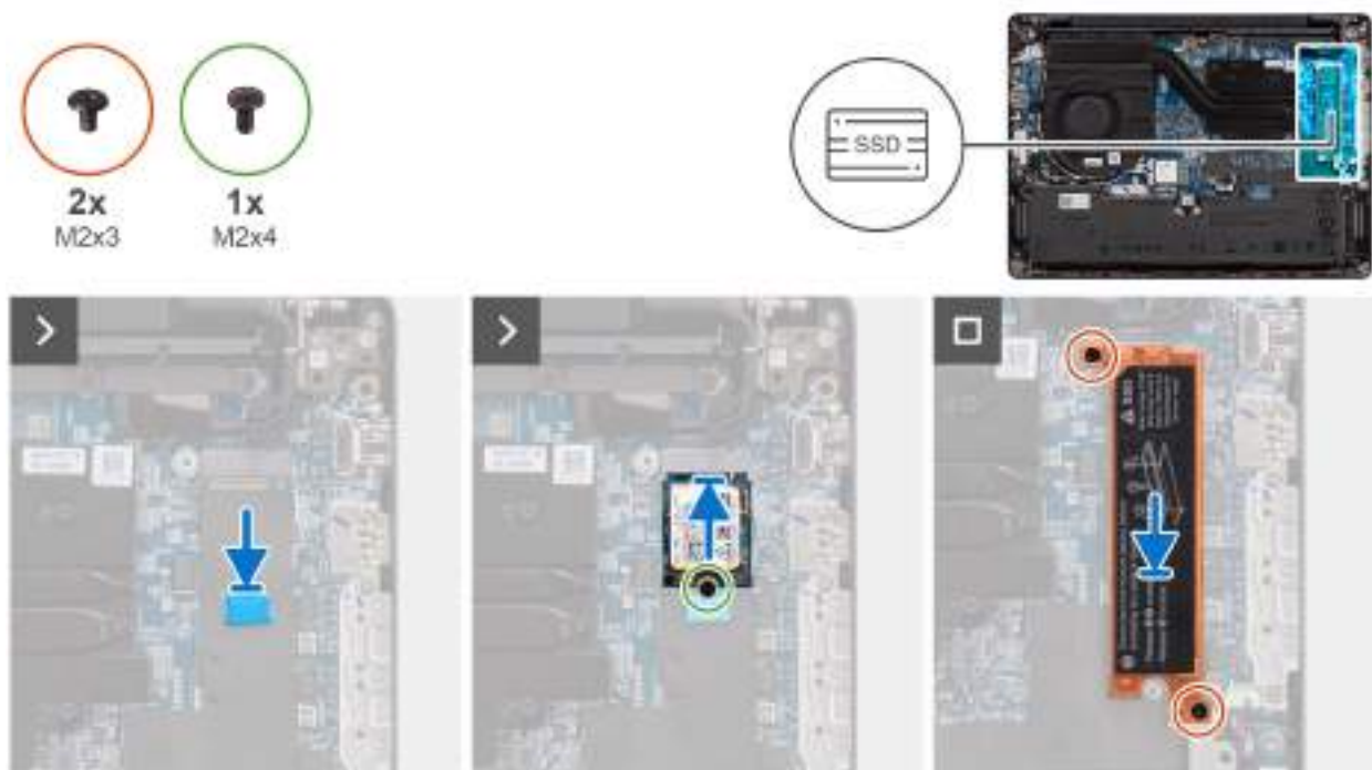
Obrázek 21. Instalace disku SSD M.2 2230
