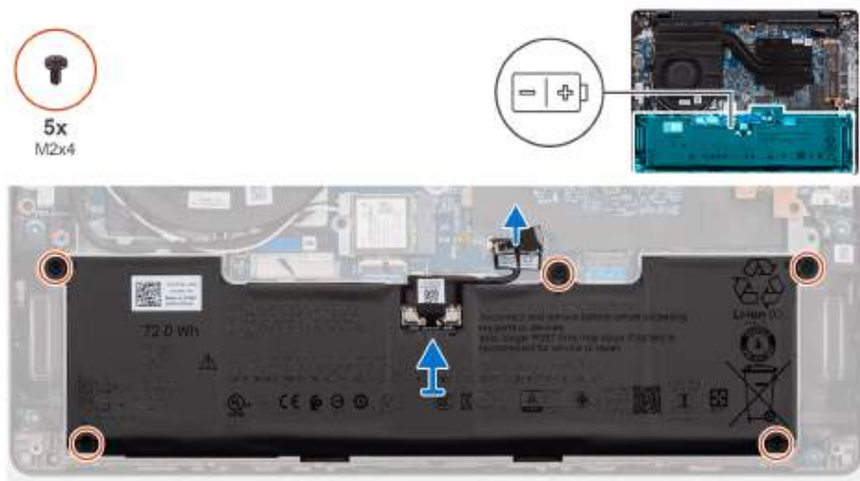
Obrázek 16. Vyjmutí baterie
