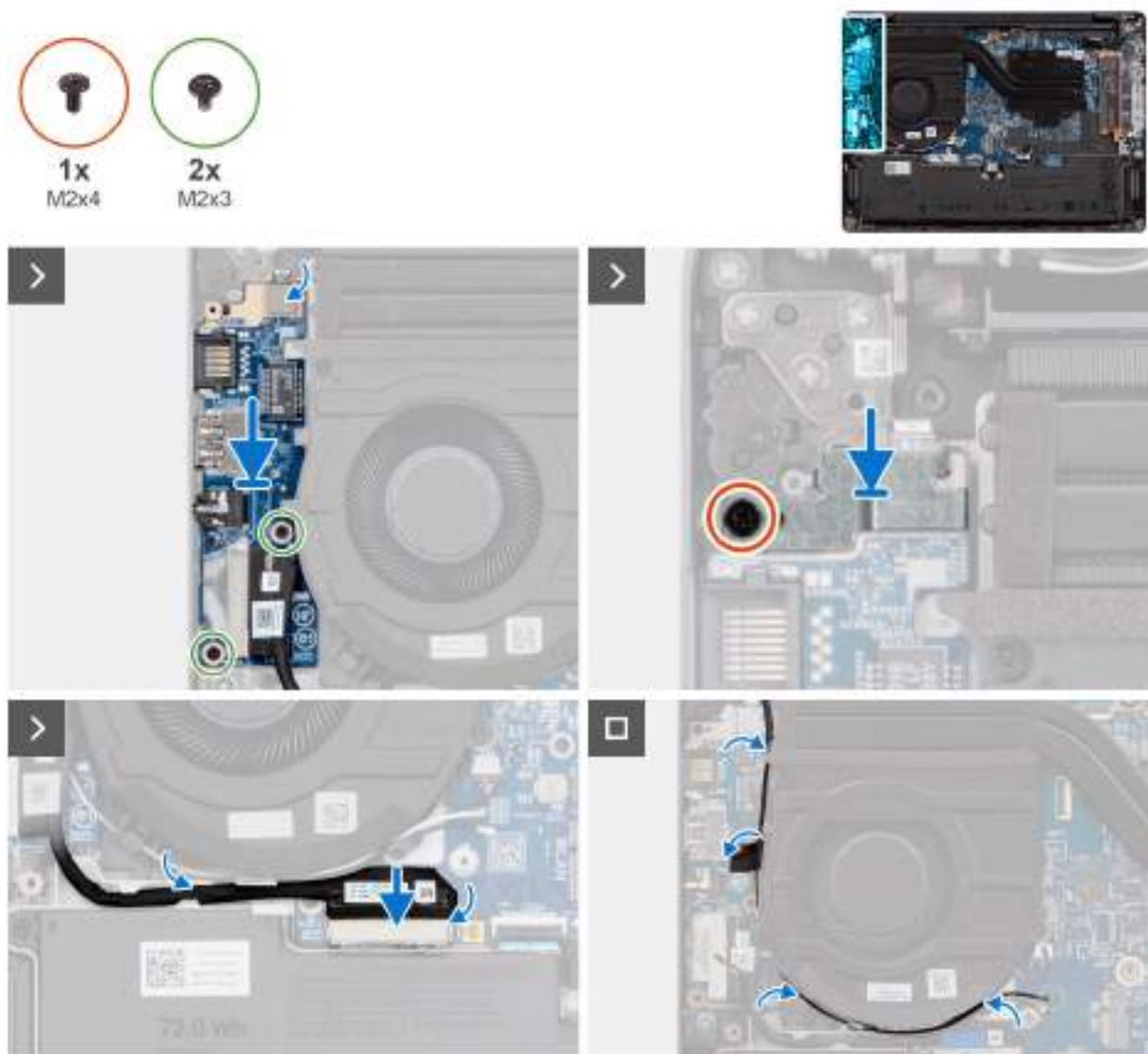
Obrázek 40. Vložení desky I/O
