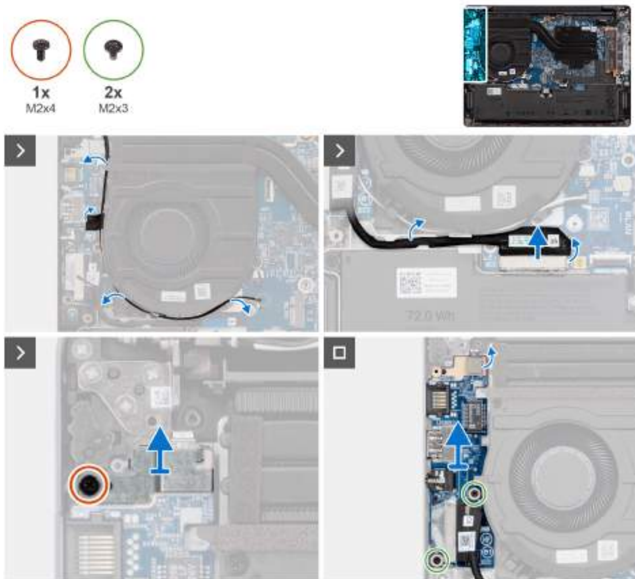
Obrázek 39. Demontáž desky I/O
