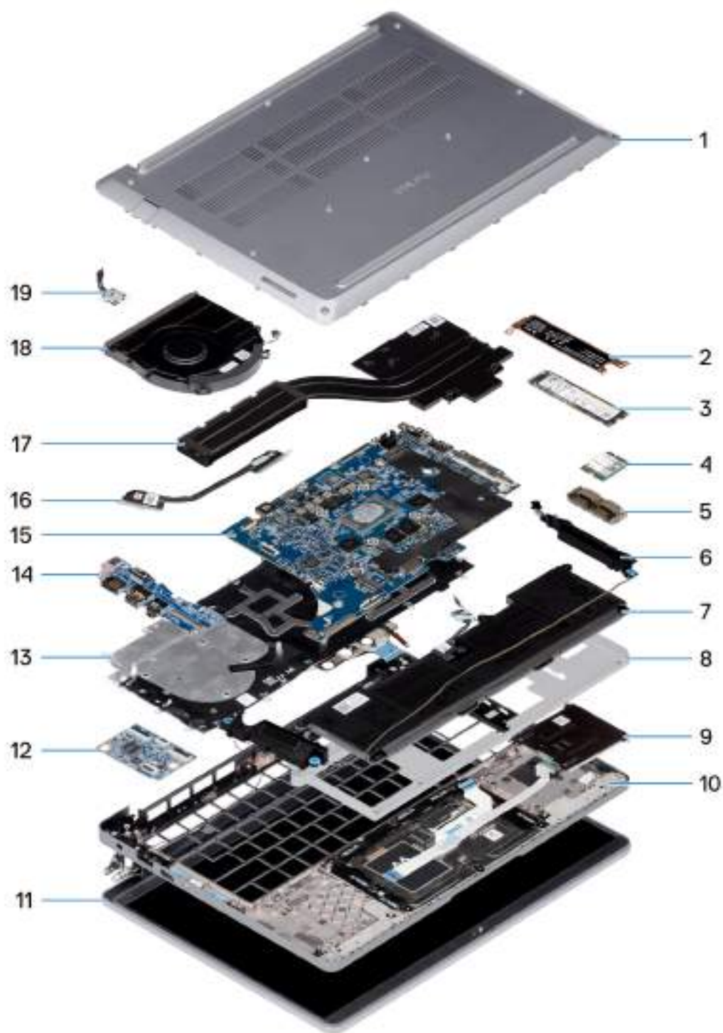
Obrázek 10. Hlavní komponenty Dell Pro Max 14 MC14255
