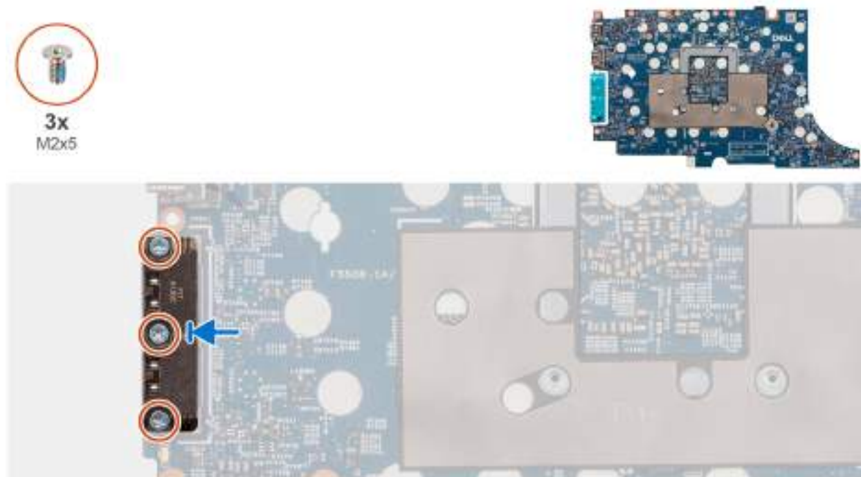
Obrázek 79. Montáž modulu USB Type-C
