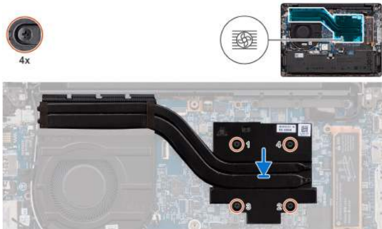
Obrázek 38. Montáž chladiče
