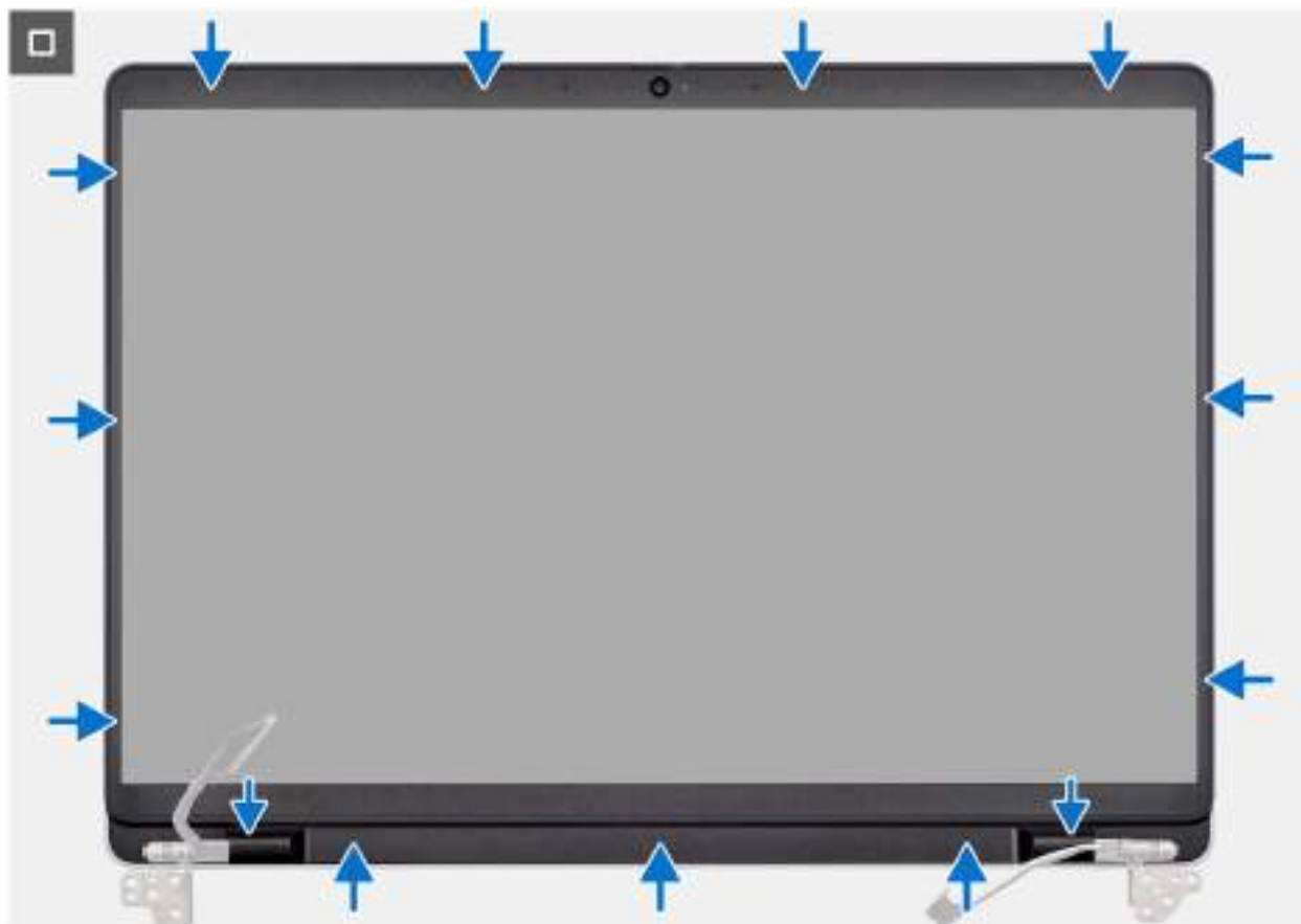
Obrázek 55. Montáž čelního krytu displeje
