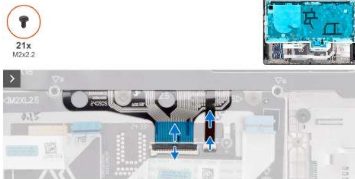
Obrázek 80. Demontáž klávesnice
