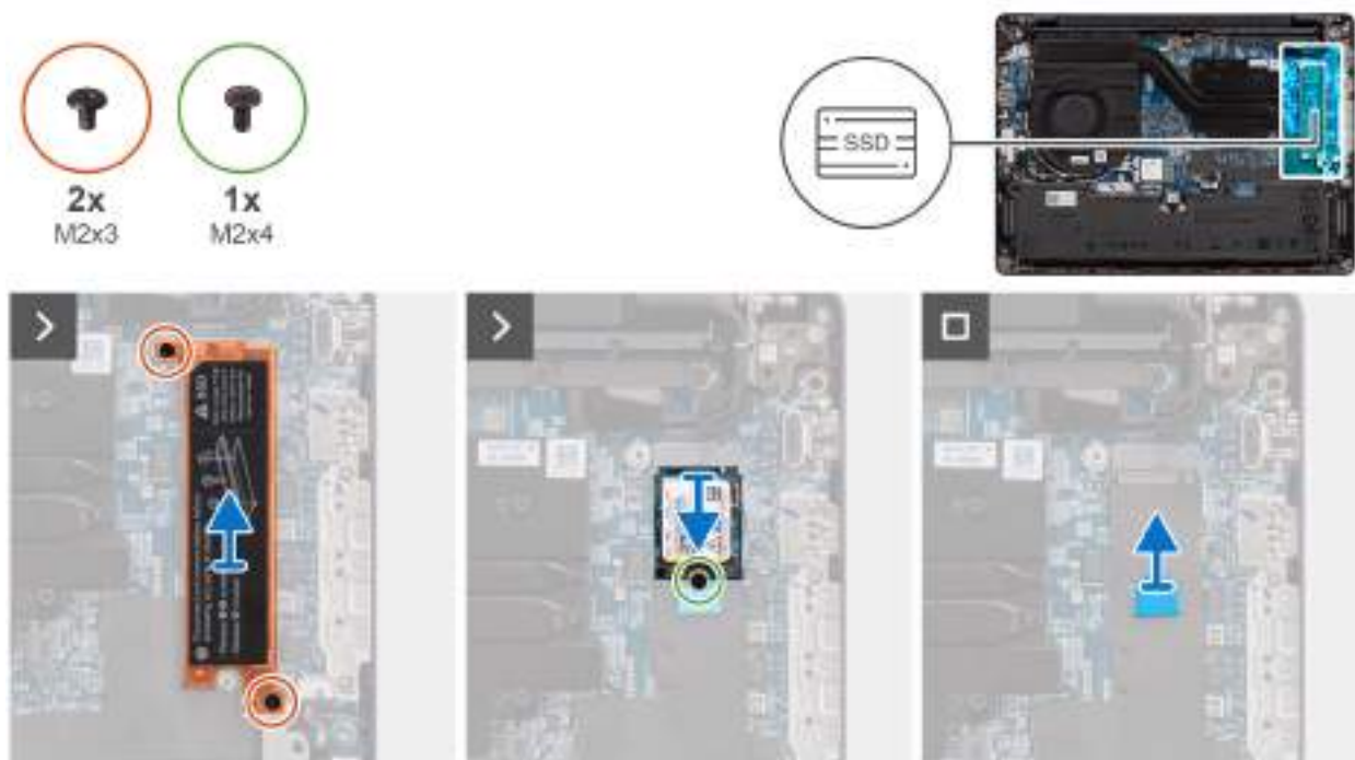
Obrázek 20. Demontáž disku SSD M.2 2230
