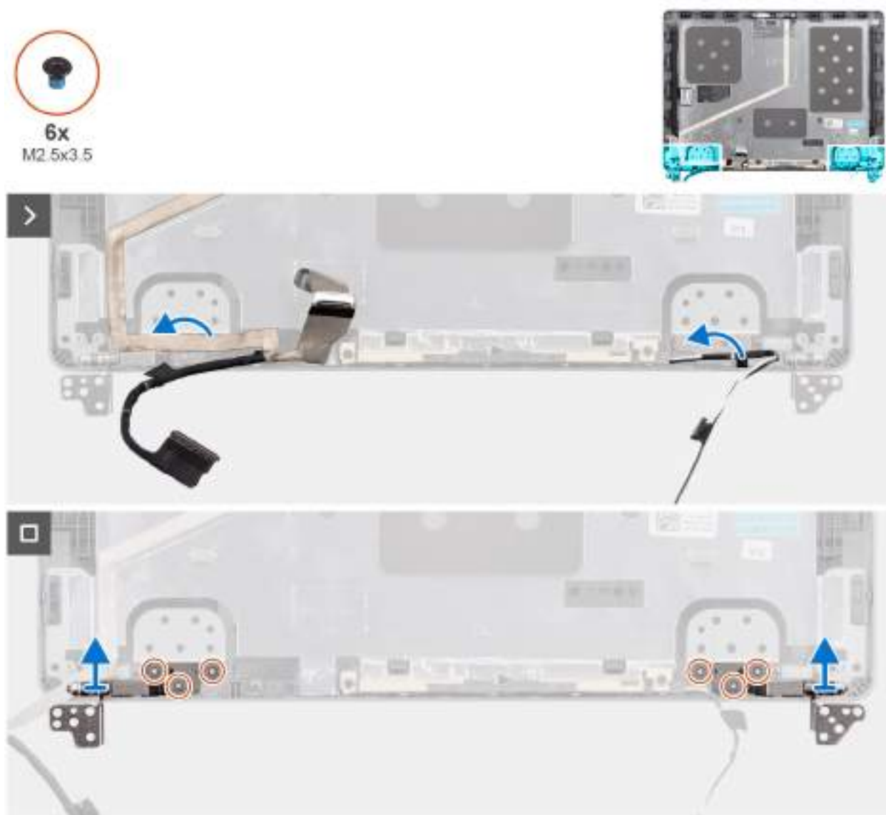
Obrázek 62. Demontáž pantů displeje
