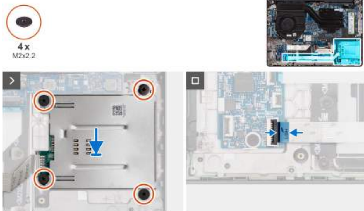
Obrázek 36. Montáž čtečky čipových karet
