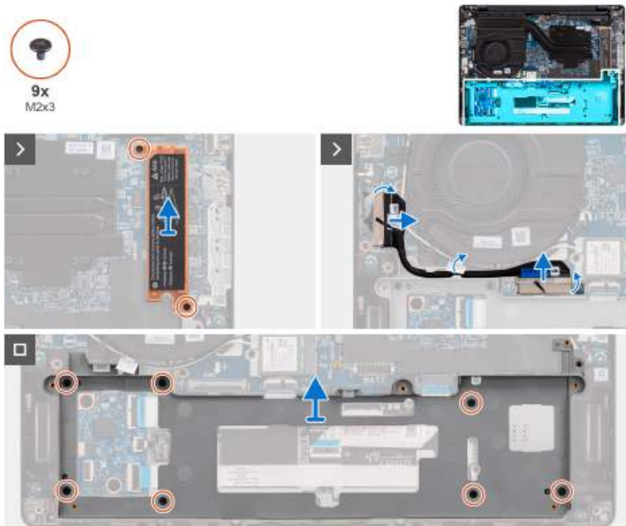
Obrázek 31. Demontáž rámu baterie
