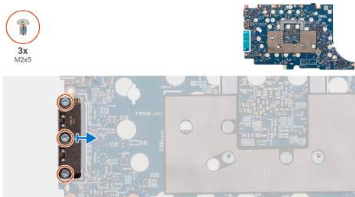
Obrázek 78. Demontáž modulu USB Type-C
