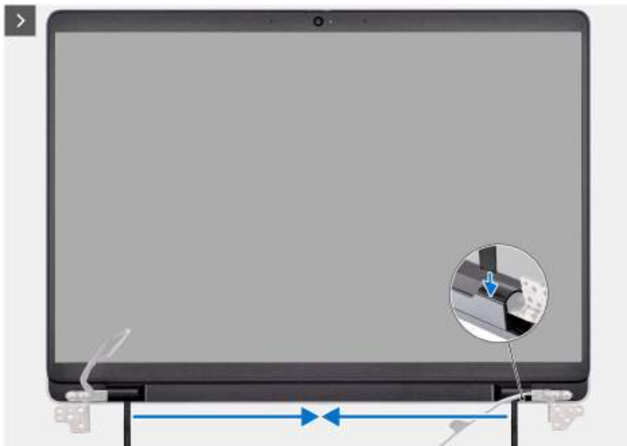
Obrázek 51. Demontáž čelního krytu displeje
