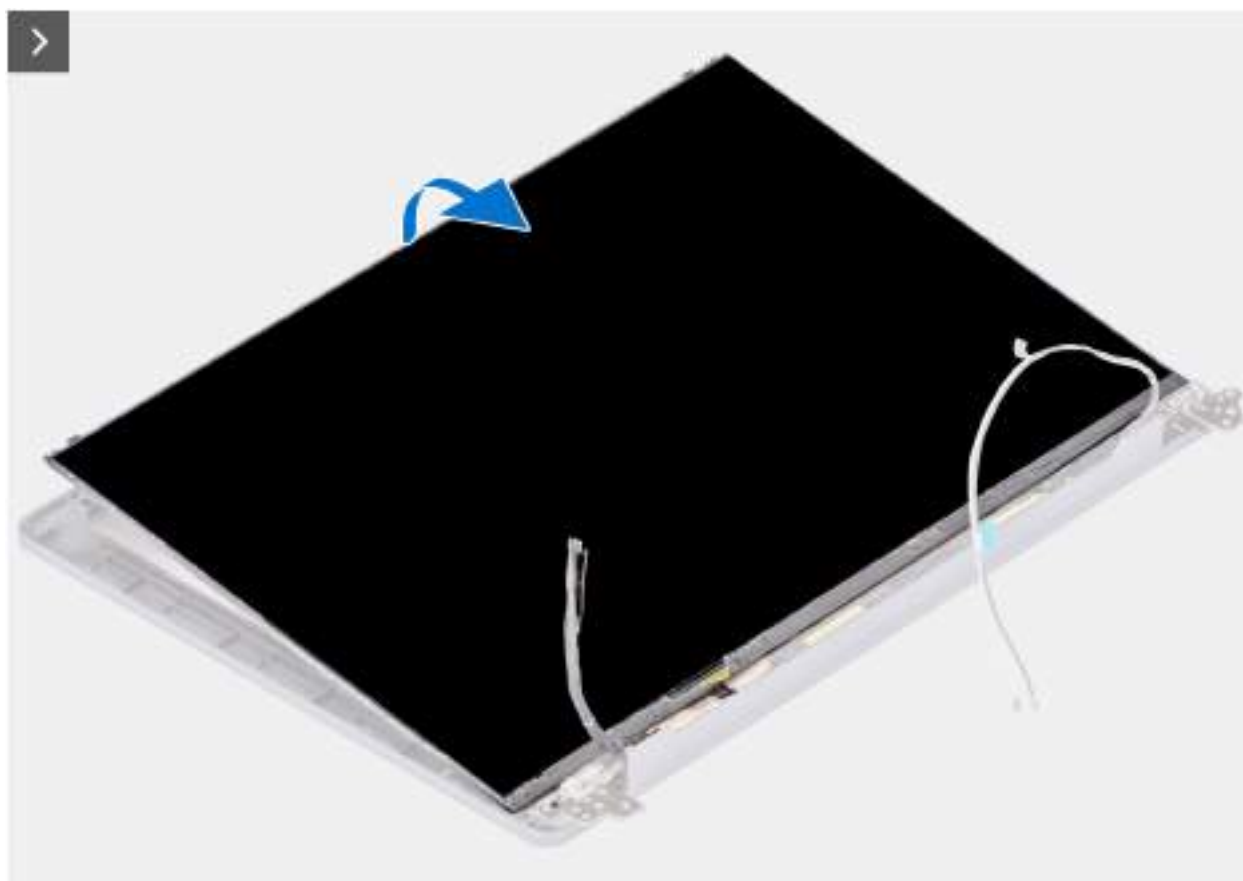
Obrázek 57. Demontáž obrazovky displeje
