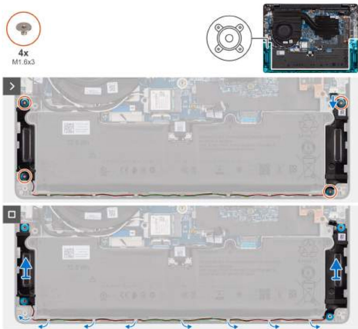
Obrázek 26. Demontáž reproduktorů
