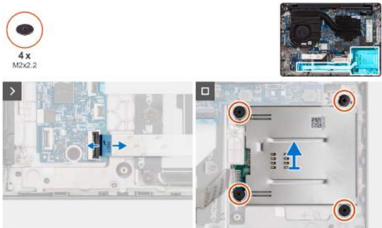
Obrázek 35. Demontáž čtečky čipových karet
