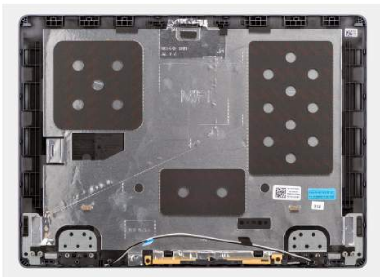
Obrázek 68. Zadní kryt displeje a sestava antény
