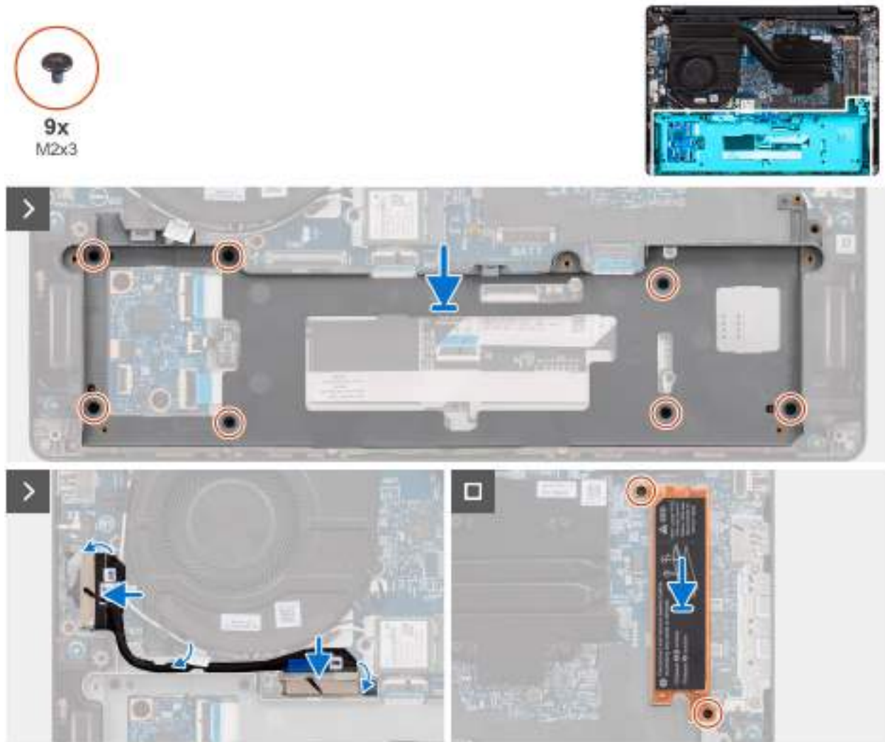
Obrázek 32. Montáž rámu baterie
