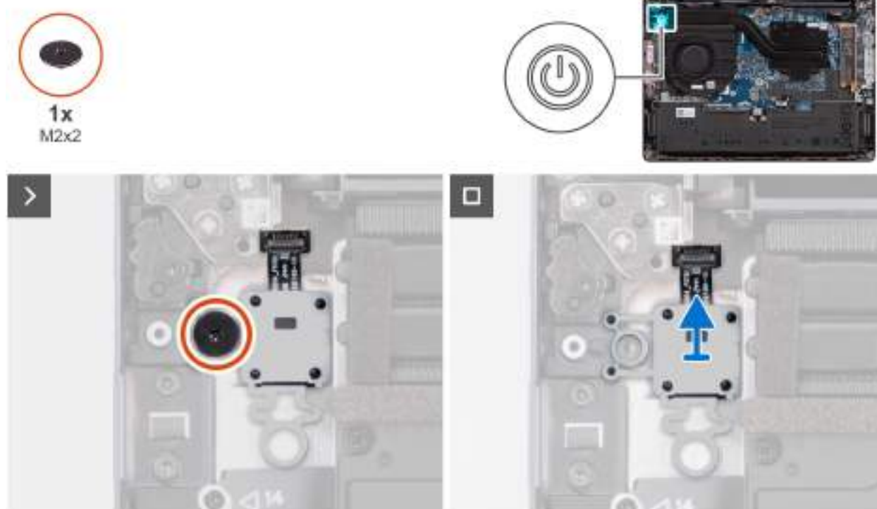
Obrázek 41. Demontáž vypínače
