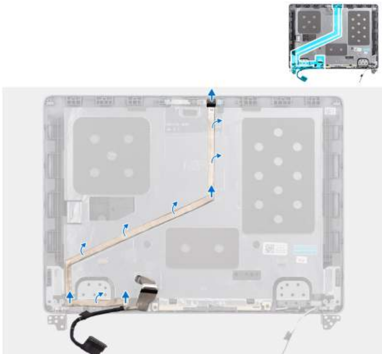
Obrázek 64. Vyjmutí kabelu displeje
