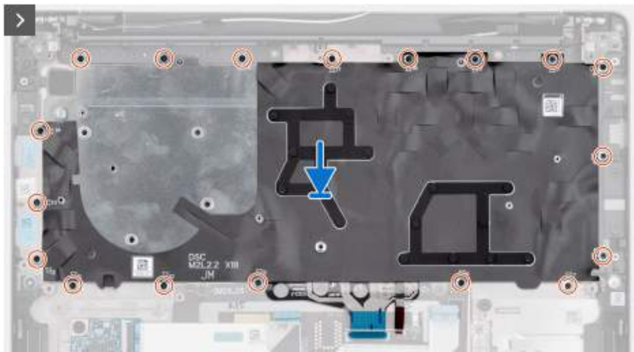
Obrázek 84. Montáž klávesnice
