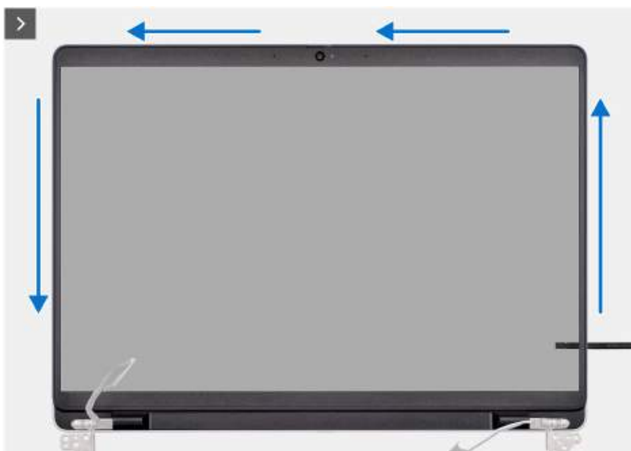
Obrázek 50. Demontáž čelního krytu displeje
