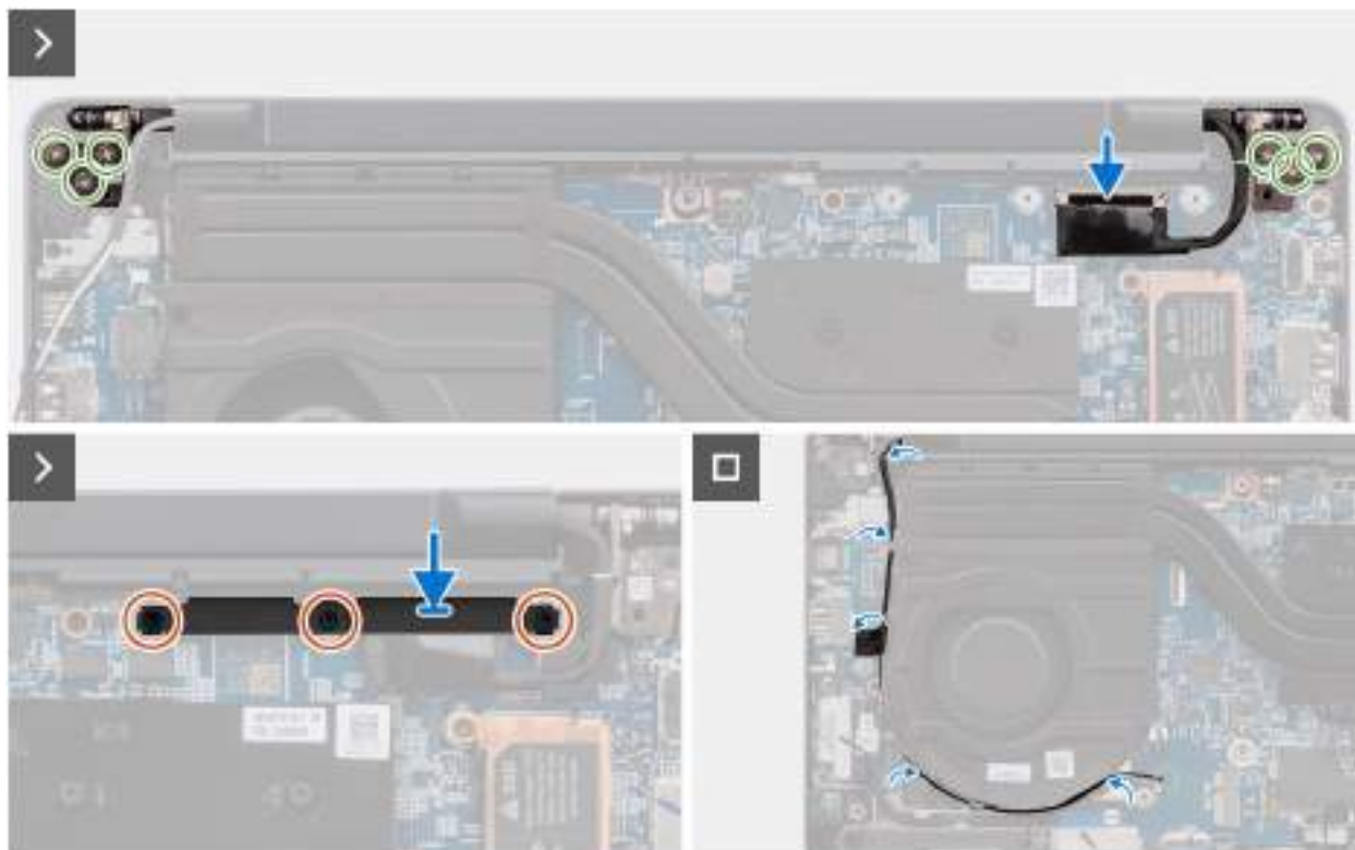
Obrázek 47. Montáž sestavy displeje
