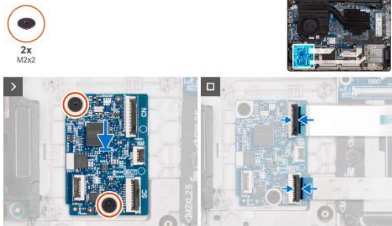
Obrázek 34. Montáž desky USH
