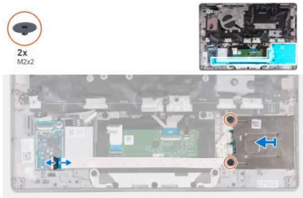
Obrázek 88. Demontáž čtečky čipových karet
