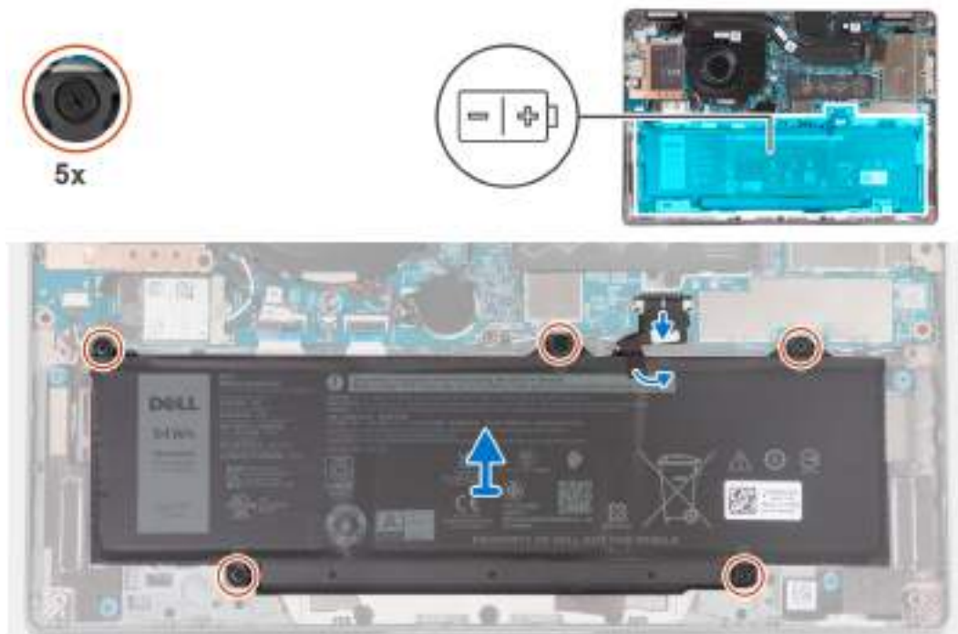
Obrázek 36. Vyjmutí baterie
