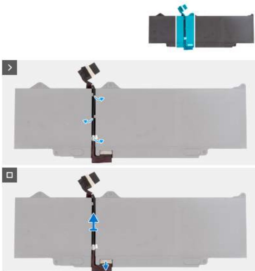
Obrázek 38. Demontáž kabelu baterie
