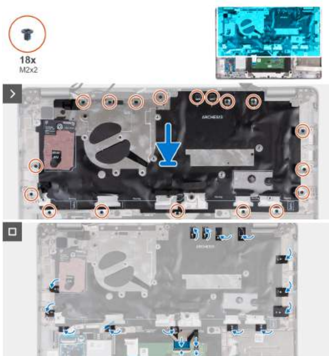
Obrázek 62. Montáž sestavy klávesnice
