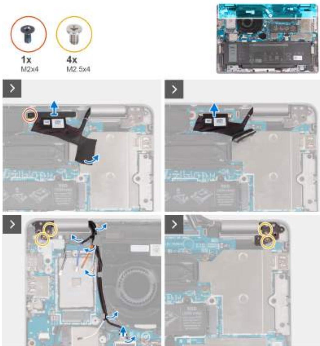
Obrázek 63. Demontáž sestavy displeje
