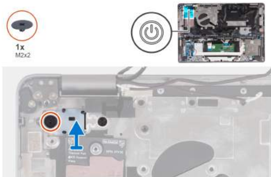
Obrázek 55. Demontáž vypínače
