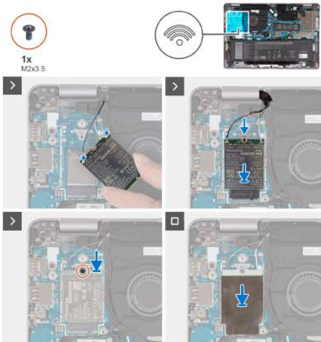
Obrázek 29. Namontujte kartu síť WWAN 4G.
