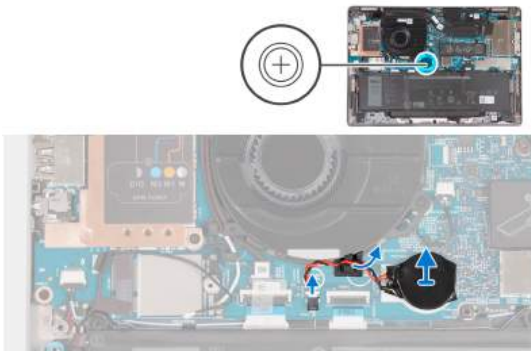
Obrázek 40. Vymutí knoflíkové baterie
