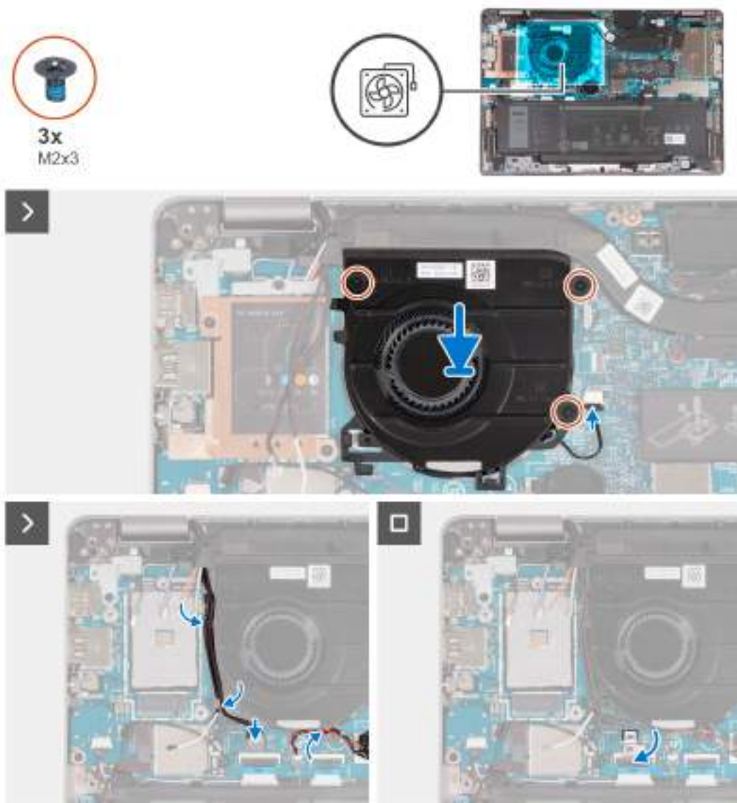
Obrázek 35. Nainstalujte ventilátor
