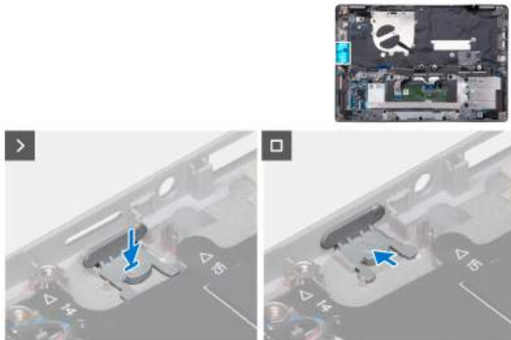
Obrázek 91. Montáž výplně slotu karty SIM
