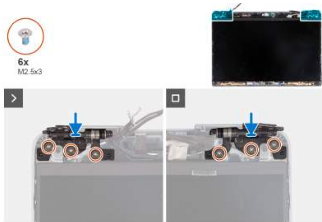
Obrázek 71. Demontáž pantů displeje (notebook)
