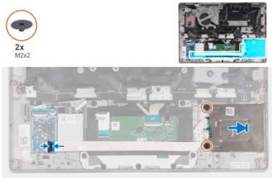
Obrázek 89. Montáž čtečky čipových karet
