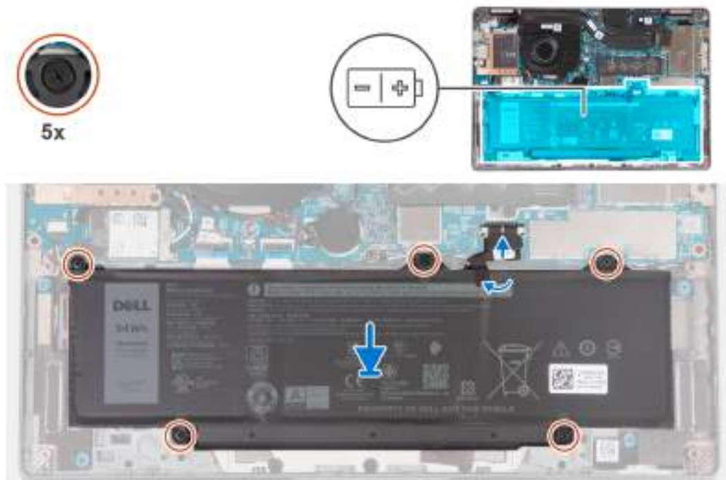
Obrázek 37. Vložení baterie
