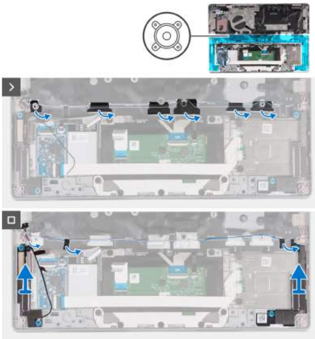
Obrázek 52. Demontáž reproduktorů
