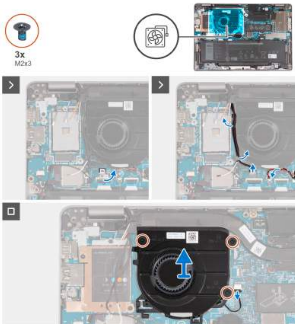
Obrázek 34. Demontujte ventilátor
