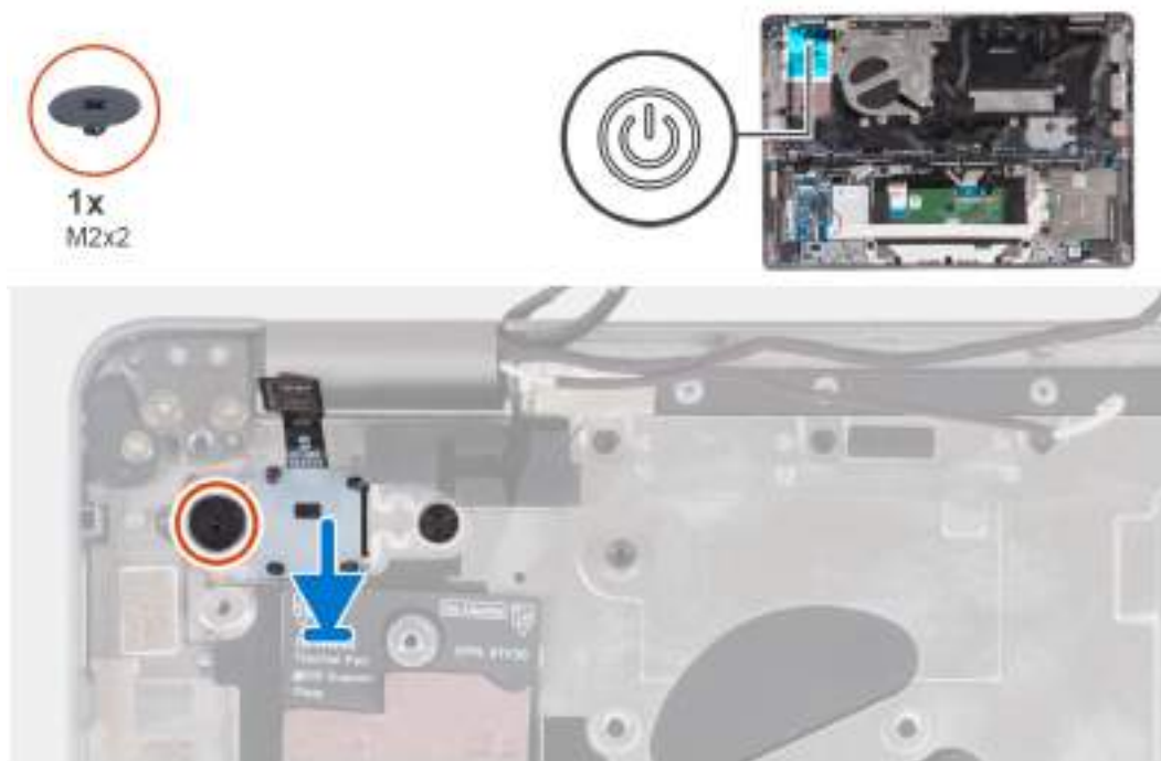
Obrázek 58. Montáž vypínače se čtečkou otisků prstů
