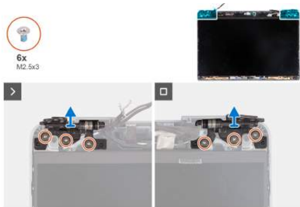
Obrázek 70. Demontáž pantů displeje (notebook)
