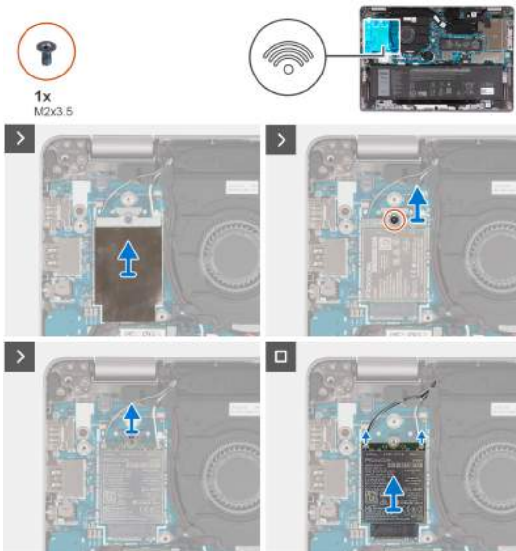
Obrázek 28. Vyjměte kartu WWAN 4G
