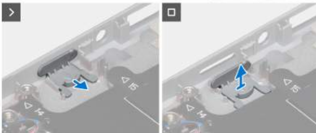
Obrázek 90. Demontáž výplně slotu karty SIM
