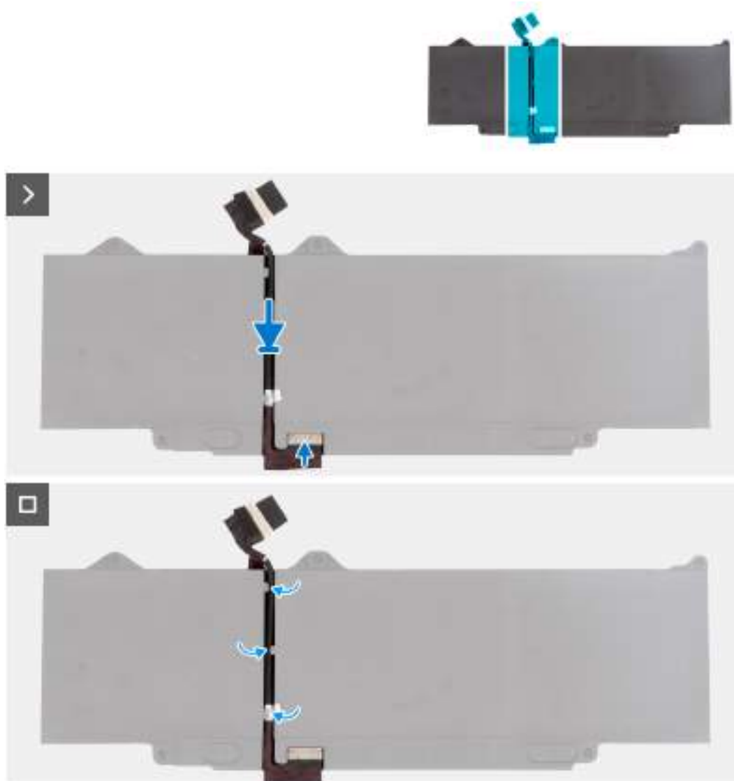
Obrázek 39. Montáž kabelu baterie
