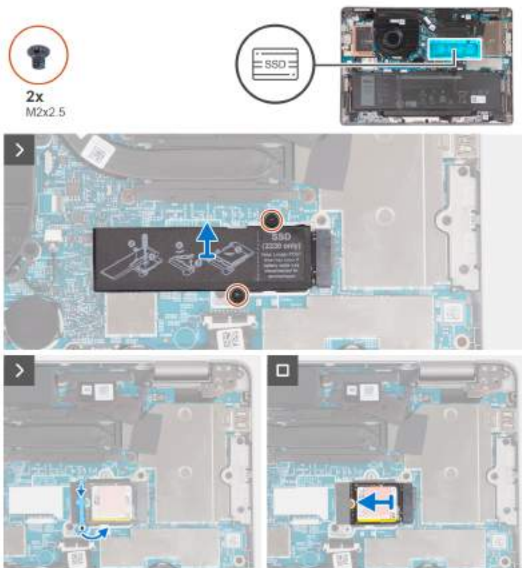
Obrázek 23. Vyjměte disk SSD M.2 2230.
