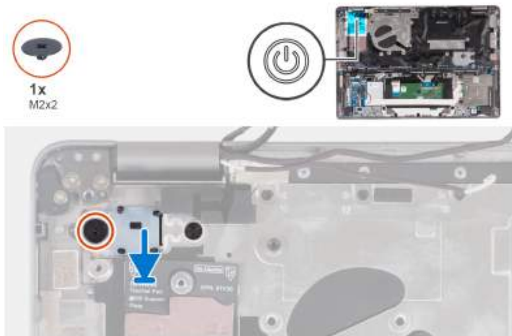
Obrázek 56. Montáž vypínače
