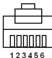
Konektor kabelu číslovaní pinů
